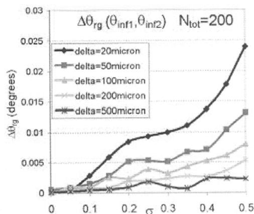
Figure 1.9 : Déviation de \theta_{rg} à partir de sa valeur à \sigma=0 en fonction de \sigma pour différentes valeurs du diamètre moyen \delta .
