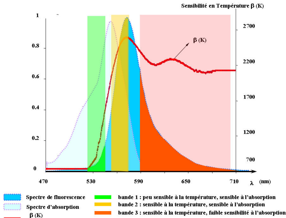
Figure 3.2 : Spectre absorption, d'émission de la rhodamine B excitée par la longueur d'onde \lambda=514,5 nm. Positions des 3 bandes spectrales de détection LIF et sensibilité en température de l'intensité de fluorescence.
