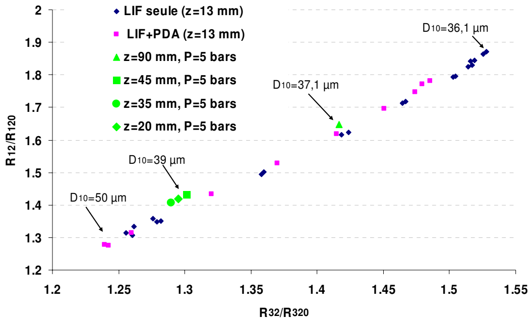
Figure 4.90 : Evolution du rapport de fluorescence normalisé R_{12} en fonction de R_{32} à z=13 mm, obtenue par modification de la pression d'injection. Mesures réalisées à d'autres distances axiales.
