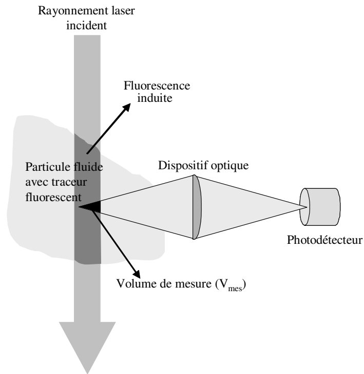
Figure 2.3 : Schéma typique d'une chaîne de fluorescence induite par laser.
