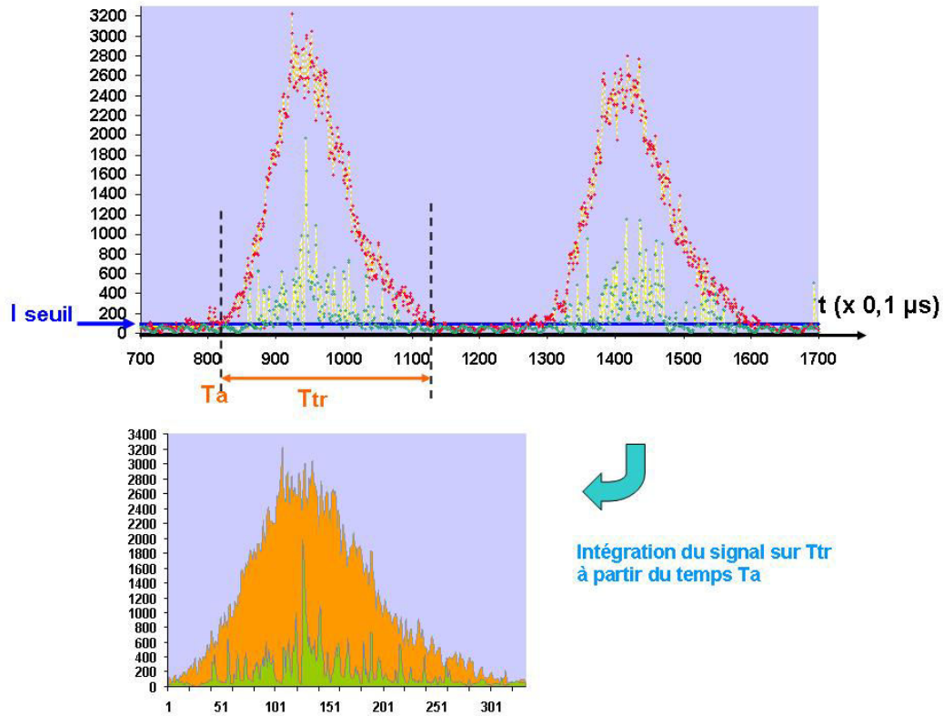
Figure 4.27 : exemple de seuillage sur la voie 2 et intégration du signal sur le passage d'une goutte
