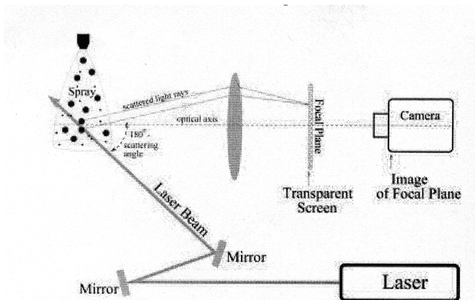
Figure 1.7 : Dispositif expérimental de réfractométrie d’arc-en-ciel global.
