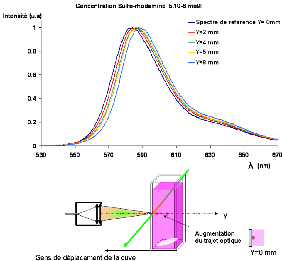
Figure 4.54 : Comparaison de spectres de fluorescence pour différents chemins optiques y . Influence de la réabsorption.
