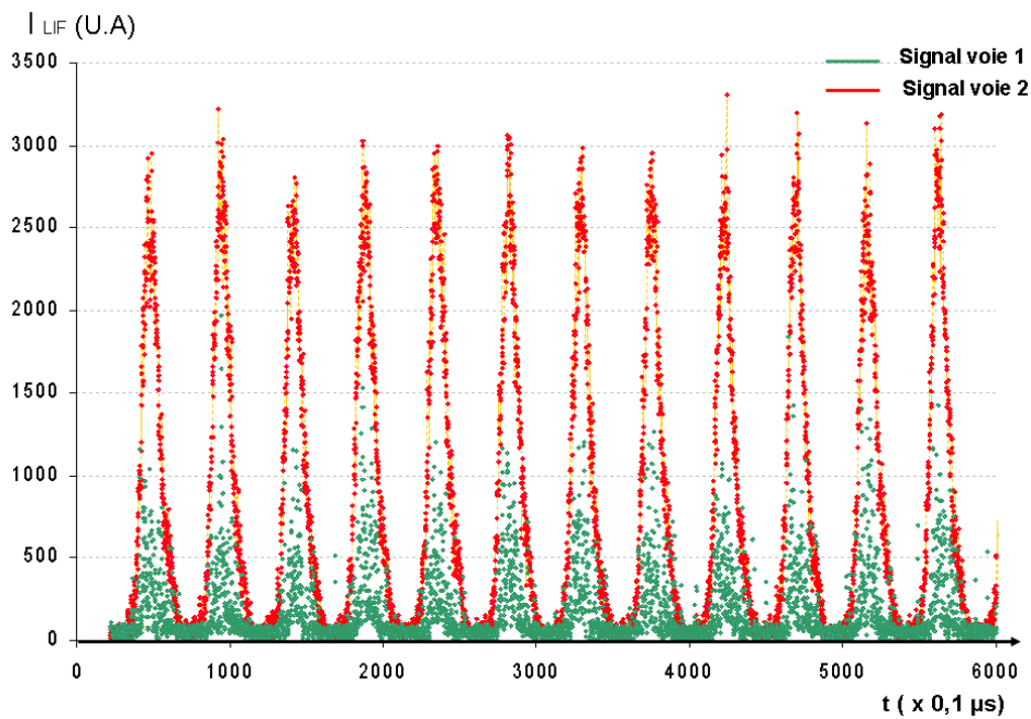
Figure 4.26: signaux de fluorescence issus de gouttelettes monodisperses (diamètre 116 \mu\text{m} ).
