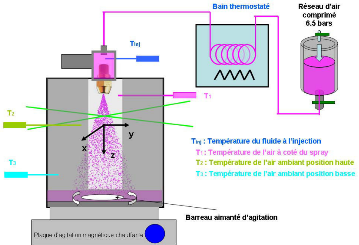
Figure 4.97: Dispositif expérimental d'injection du spray dans une cellule saturée.
