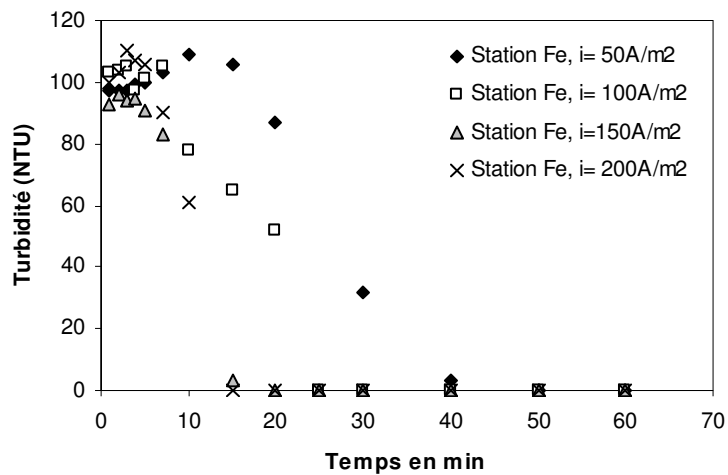
Figure III-41 : Evolution de la turbidité de l'effluent « station » au cours du traitement avec des électrodes de fer.
