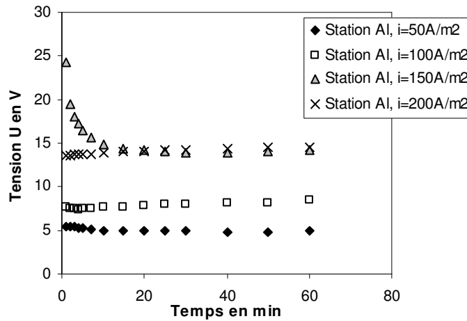
Figure III-8 : Evolution de la tension au cours du traitement de l'effluent station avec les électrodes d'aluminium
