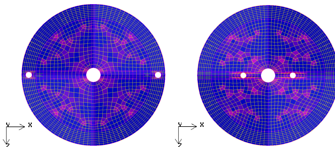
Figure III-7 : Faces optimisées dans le plan XZ (de gauche à droite) : face supérieure, face inférieure
