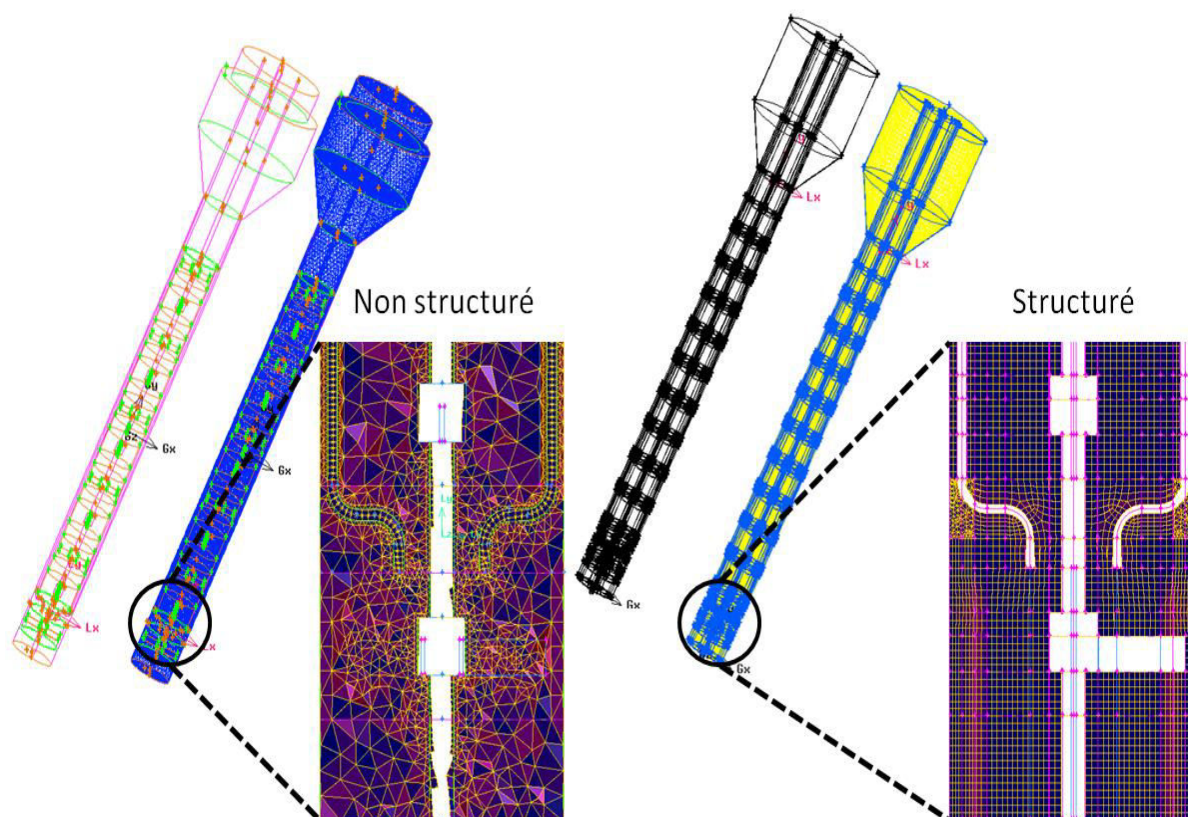
Figure III-5 : Maillages non structuré et structuré
