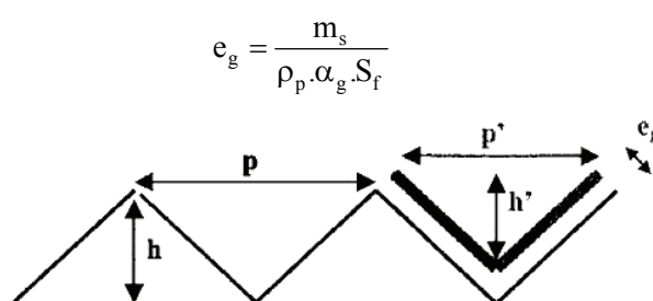
Figure 1-16: Réduction de la surface de filtration engendrée par le dépôt de particules sur le medium filtrant, le long de la hauteur d'un pli (Del Fabbro, 2001)
