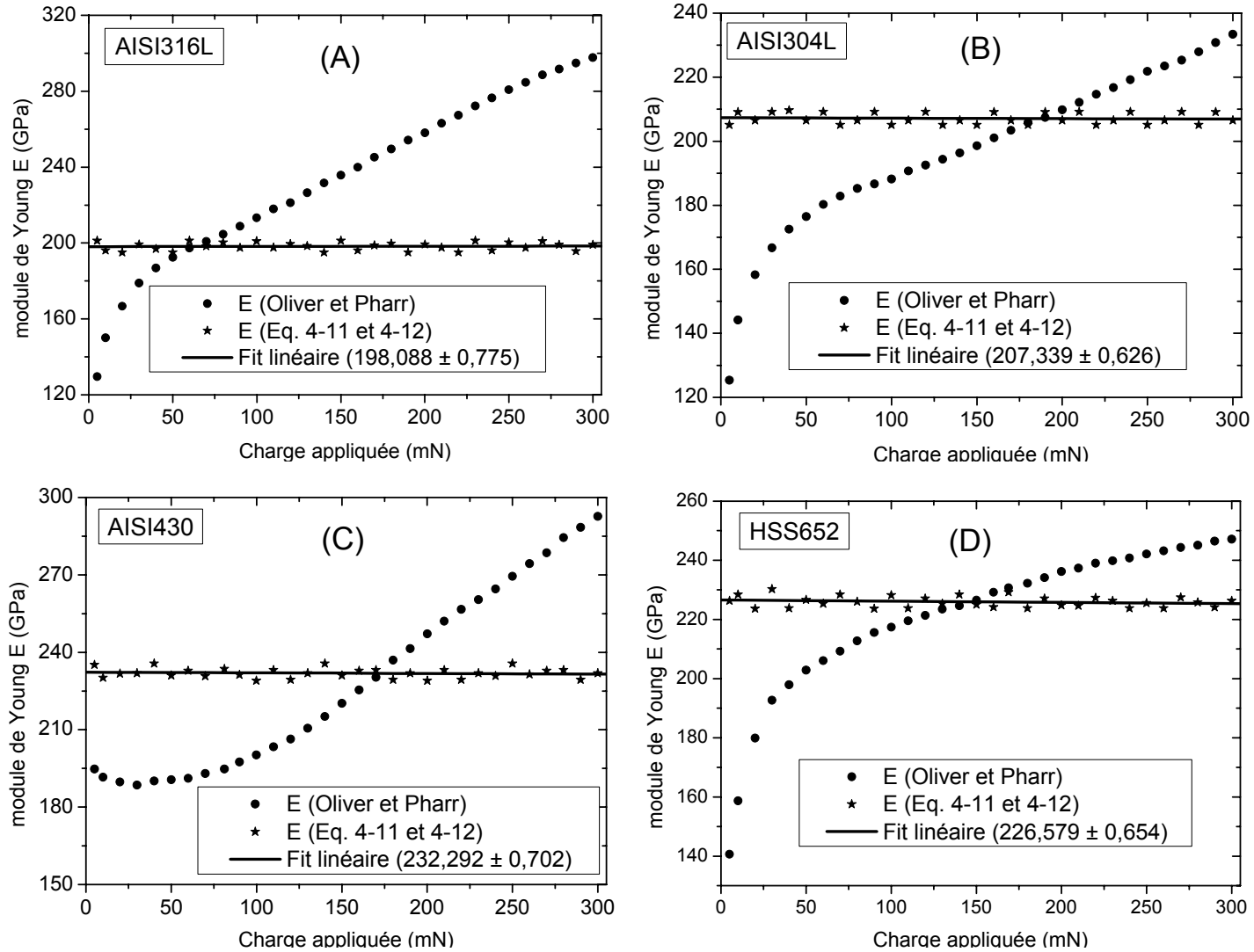
Figure 4-19 : Comparaison entre les résultats obtenus avec la méthode de Oliver et Pharr et celle basée sur les équations 4-11 et 4-12.
