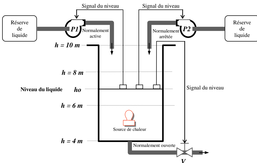
Figure 3.18 – Réservoir et sa régulation de niveau.
