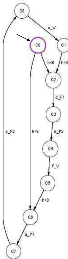
(e) Automate de la commande
