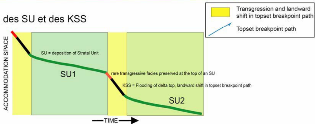
Figure 5.25 : a) Graphique simplifié représentant l'évolution qualitative de l'espace d'accommodation (A) pendant deux cycles de variations du niveau marin de 100 ka. Les variations eustatiques sont superposées au déplacement sur une faille normale. La somme de ces deux courbes donne la courbe verte représentant l'accommodation cumulée avec le temps. L'augmentation et la baisse du débit de la rivière, ainsi que de l'apport sédimentaire, contrôlés respectivement par les périodes glaciaires et interglaciaires, sont indiquées. b) Succession simplifiée de deux Unités Stratigraphiques (SU) et de leurs Surfaces Stratigraphiques clés (KSS) se déposant pendant les cycles représentés en a. c) Position des SU et des KSS montrées en (b) sur la courbe de l'accommodation. En encart : symboles utilisés en (b), (modifié d'après Backert et al. , 2009).
