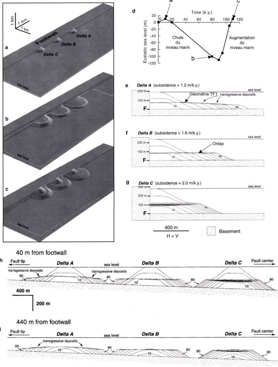
Figure 5.31 : Modélisation 3D de la formation des «fan-deltas» (modifié d'après Hardy & Gawthorpe, 1998) à S constant ( 960 \text{ m}^3/\text{ka} ), variations eustatiques asymétriques (période de 100 ka et amplitude de 120 m, Fig. d) et taux de subsidence qui varie parallèlement à la faille bordière, de l'extrémité vers le centre, de 0 à 3 m/ka. Le delta A correspond à un taux de subsidence de 1,2 m/ka, le delta B à un taux de 1,6 m/ka et le delta C à un taux de 2 m/ka. a) Etat du modèle après 10 ka et après une première augmentation du niveau marin. b) Etat du modèle après 80 ka, correspondant à la fin d'une période de chute maximum du niveau de la mer. c) Etat à la fin de la modélisation (110 ka). d) Allure de la courbe de variations du niveau marin et positions des figures a), b) et c). e), f), g) Coupes orthogonales à la direction de la faille bordière à travers les deltas A, B et C à la fin de la modélisation. Dans le cas de la figure e), des géométries de type TF1 (Fig. 5.2) sont identifiées. h), i) Coupes réalisées dans les trois deltas, parallèlement à la direction de la faille, à la fin de la modélisation, respectivement à 40 m et à 440 m du plan de faille.
