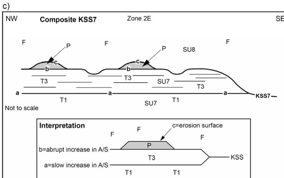
Figure 5.12 : Analyse du caractère composite des KSS3, KSS6 et KSS7. a) Coupe simplifiée orientée NO-SE/SO-NE de KSS3 (Figs 5.8 et 5.10). La surface «a» et la surface «b» sont définies sur ce schéma de corrélation. Un déplacement majeur en position proximale de plus de 1 km du TBP est enregistré par la surface «b».
