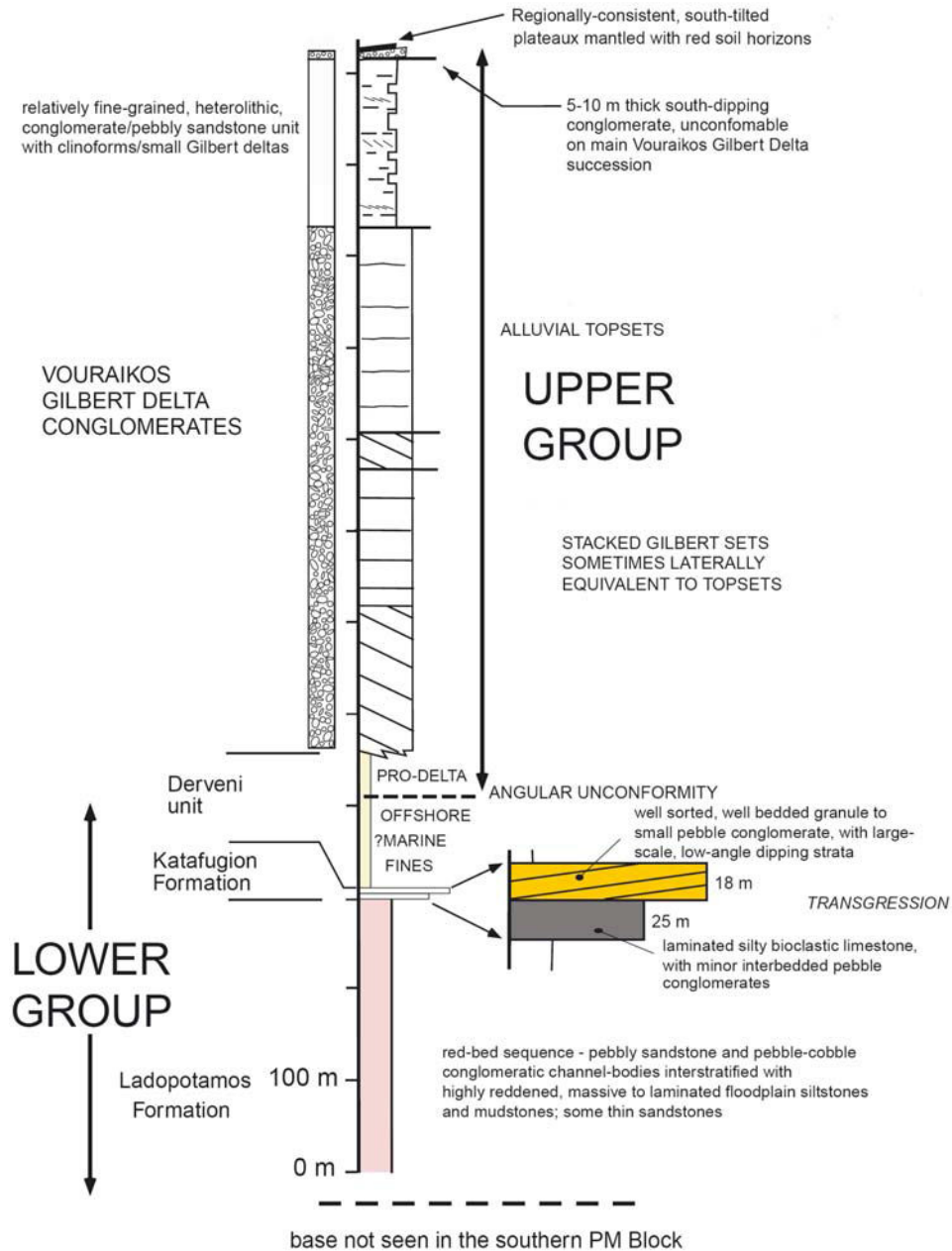
Figure 2.31 : Colonne stratigraphique synthétique modifiée d'après Ford et al. (2007b), représentant l'organisation des dépôts synrifts sur le bloc Pirgaki-Mamoussia (PM, Fig. 1.8 pour une localisation).
