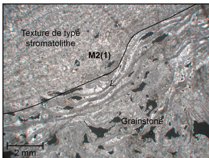
Figure 4.17 : Encroûtement algair ( L = Lithophyllum ) à lamines micritiques concentriques autour d'un nucléus de grainstone à bioclastes d'algues rouges (lame mince C32b, Fig. 4.12.b).
