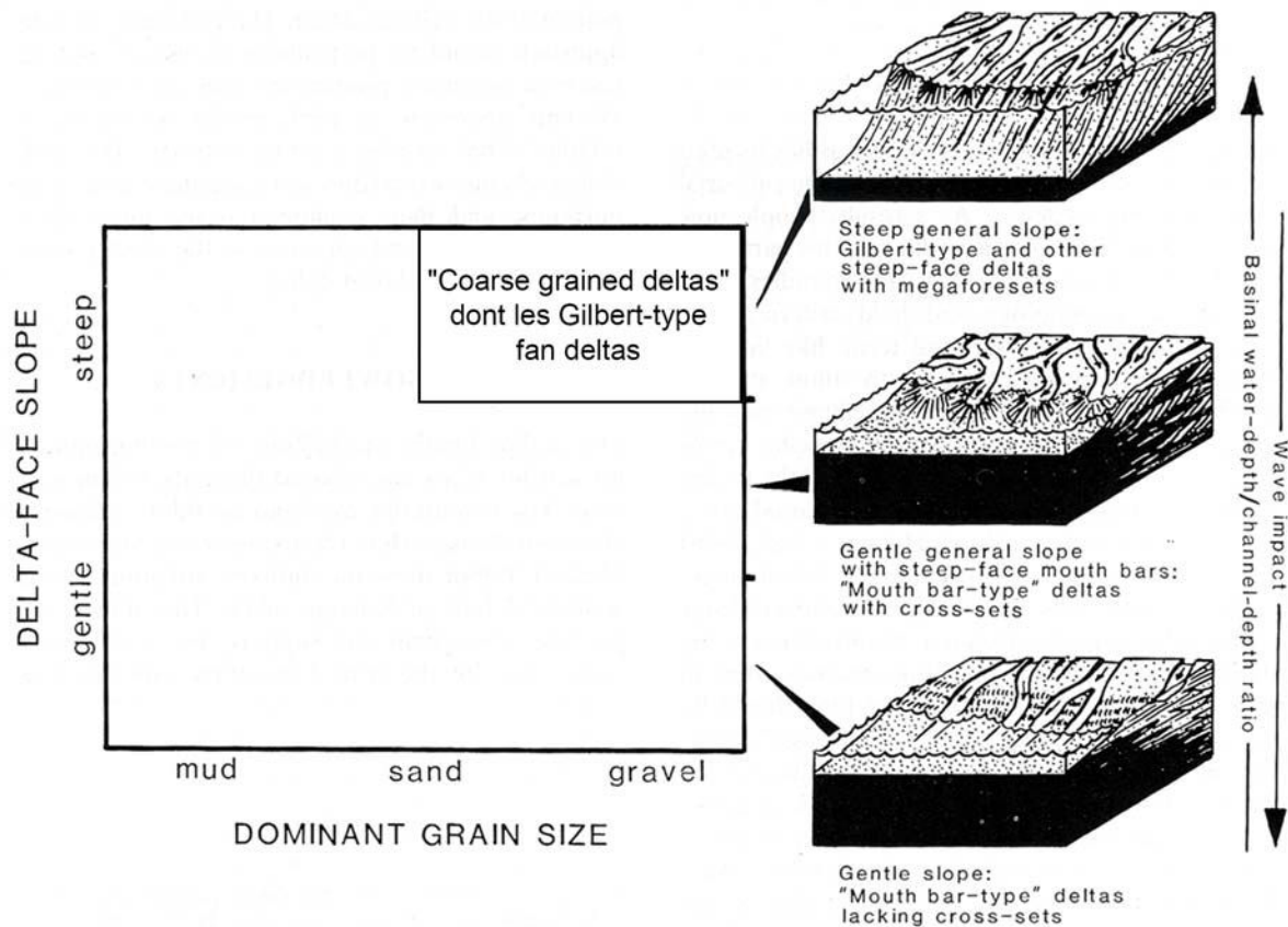
Figure 3.3 : Classification modifiée de Nemec (1990b) basée sur le diagramme bivariant de Corner et al. (1990) utilisant à la fois la pente des foresets du delta et la granulométrie des sédiments à la sortie du système distributaire.
