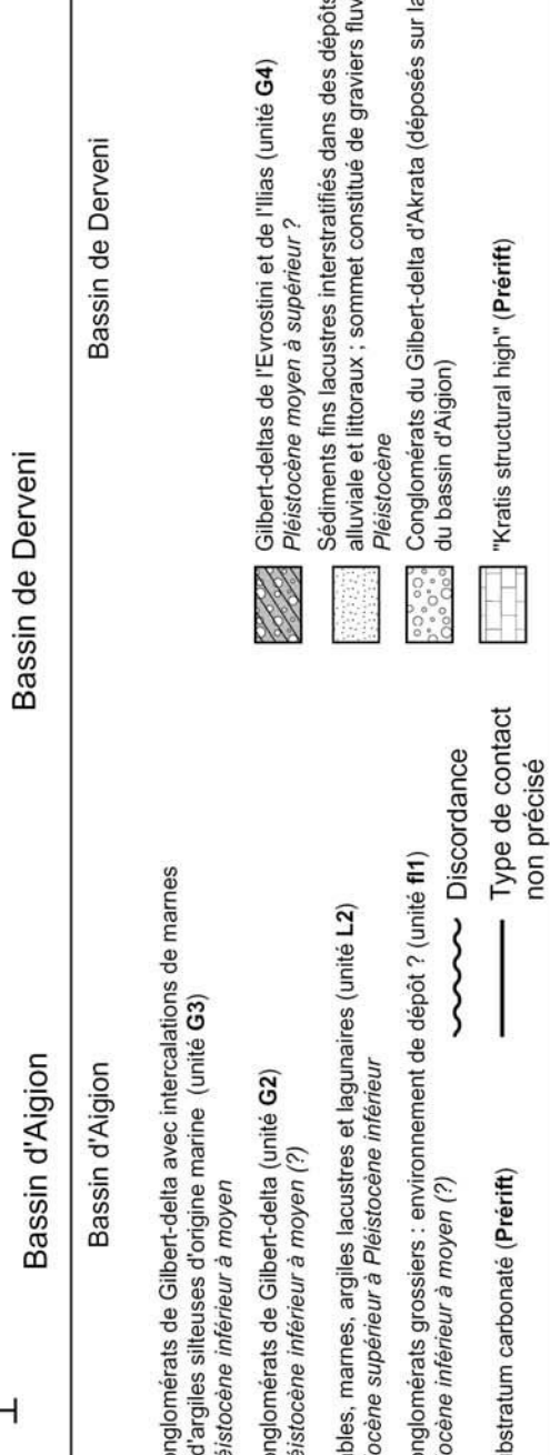
Figure 2.29 : Colonnes stratigraphiques synthétiques des bassins a) d'Aigion et de b) Derveni d'après les données de Ghisetti & Vezzani, 2004. Des corrélations sont proposées entre le découpage stratigraphique de Ghisetti & Vezzani (2004) et celui de Ori (1989) (figure c) dans le bassin de Derveni. Les chiffres entourés disposés le long des logs correspondent aux étapes de dépôt définies par Ghisetti & Vezzani (2004).
