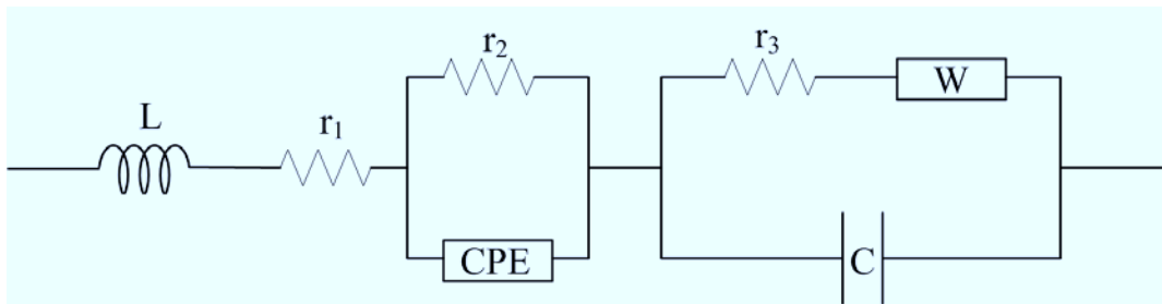
Figure 2.18 : Modèle avec composants électrochimiques [53] [54] [55]
