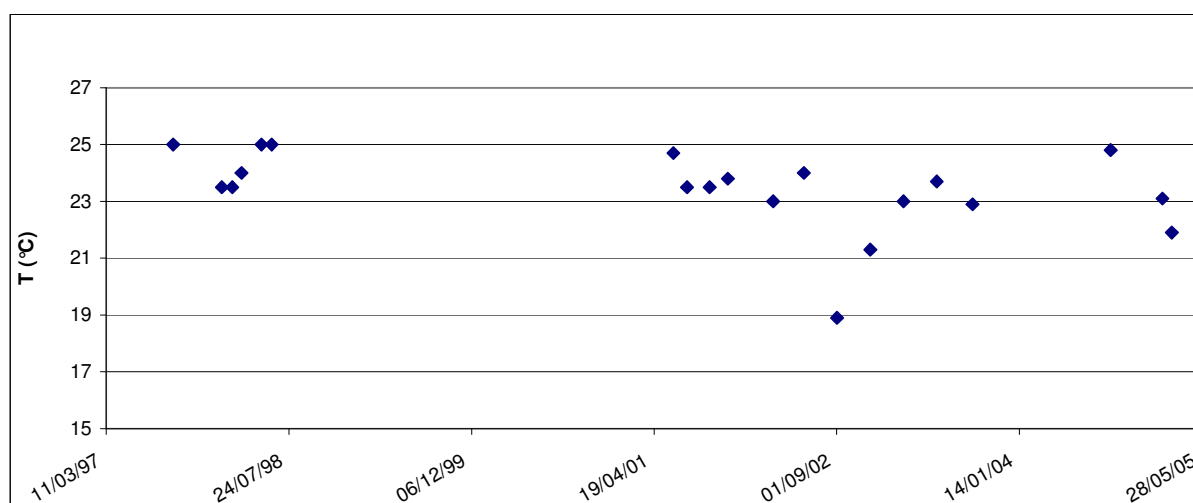
Figure 119 : Valeurs de la température des eaux issues de la mine au niveau du pompage de Fontanes entre 1997 et 2005
