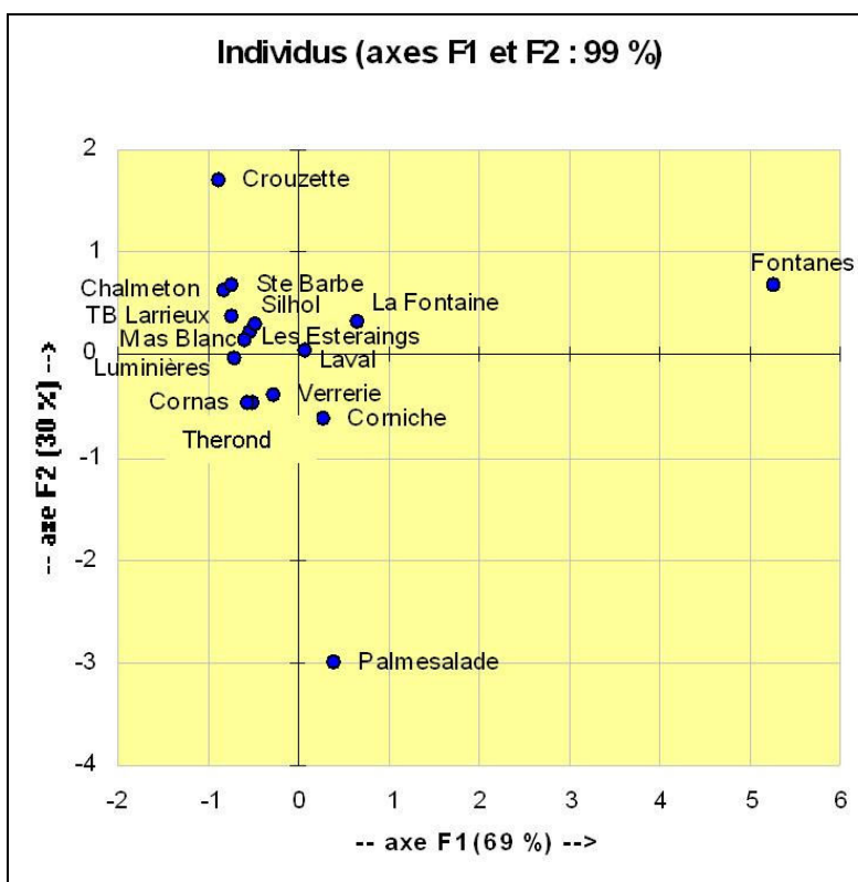
Figure 51 : Représentation de la répartition des individus (16 émergences) de l'ACP n°5 utilisant les variables pH, Fe 2+ , Mn 2+
