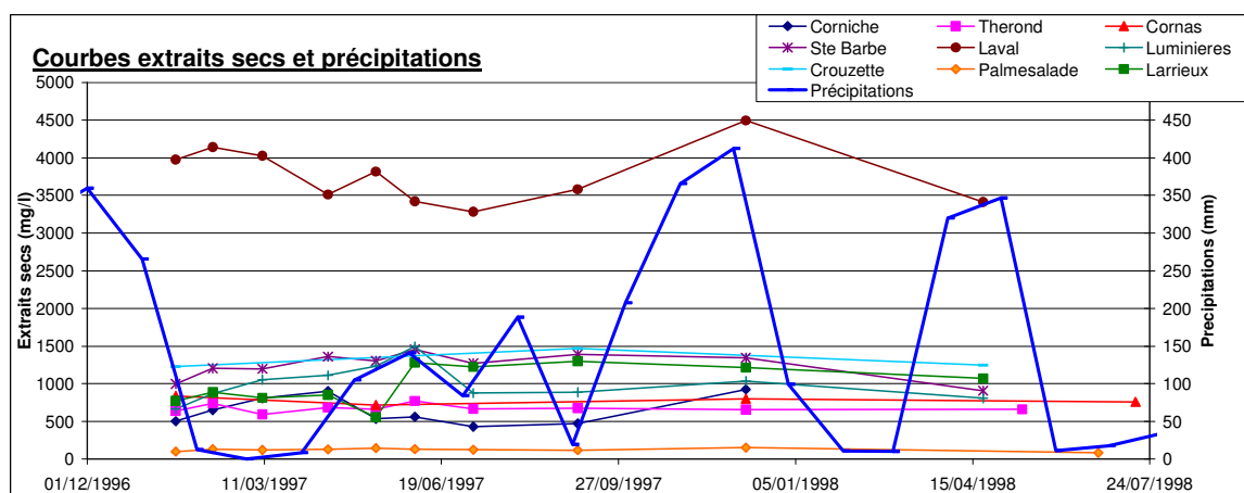
Figure 80 : Evolution temporelle des extraits secs pour les émergences de Corniche, Ste Barbe, Crouzette, Théron, Laval, Palmesalade, Cornas, Lumières et Larrieux.
