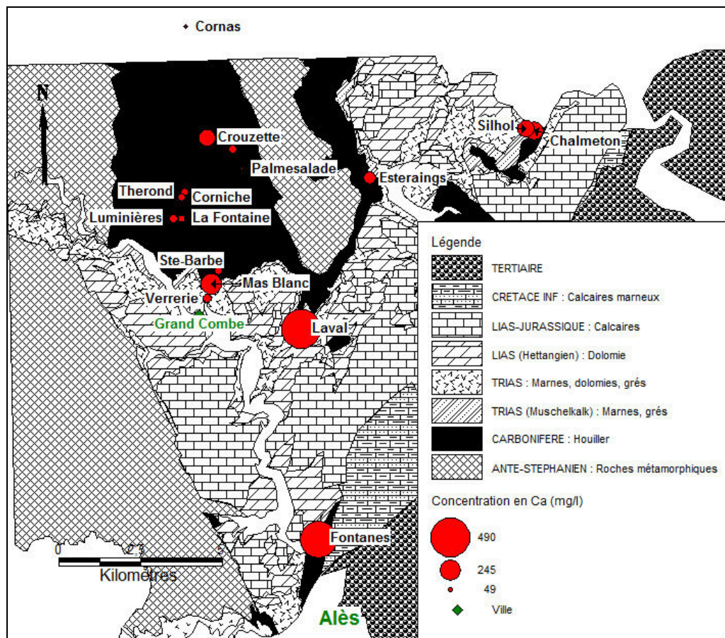
Figure 67 : Représentation des émergences en fonction de leurs concentrations en calcium
