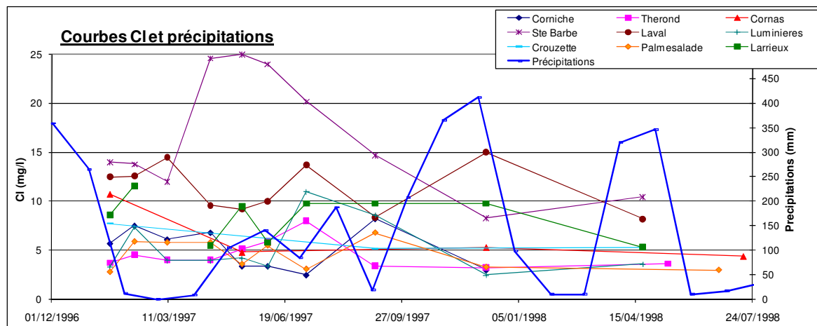
Figure 90 : Evolution temporelle de la concentration en chlorures pour les émergences de Corniche, Ste Barbe, Crouzette, Thérond, Palmesalade, Cornas, Luminières, Larrioux et Laval ainsi que les précipitations.
