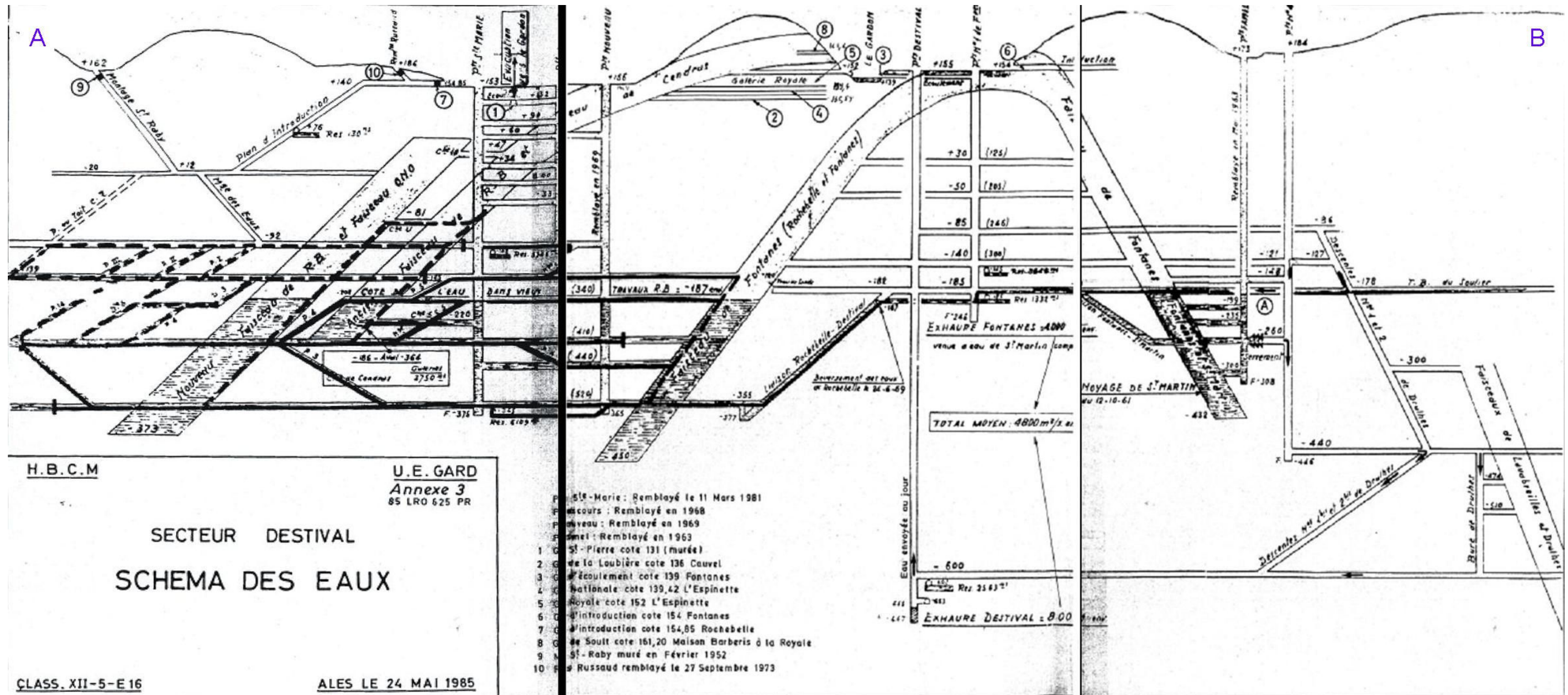
Figure 100 : Représentation de la coupe de l'exploitation de houille de Rochebelle-St Martin de Valgalgues (HBCM) dont la localisation se trouve Figure 131.
