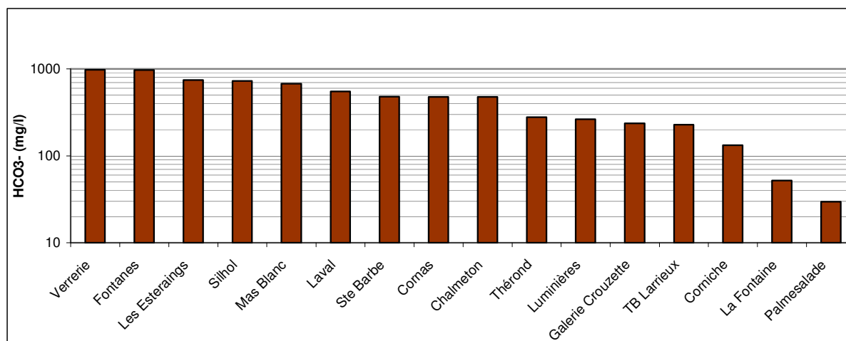
Figure 73 : Moyenne des concentrations en hydrogencarbonate par émergence
