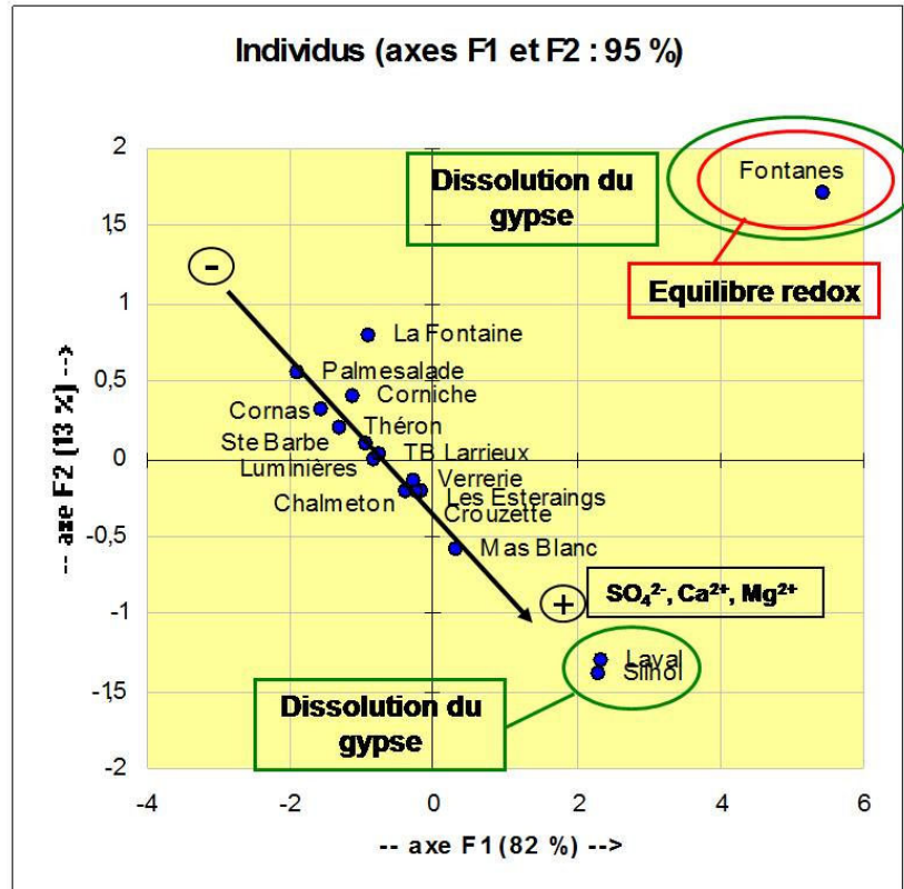
Figure 44 : Représentation de la répartition des individus (16 émergences) de l'ACP n°2 utilisant les variables \text{SO}_4^{2-} , \text{Ca}^{2+}+\text{Mg}^{2+} , \text{Fe}^{2+} et la somme des cations et des anions.
