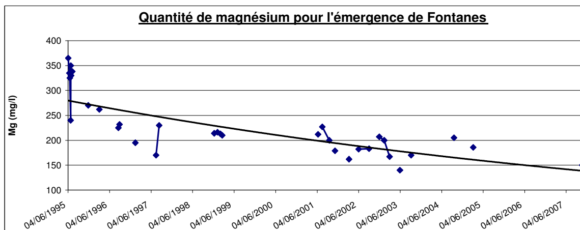
Figure 91 : Evolution temporelle de la concentration en magnésium pour l'émergence de Fontanes
