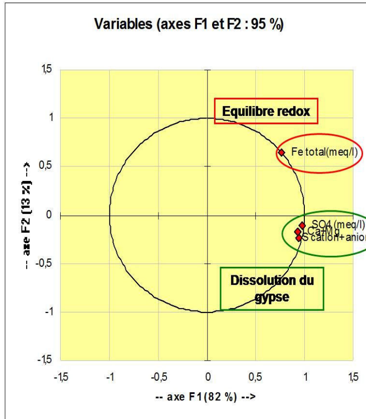
Figure 43 : Représentation de la répartition des variables ( \text{SO}_4^{2-} , \text{Ca}^{2+}+\text{Mg}^{2+} et \text{Fe}^{2+} et la somme des cations et des anions) de l'ACP pour les 16 émergences de l'ACP n°2
