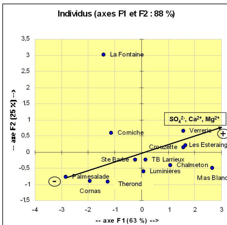
Figure 46 : Représentation de la répartition des individus (sans les émergences de Fontanes, Laval et Silhol) de l'ACP n°3 utilisant les variables SO 4 2- , Ca 2+ + Mg 2+ , Fe 2+ et la somme des cations et des anions.
