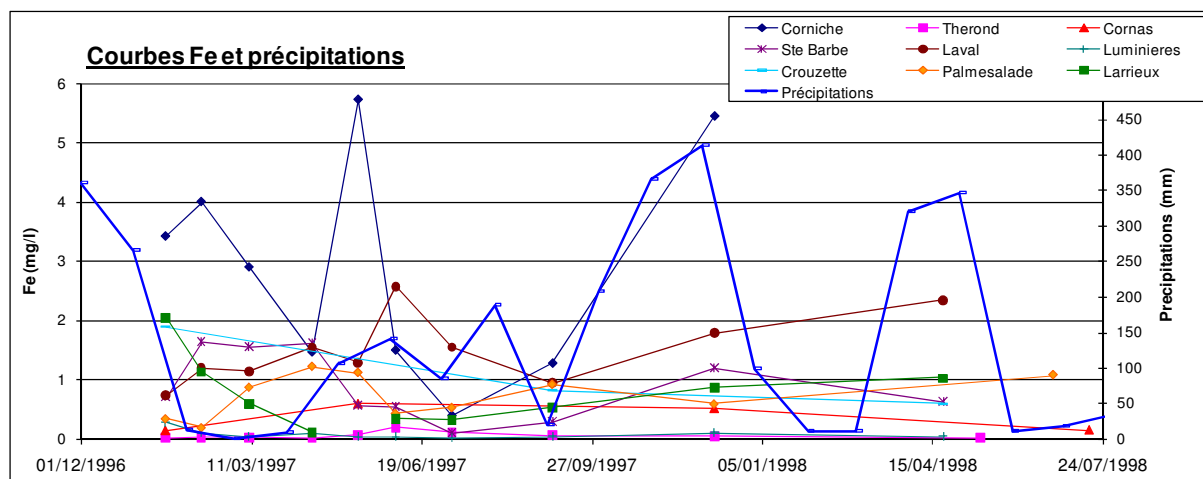
Figure 87 : Evolution temporelle de la concentration en fer pour les émergences de Corniche, Ste Barbe, Crouzette, Théron, Laval, Palmesalade, Cornas, Luminieres, Larrieux ainsi que les précipitations.
