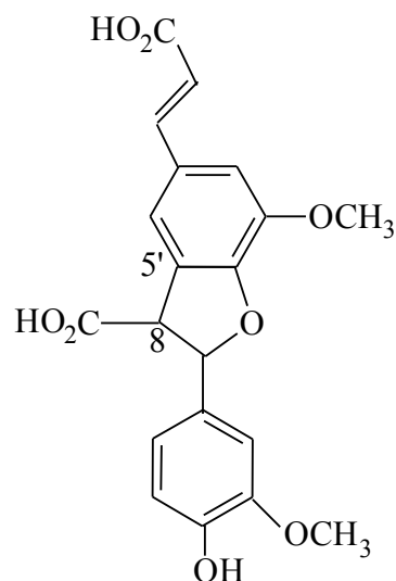
8-5'-benzofuran-DiF (P3) (incolore)
