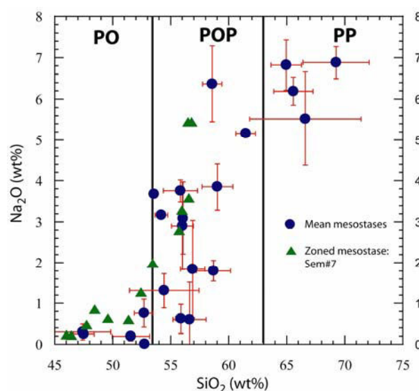
Figure VI.1 : Composition du verre de la mésostase de chondres de Semarkona (d'après Libourel et al. , 2003)
