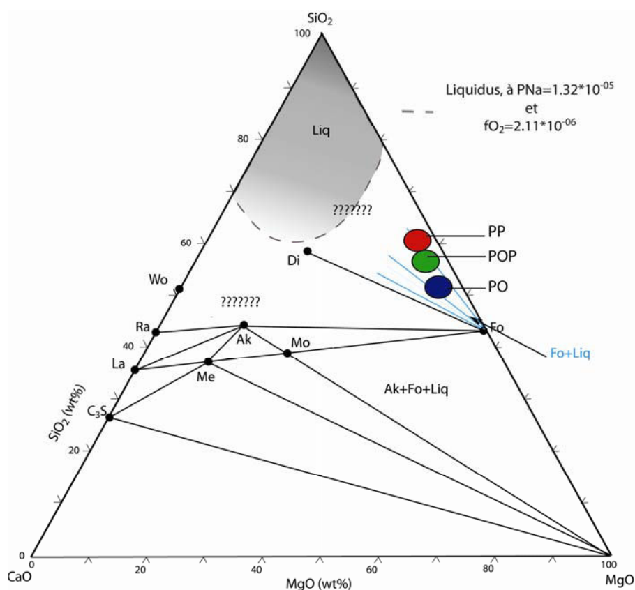
Figure VI.10 : Section isotherme à 1400°C, dans le pseudo système Na 2 O-CaO-MgO-SiO 2 , à P=1atm, sous une a_{\text{Na}_2\text{O}}=2.11 \cdot 10^{-7} ou [PNa= 1.32 \cdot 10^{-5} atm ; f_{\text{O}_2} = 2.11 \cdot 10^{-6} atm] , avec surimposés les équivalents dans ce système des chondres de Semarkona de type I
