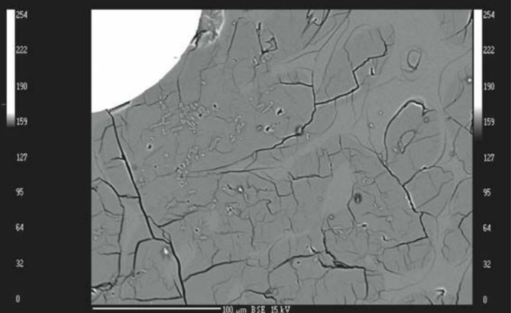
NS 2 - 1400 - ACMAS 20 - NAS1 - b
