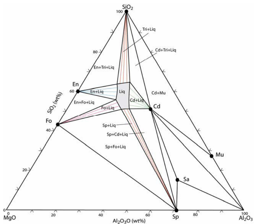
Figure VI.13: Section isotherme à 1400°C, a) dans le système MgO-Al 2 O 3 -SiO 2 , à P=1 atm.
