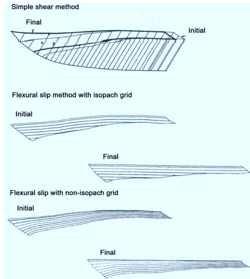
Figure 1.8 – Trois méthodes de restauration utilisées par le logiciel LOCACE. a) Cisaillement simple. b) Flexion-glisement avec une grille isopaque, préservant les aires et les longueurs des bancs parallèles à la grille. c) Flexion-glisement avec une grille anisopaque, utilisée pour des couches ayant un gradient d'épaisseur. Cette dernière méthode préserve les aires et toutes les longueurs. D'après Moretti et al. [1990] .
