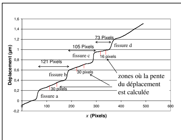
Figure 58. Profil du déplacement sur le plan moyen, noyau de filtrage : 11 pixels.
