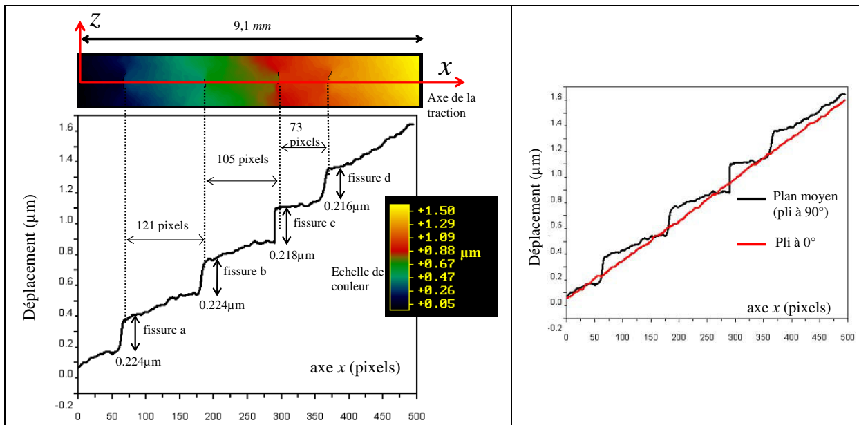
Figure 54. Carte de déplacement et profil tracé sur le plan moyen, 1 Pixel=18,22 μm,
