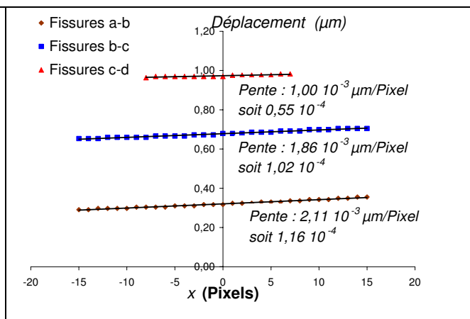
Figure 59. Détermination de la pente du déplacement entre deux fissures.
