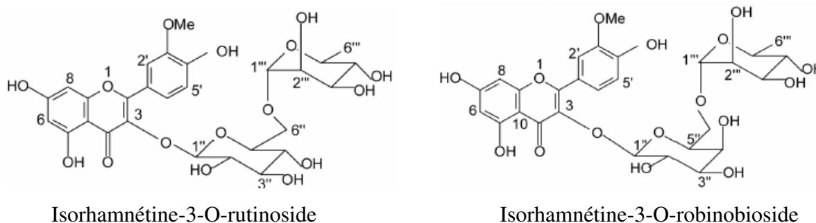
Figure 52: Structures des deux isomères, l'isorhamnétine-3-O-rutinoside et l'isorhamnétine-3-O-robinobioside
