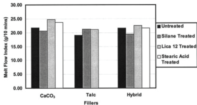
Figure A.20 : MFI de composites chargés avec des particules traitées et non traitées (15% de chaque type de charges pour les hybrides, sinon 30%) (Leong et al. (2005)).
