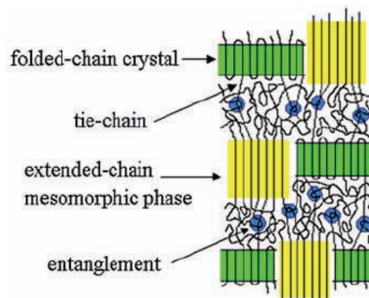
Figure 1.3.7 : Schéma général illustrant les effets d'un étirage uniaxiale sur un polymère semi-cristallin (cas d'une traction uniaxiale à faible vitesse de déformation) (Zuo et al. , 2007).
