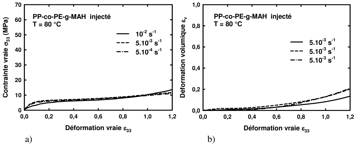
Figure 4.1.7 : Influence de la vitesse de déformation vraie sur le comportement mécanique en traction uniaxiale du PP-co-PE-g-MAH à 80 °C. a) Comportement vrai et b) Déformation volumique.
