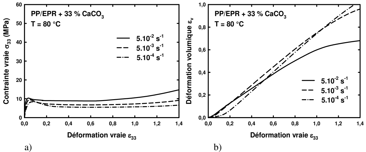
Figure 4.1.14 : Influence de la vitesse de déformation vraie sur le comportement mécanique en traction uniaxiale du PP/EPR chargé \text{CaCO}_3 à 80\text{ }^\circ\text{C} . a) Comportement vrai et b) Déformation volumique.
