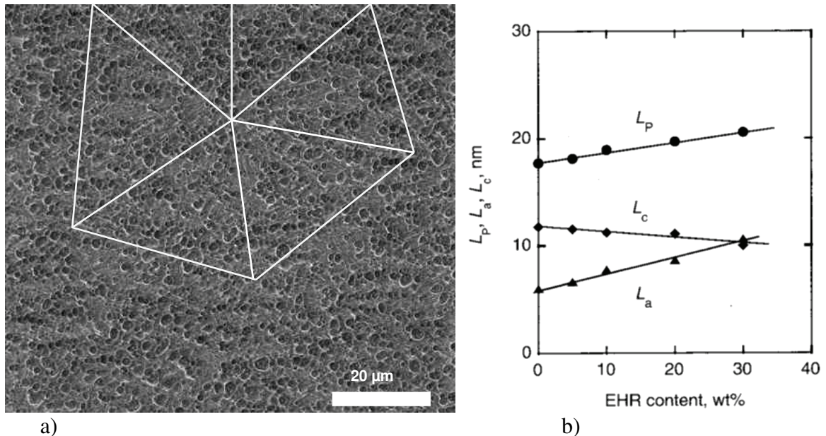
a) Observation au microscope électronique à balayage du cœur d'une plaque injectée de PP/EPR. Dispersion homogène des nodules d'EPR au sein de la structure cristalline sphérolitique de la matrice de polypropylène.
