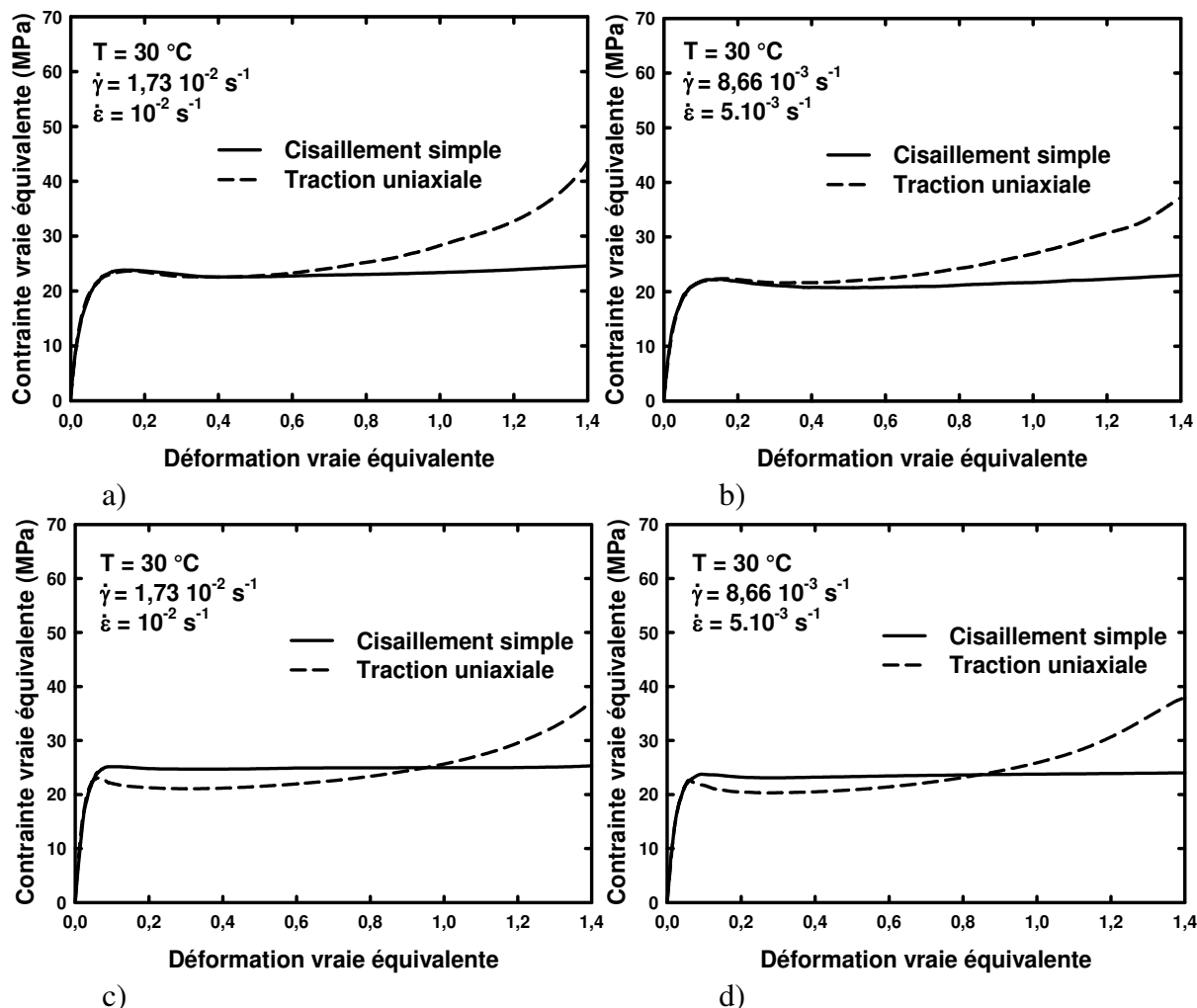
Figure J.1 : Comparaison à 30 °C des comportements vrais en traction uniaxiale et en cisaillement simple selon le critère de plasticité de Von Mises : a) et c) à 1.10^{-2} \text{ s}^{-1} et b) et d) à 5.10^{-3} \text{ s}^{-1} pour le PP-co-PE-g-MAH et le PP/EPR respectivement.
