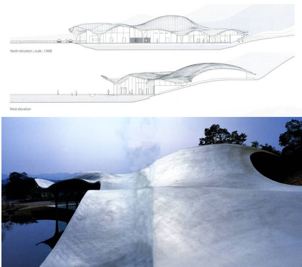
Figure 228. « Funeral Hall » de l'architecte Japonais Toyo Ito ("Roof Dynamics", 2008).
