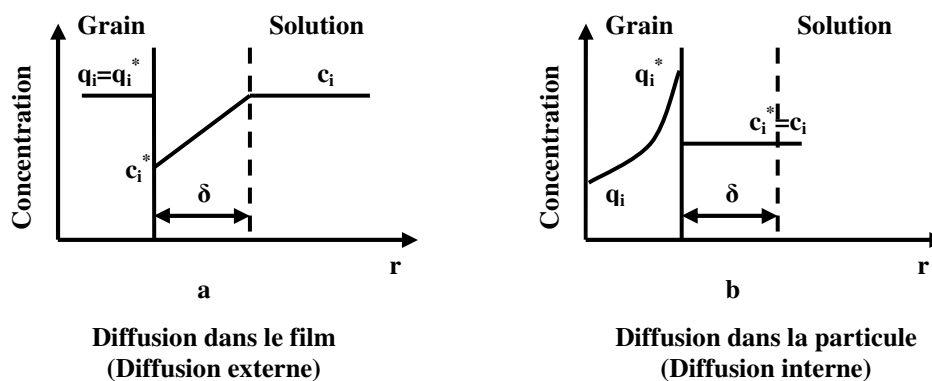
Figure 1-3: Deux types de limitation par la diffusion : a : diffusion dans le film ; b : diffusion dans la particule)
