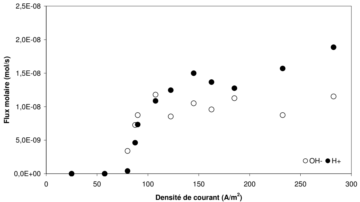
Figure 3-36: Flux molaires et concentration des ions H^+ et OH^- en régime stationnaire en fonction de la densité de courant dans le cas de la dissociation de l'eau dans une membrane échangeuse de cations (MC), i_{lim}=83,3 A/m^2
