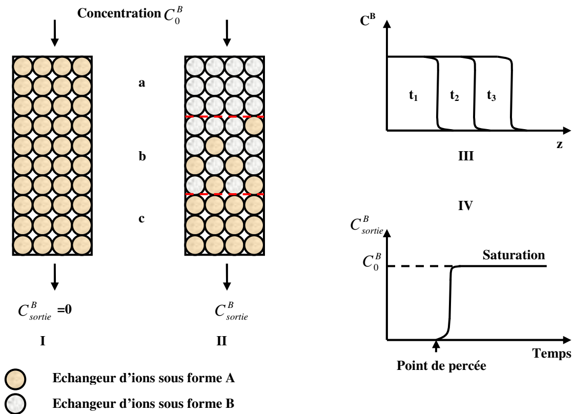
Figure 1-1: I : Permutation d'ions par une colonne; II : Front de saturation dans une colonne de résine; III : Propagation d'un front de saturation dans la colonne (isochrone) ; IV : Front de percée de saturation.
