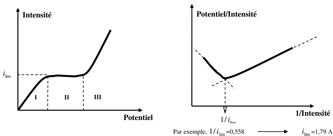
Figure 3-2: A (à droite) Courbe intensité/potentiel; B (à gauche) Principe de détermination du courant limite
