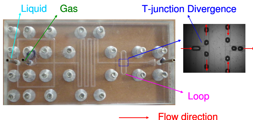
图 4-81 复杂微通道内流体流动示意图
