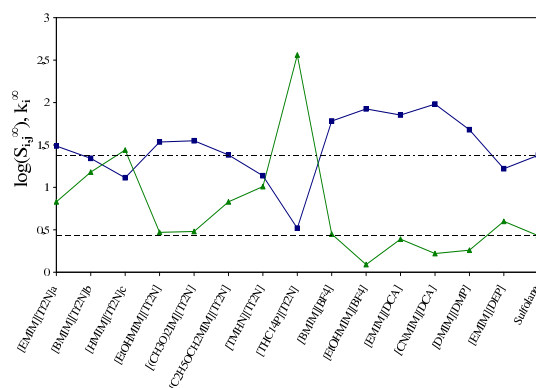
Figure II.7 – Influence du cation sur les valeurs de S_{i,j}^{\infty} et k_i^{\infty} pour différents liquides ioniques. —■—, S_{i,j}^{\infty} heptane,benzène ; —▲—, k_i^{\infty} benzène ; - - -, S_{i,j}^{\infty} heptane,benzène dans le sulfolane ; - - -, k_i^{\infty} benzène dans le sulfolane. a : [8] ; b : [59] ; c : [60].
