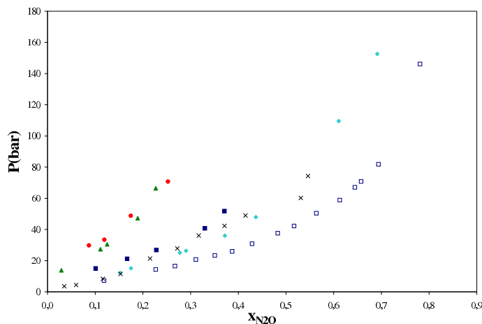
Figure IV.8 – Solubilité du N_2O dans les différents liquides ioniques à 40\text{ }^\circ\text{C} . \blacksquare , [BMIM][BF_4] ; \blacktriangle , [BMIM][SCN] ; \bullet , [DMIM][MP] ; \blacklozenge , [(OH)_2IM][Tf_2N] ; \square , [(CH_3CH_2O)_2IM][Tf_2N] et \times , TEGMME [21].
