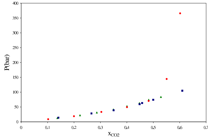
Figure IV.3 – Solubilité du CO 2 dans le LI [BMIM][BF 4 ] à 40°C. ■, ce travail ; ▲, AKI [6] ; ●, KROON [7].
