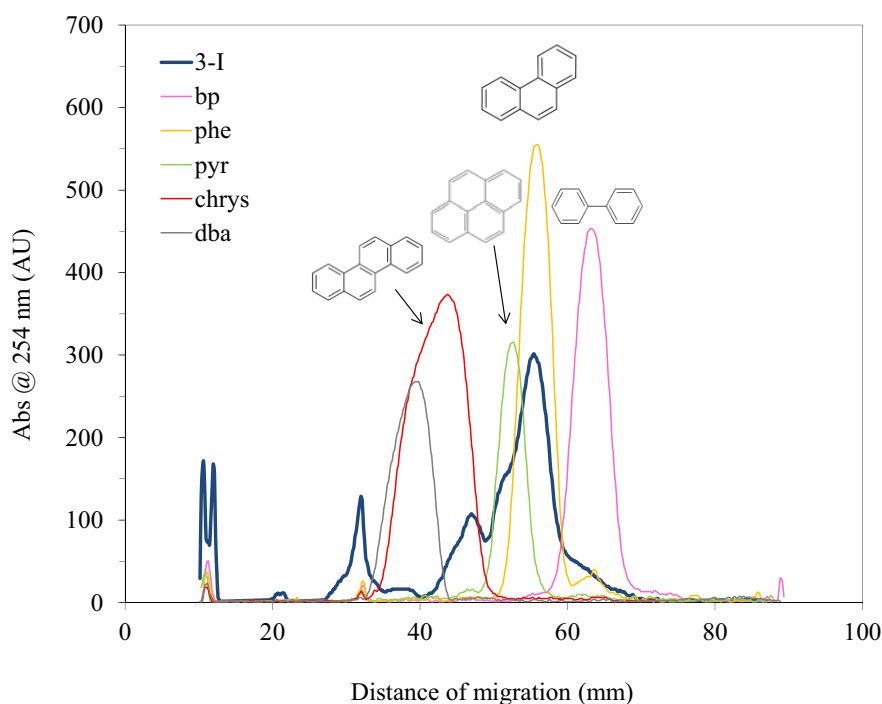
Figure 18: Chromatogramme de l'échantillon 3-I (Fe/olivine) et de 5 étalons sur plaque HPLTC Silica gel 60 \text{NH}_2 \lambda = 254 nm
