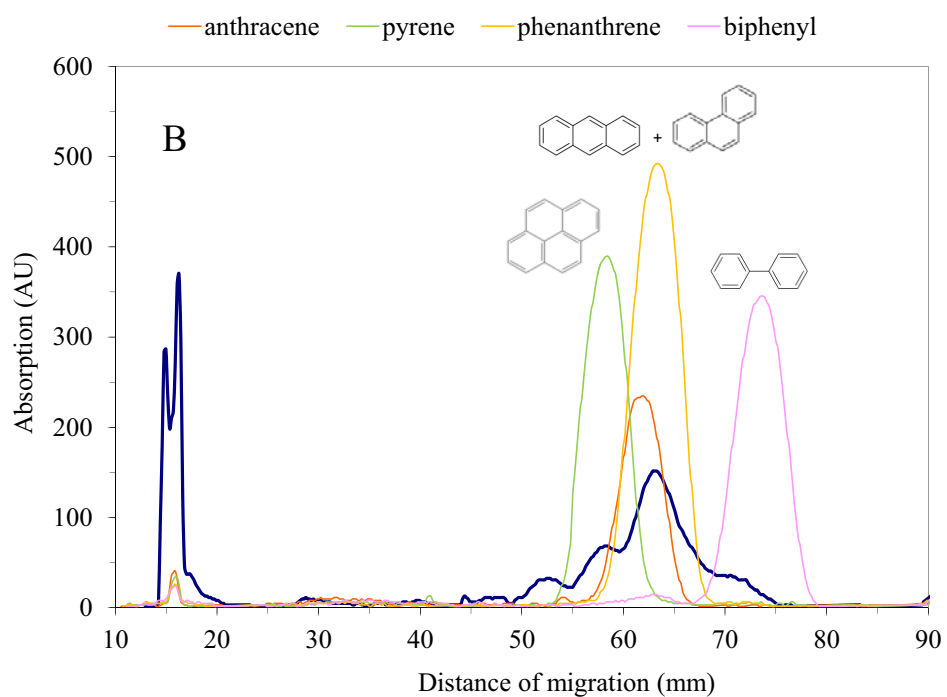
Figure 17: (A) Chromatogramme de l'échantillon 2-I (coque d'amandes sur lit d'olivine) par HPLTC Nano-SIL 20 et sur plaque RP-18 F 254 . (B) Chromatogramme du même échantillon, migration d'étalons sur plaque RP-18 F 254 ; migration avec du n-hexane sur 90 mm
