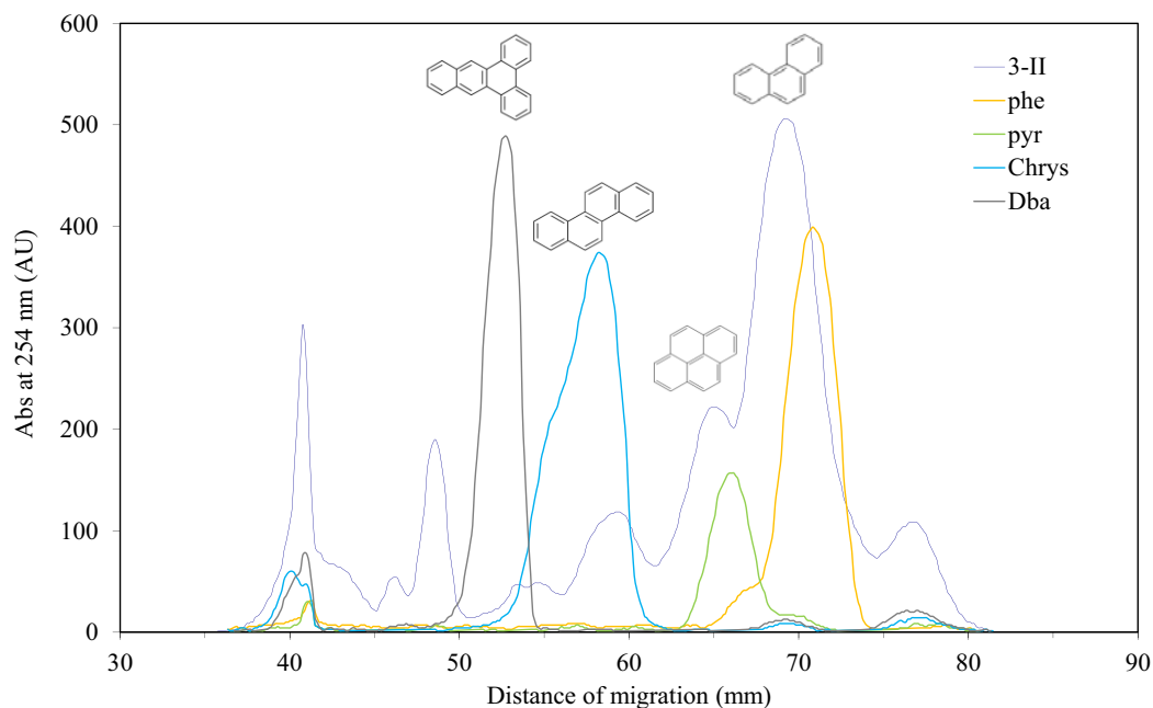
Figure 19: Chromatogramme de l'échantillon 3-II (Fe/olivine) et de 4 étalons sur plaque HPLTC Silica gel 60 RP-18 avec zone de concentration (migration à -23^{\circ}\text{C} ), \lambda = 254 \text{ nm}
