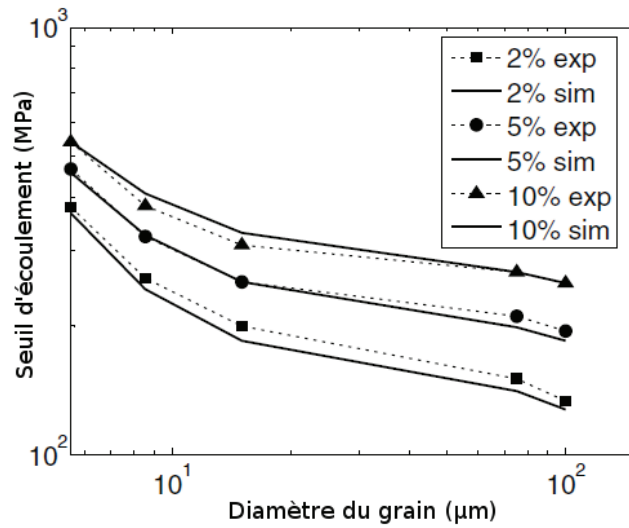
FIGURE 2.19 – Evolution du seuil d’écoulement, au cours du chargement pour des déformations de 2, 5 et 10%, en fonction de la taille de grain [PNB+09]
