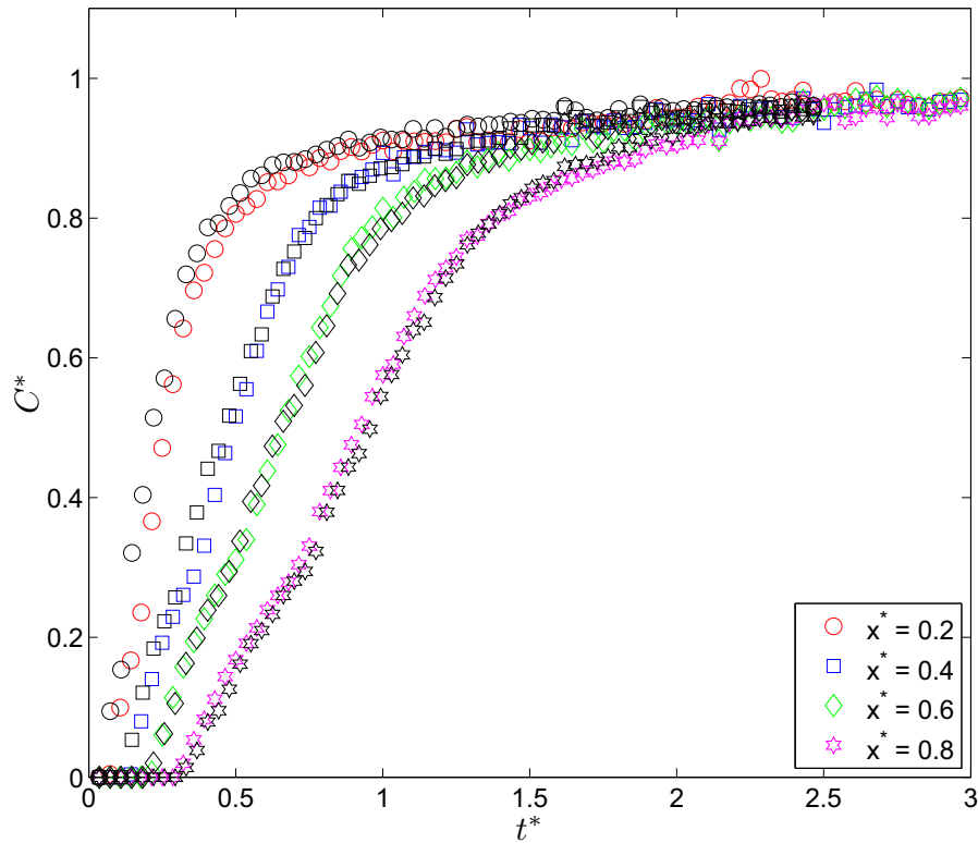
Fig. III.29 : Influence de la densité de traceur sur les profils de concentration (granit ( Pe = 3.46e+5 )).
