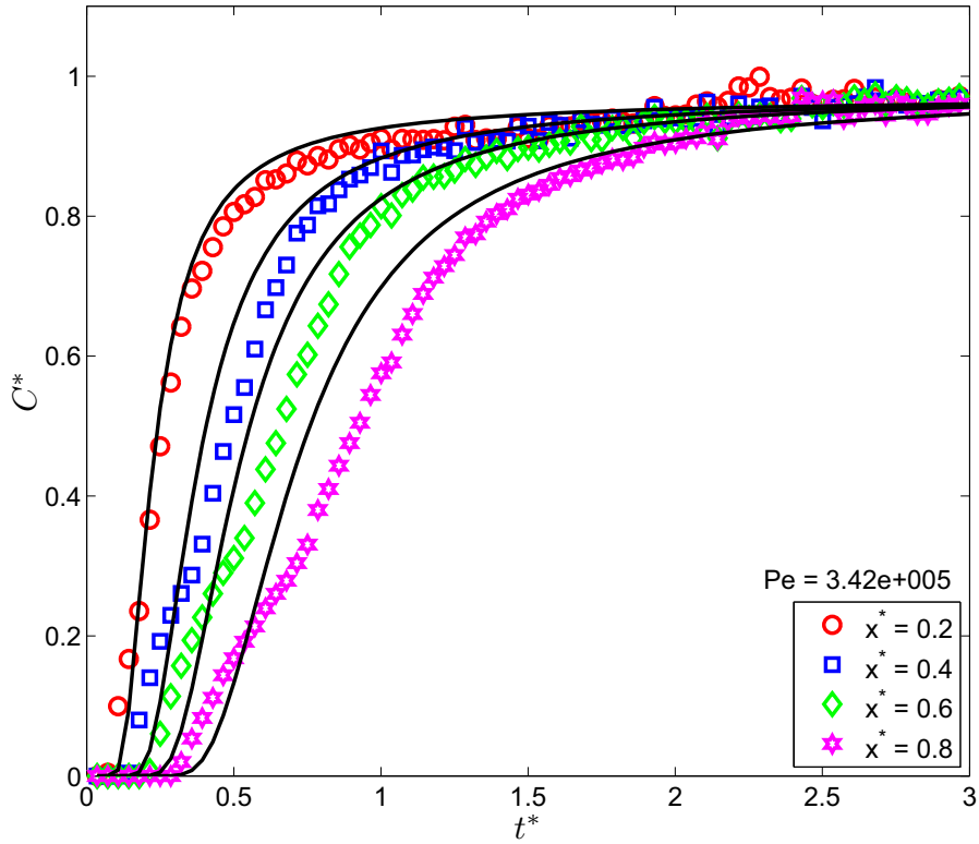
Fig. III.62 : Concentration en fonction de t^* (granit (distribution normale)).
