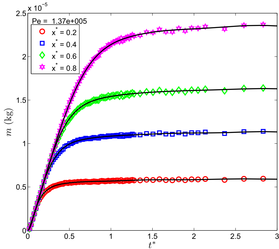
Fig. III.32 : Masse accumulée en fonction de t^* (grès des Vosges).
