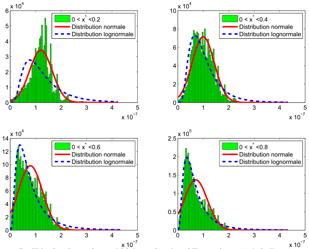
Fig. III.54 : Distributions des perméabilités entre l'entrée et différentes abscisses (grés des Vosges).
