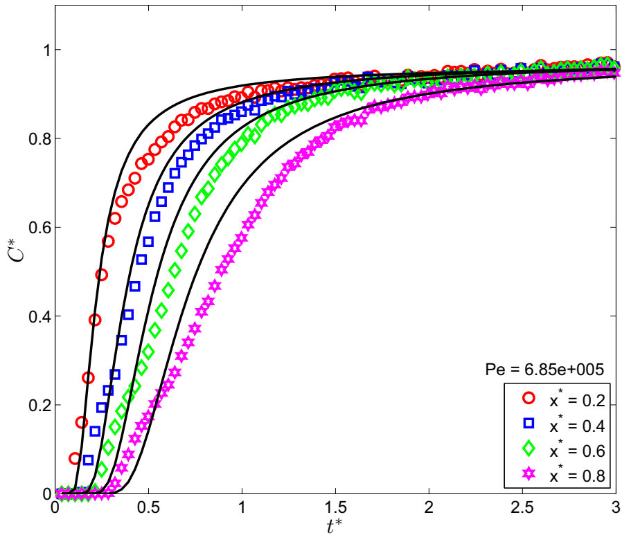
Fig. III.63 : Concentration en fonction de t^* (granit (distribution normale)).
