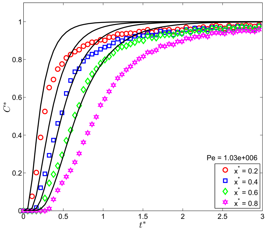
Fig. III.51 : Concentration en fonction de t^* (granit - Modèle classique de convection-dispersion).
