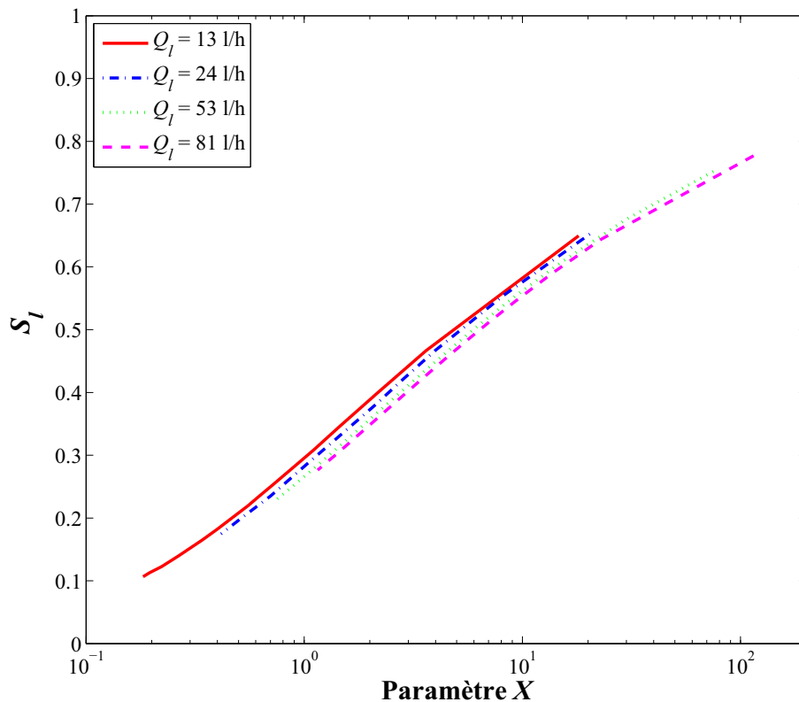
Fig. II.27: Saturation estimée en fonction du paramètre X (Grès des Vosges - Généralisation de la loi cubique complète).
