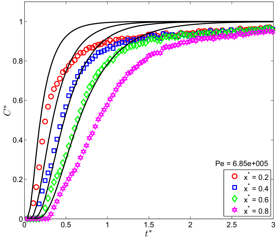
Fig. III.50 : Concentration en fonction de t^* (granit - Modèle classique de convection-dispersion).
