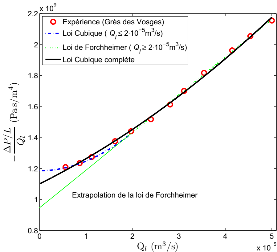
Fig. I.14 : Gradient de pression divisée par le débit ( -\Delta P/(LQ_l) ) en fonction du débit (Grès des Vosges - Les régimes d'écoulement associés aux lois cubique et Forchheimer).
