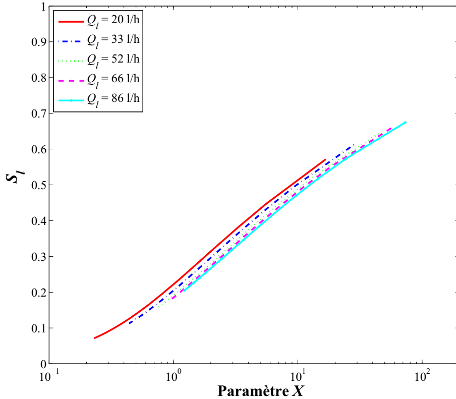
Fig. II.28 : Saturation estimée en fonction du paramètre X (Granit - Généralisation de la loi cubique complète).
