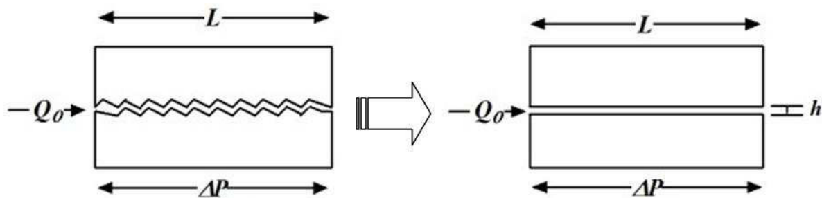
Fig. I.1 : Notion d'ouverture hydraulique d'une fracture rugueuse.
