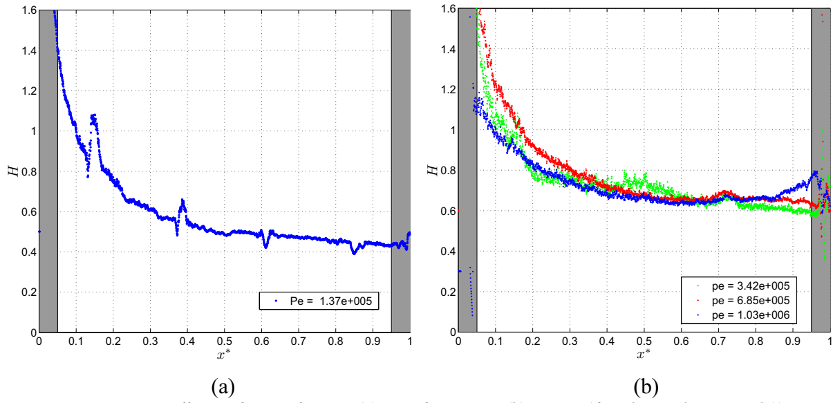
Fig. III.60 : Coefficient de stratification (a) grès des Vosges (b) granit (distribution log normale).
