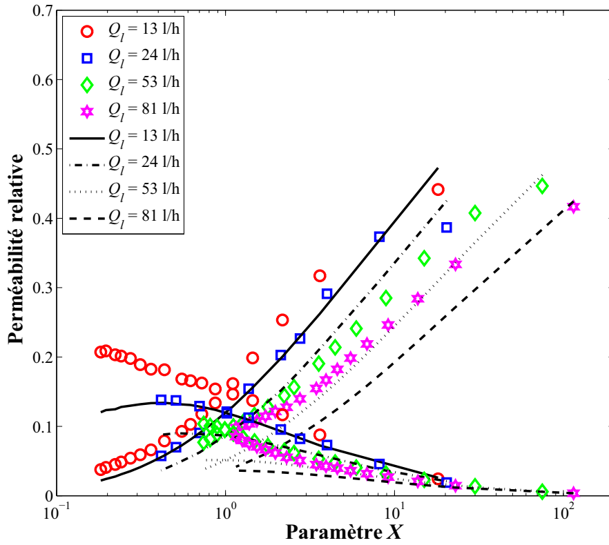
Fig. II.25 : Perméabilités relatives en fonction du paramètre X (Grès des Vosges - Généralisation de la loi de Forchheimer).
