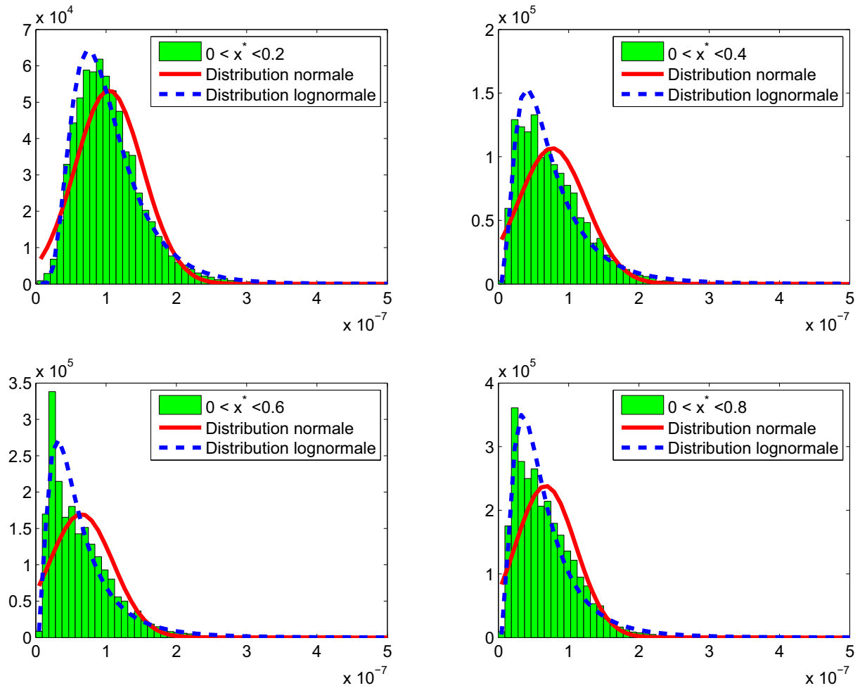
Fig. III.55 : Distributions des perméabilités entre l'entrée et différentes abscisses (granit).
