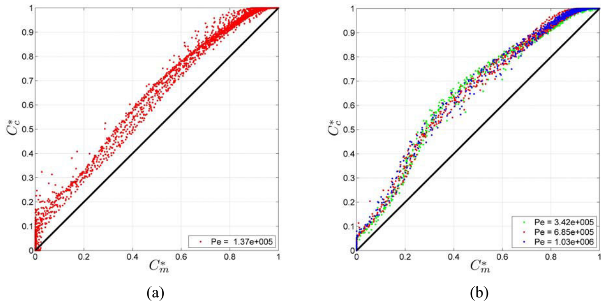
Fig. III.53 : Concentrations calculées en fonction des résultats expérimentaux a) grès des Vosges b) granit (Modèle classique de convection-dispersion).
