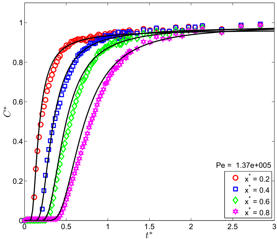
Fig. III.61 : Concentration en fonction de t^* (grès des Vosges (distribution normale)).
