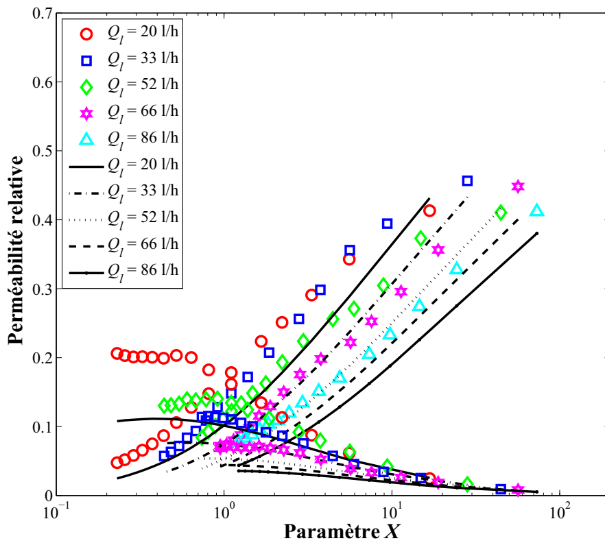
Fig. II.26 : Perméabilités relatives en fonction du paramètre X (Granit - Généralisation de la loi de Forchheimer).
