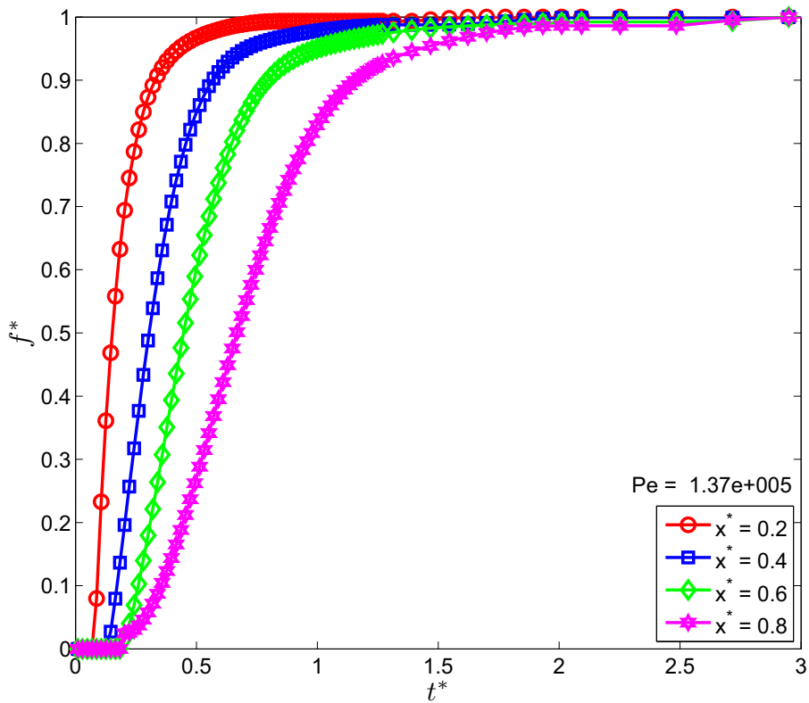
Fig. III.37 : Flux calculé en fonction de t^* (grès des Vosges).
