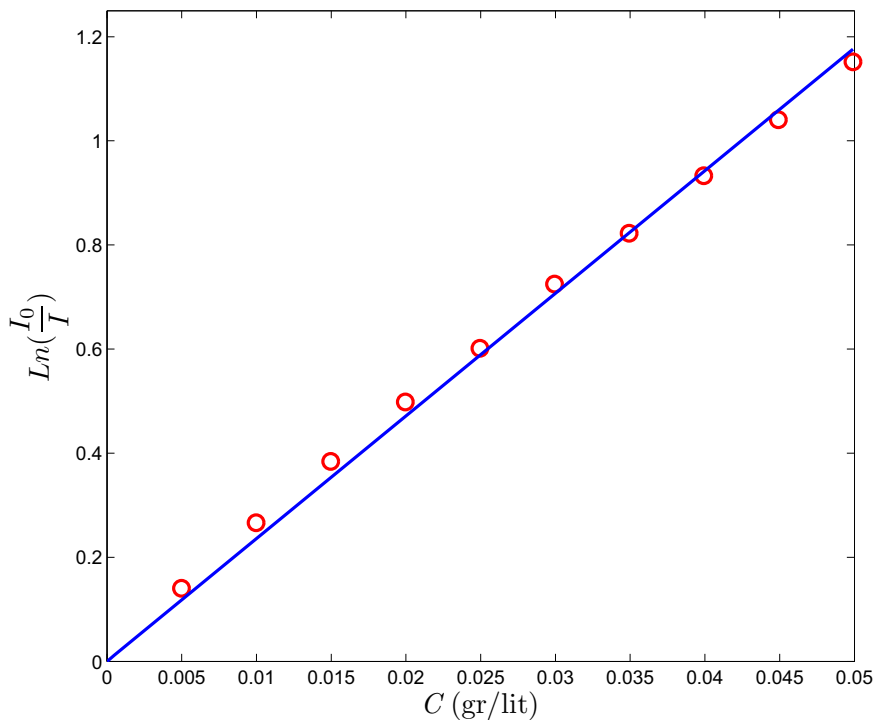
Fig. III.17 : La variation du niveau de gris mesuré en fonction de la concentration ( \zeta = 14.92 \text{ m}^2/\text{gr} )
