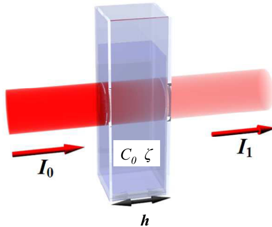
Fig. III.16 : Diminution de l'intensité d'un faisceau lumineux ( I_1 < I_0 ) traversant un milieu d'épaisseur l avec une constante d'absorption \zeta et une concentration initiale C_0 . (www.WIKIPEDIA.com)
