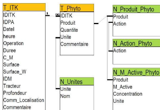
Figure 6 : tables et relations contenues dans le groupe d'entités opérationnelles « traitements phytosanitaires »
