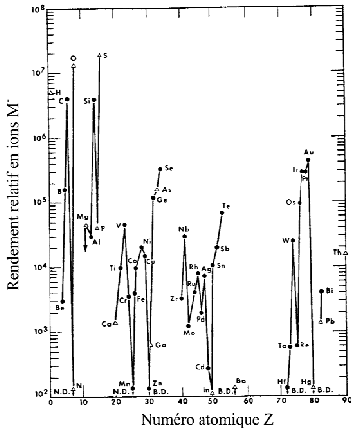
Figure 1.10. : Rendement relatif en ions secondaires négatifs pour un bombardement avec des ions primaires \text{Cs}^+ à 16.5keV et à incidence normale. Le symbole \Delta signifie qu'un échantillon composé a été utilisé pour l'élément en question [88].
