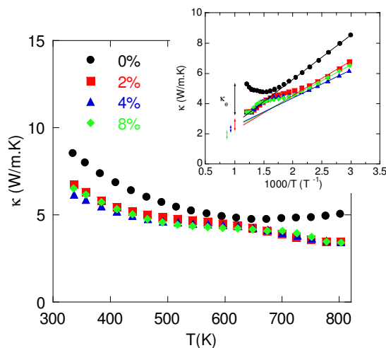
Figure 18 : Evolution de la conductivité thermique totale des composites \text{PbTe}/\text{CoSb}_3 en fonction de la température. L'insert met en évidence la prédominance des processus Umklapp entre 300 et 600 K par une dépendance de \kappa en 1/T . Les lignes tracées servent de guides pour les yeux
