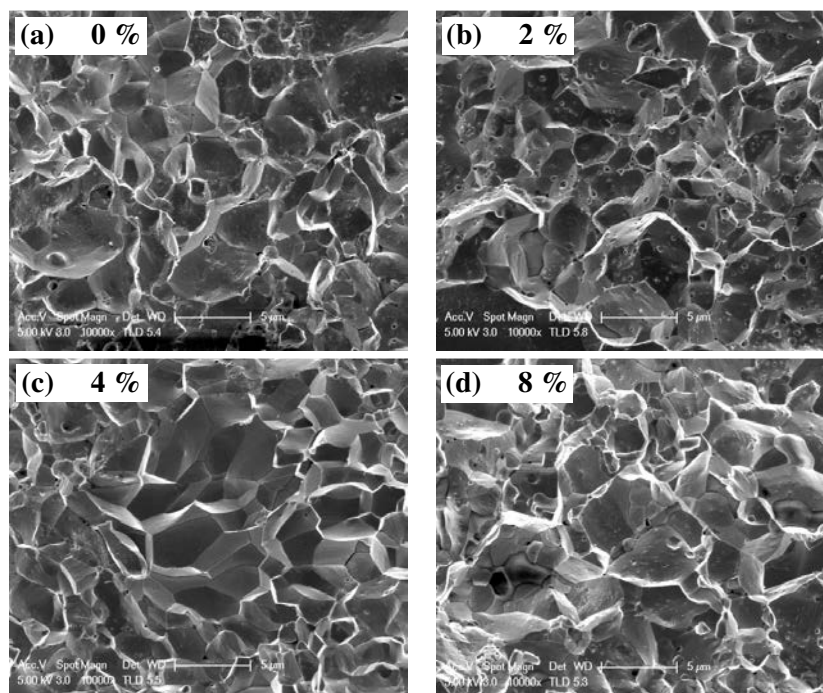
Figure 22 : Micrographies MEB réalisées sur des fractures (a) de CoSb 3 et des échantillons de la série PbTe/CoSb 3 (b) 2%, (c) 4% et (d) 8%. La taille de grains se situe autour de 2-5 µm pour tous les composés
