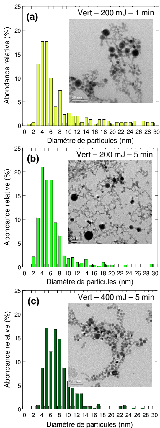
Figure 7 : Distribution en taille des particules obtenues pour des traitements à 532 nm après : a) 1 min à 200 mJ, b) 5 min à 200 mJ et c) 5 min à 400 mJ. Les images MET correspondantes sont en insert (échelle 50 nm)
