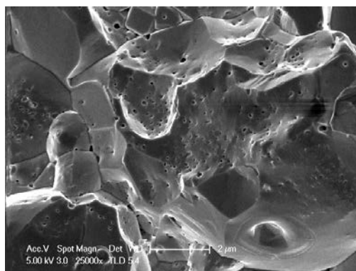
Figure 23 : Micrographie MEB (SE) de l’échantillon CoSb 3 réalisée sur une fracture. Le frittage SPS engendre une germination des grains visible par de petites protubérances de surface et une légère porosité intra-granulaire
