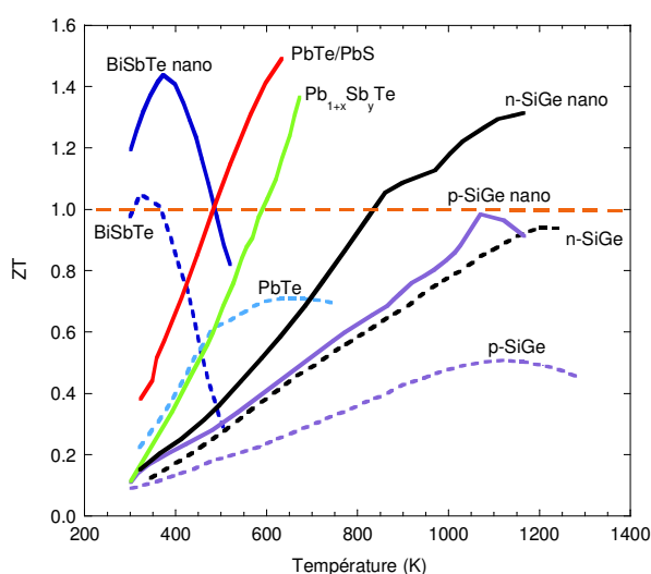
Figure 7 : Dépendance en température du facteur ZT de matériaux TE massifs conventionnels (courbes pointillées). Les courbes continues permettent de juger de l'impact de la nanostructuration sur les performances thermoélectrique [BiSbTe 64 ; PbTe/PbS 65 ; \text{Pb}_{1+x}\text{Sb}_y\text{Te} 66 ; n-SiGe 67 ; p-SiGe 68 ]
