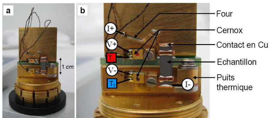
Figure 3 : a) Photos de la cellule TTO et b) zoom sur le montage. La barrette inférieure en cuivre est enserrée dans l'étai du puits thermique pour fixer le barreau au porte-échantillon. Les divers éléments (four et thermomètres) sont vissés aux contacts en cuivre. Le pulse de chaleur est délivré par un petit four résistif. Le courant d'intensité I traverse l'échantillon depuis le contact lié au four ( I+ ) jusqu'à celui du puits ( I- ). La tension résultante ( V+ , V- ) ainsi que la différence de température ( T_c , T_f ) sont prises au niveau des deux petites pièces en cuivre
