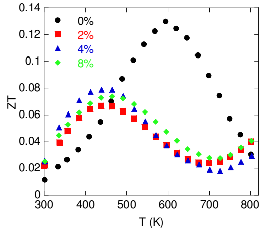
Figure 19 : Evolution du facteur de mérite adimensionnel ZT des composites à dispersion de \text{PbTe} de 300 à 800 K
