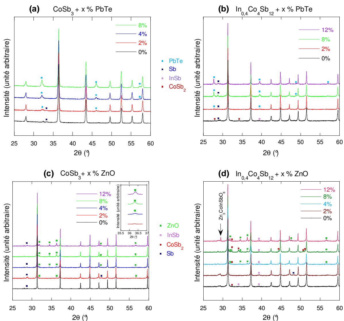
Figure 21 : Diagrammes de diffraction X des composites des séries (a) PbTe/ \text{CoSb}_3 analysés sur le D500 ( \lambda_{\text{Co}} ), (b) PbTe/ \text{In}_{0.4}\text{Co}_4\text{Sb}_{12} , (c) ZnO/ \text{CoSb}_3 et (d) ZnO/ \text{In}_{0.4}\text{Co}_4\text{Sb}_{12} analysé sur le D8 ( \lambda_{\text{Cu}} ). Les pics de diffraction des composites sont bien indexés sur ceux de leur matrice respective. Des pics supplémentaires correspondant soit au PbTe soit au ZnO apparaissent dans le domaine angulaire étudié et leurs intensités sont fonction de la quantité d'inclusions.
