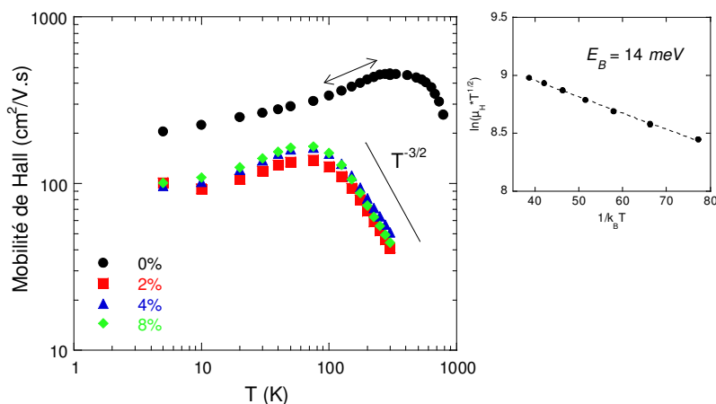
Figure 7 : Dépendance en température de la mobilité de Hall des composites \text{PbTe}/\text{CoSb}_3 . L'insert représente l'ajustement de la courbe du \text{CoSb}_3 selon l'équation de Seto (V-8) entre 100 et 250 K
