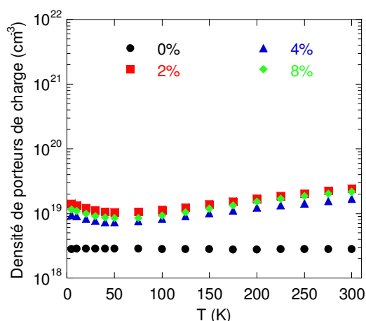
Figure 3 : Evolution de la concentration de porteurs en fonction de la température et du taux d'inclusions
