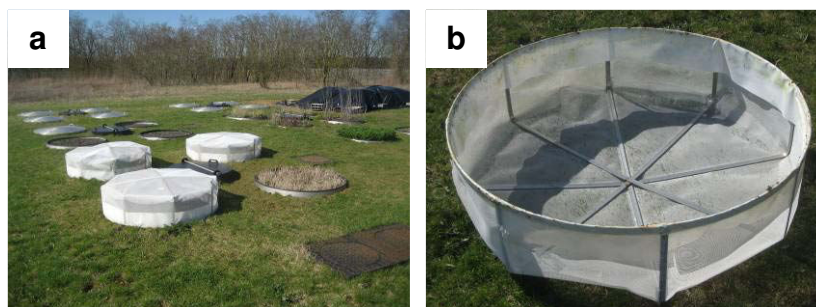
Figure 17. Photographies des cloches à lysimètres, a) vue d'ensemble des trois lysimètres, b) intérieur de la cloche et son armature métallique.
