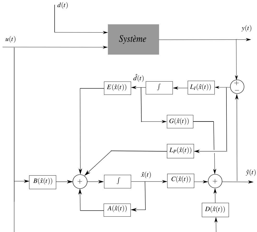
Figure 4.3 – Structure d'un observateur proportionnel-intégral (PI)
