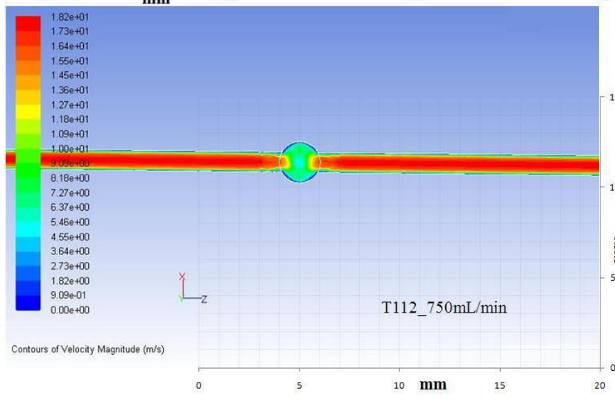
Figure VI. 12 : Champs de vitesse pour le mélangeur T112 à différents débits d'alimentation (surface A)
