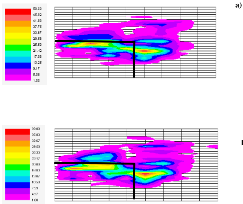
Figures 5 : nombre total des particules : a) injection aléatoire, b) pondérée par le débit. (RK2)
