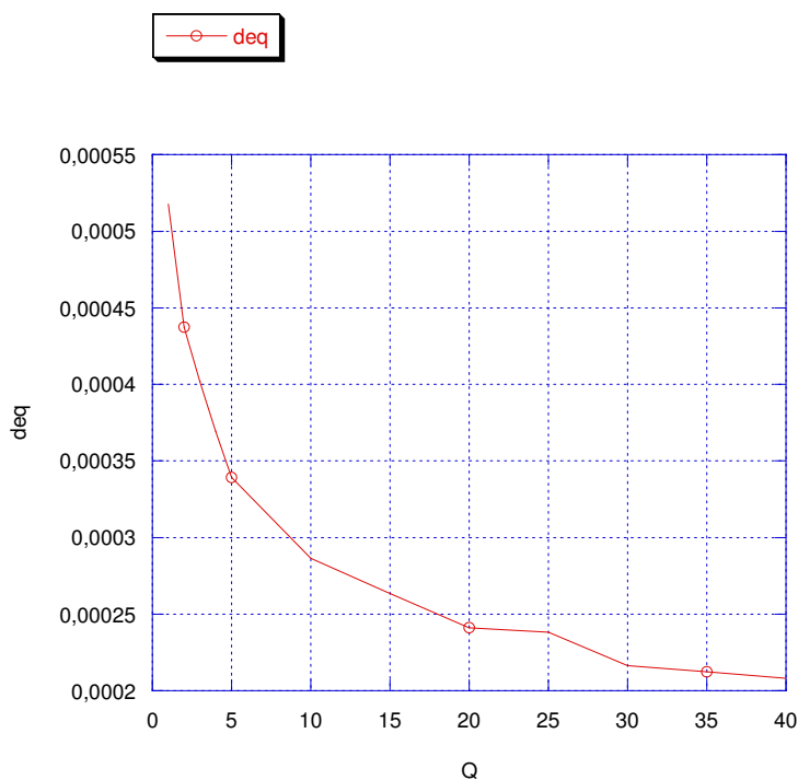
Figure III-20 : évolution du diamètre équivalent moyen en fonction du coefficient de restriction de croissance Q .
