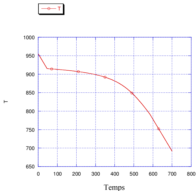
Figure III-13 : évolution de la température en fonction du temps.
