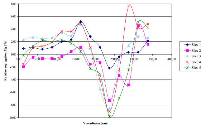
Figure II-36 : profils de ségrégation relative à Mg(%) suivant l'épaisseur (de la peau vers le centre, en mm).
