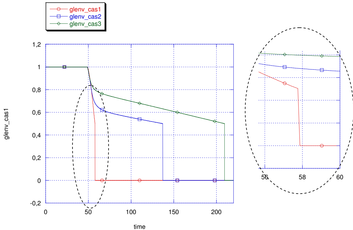
Figure III-43 : évolution de la fraction liquide extragranulaire (méthode d'injection de particules).
