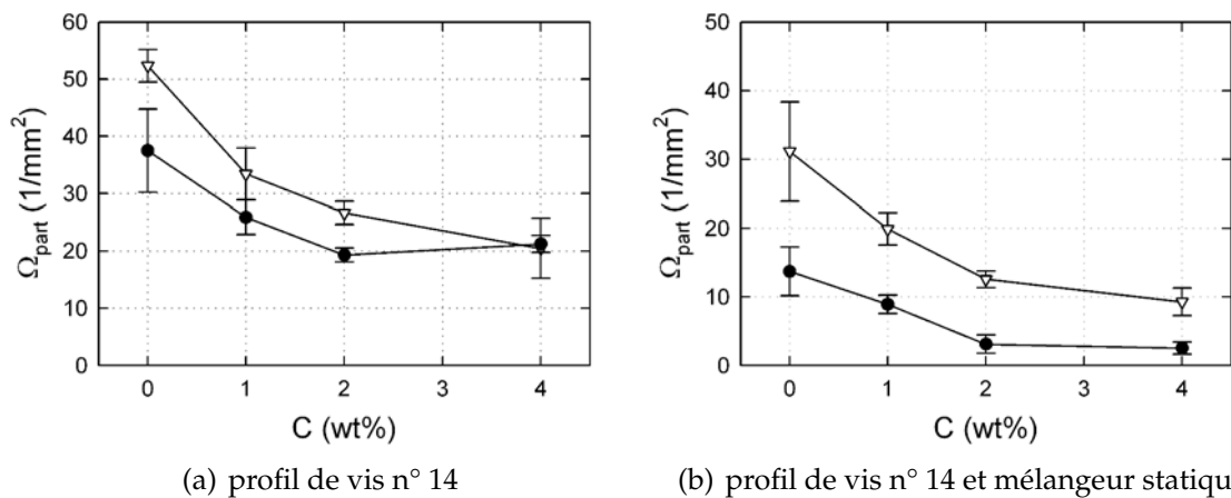
Figure 4.22. Influence du \text{CO}_2 et de la vitesse de rotation des vis sur la densité de particules selon la configuration d'extrudeuse ( Q_m=1.8 \text{ kg/h} ); N=100 \text{ min}^{-1} ( \nabla ), N=300 \text{ min}^{-1} ( \bullet )
