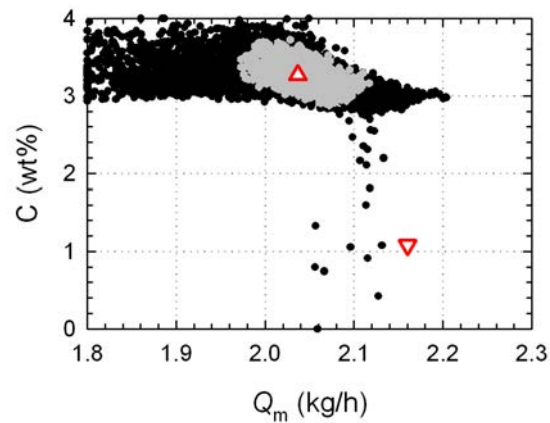
(c) Titre massique du CO 2 en fonction du débit de polymère
