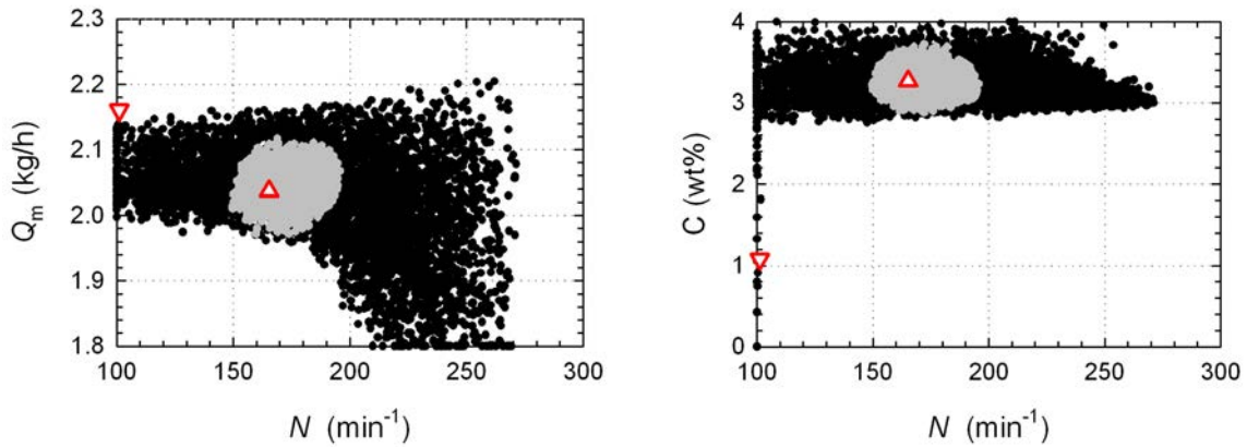
(a) Débit de polymère en fonction de la vitesse de rotation des vis
