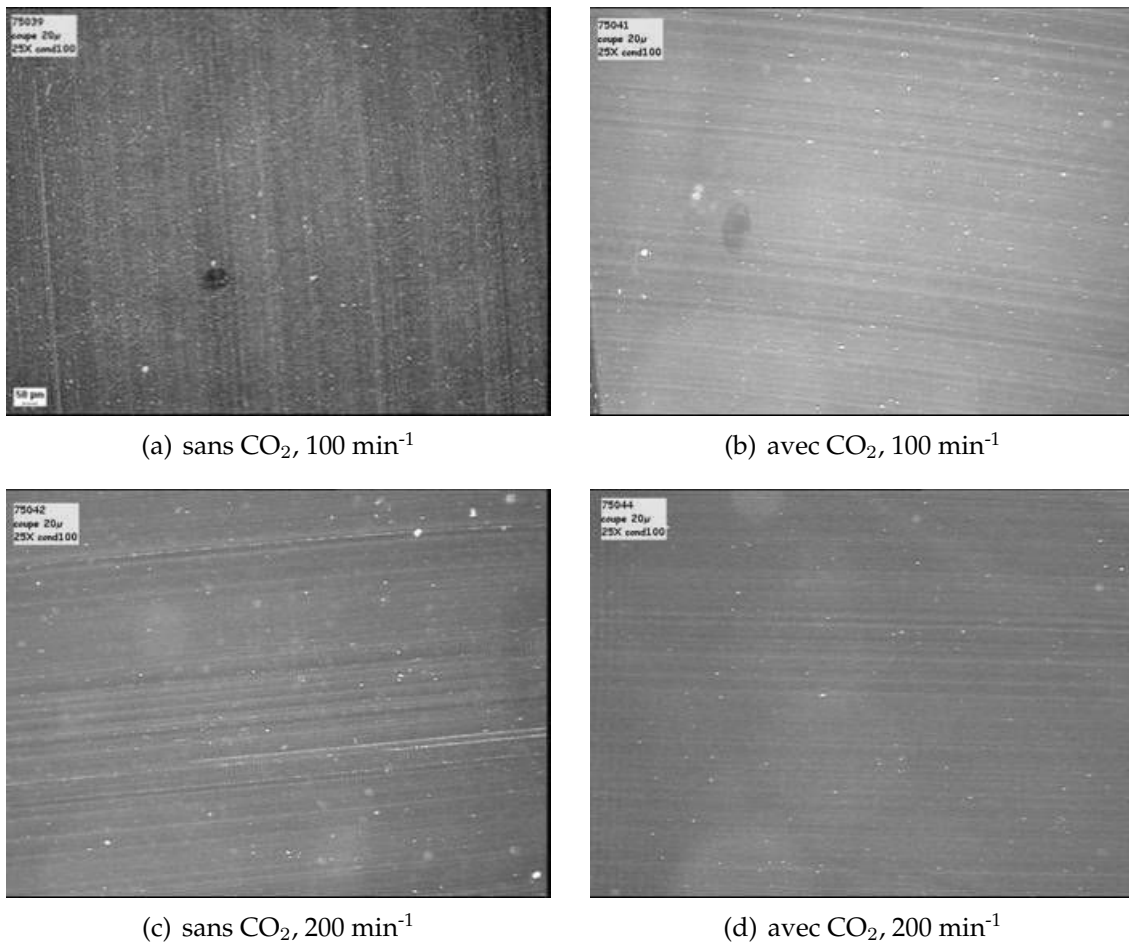
Figure 4.4. Comparaison des morphologies du PE2 après extrusion sans et avec CO 2 (profil n° 9)
