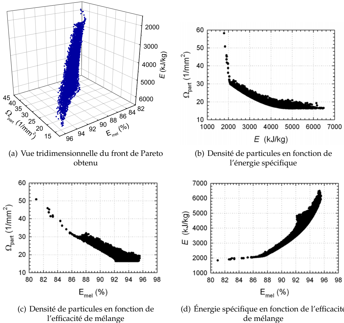
Figure 6.5. Front de Pareto (profil n° 14)
