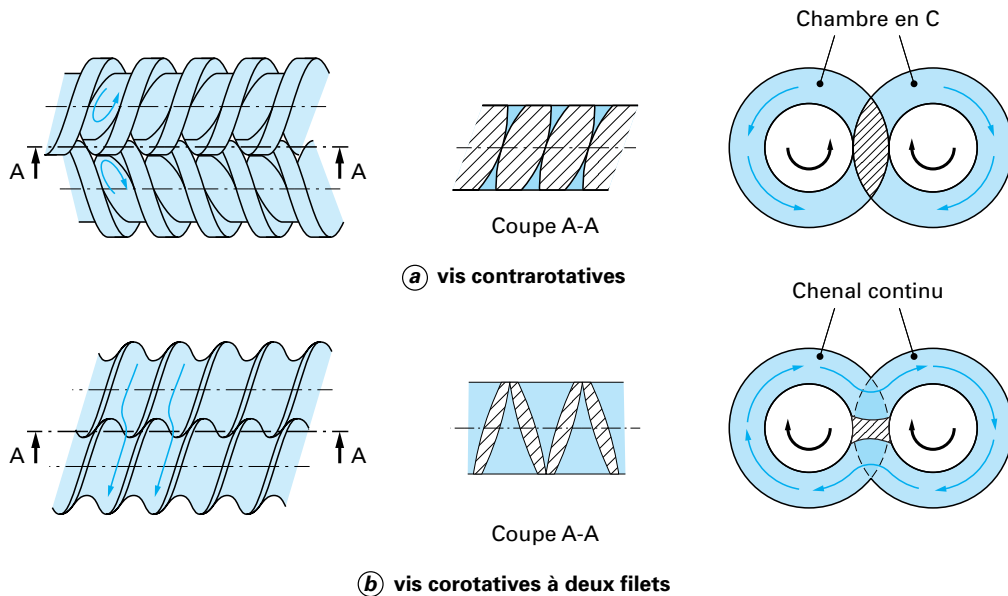
Figure 1.4. Géométrie et mode d'écoulement pour deux types de vis (Vergnes et Chapet, 2001)
