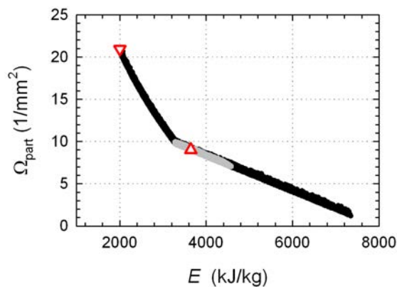
(c) Densité de particules en fonction de l'énergie spécifique
