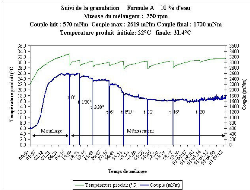
Figure 101. Suivi de la granulation de l'essai sur l'étude du temps de mûrissement
