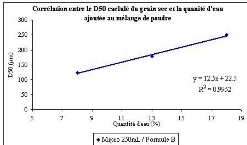
Figure 86. Corrélation entre la valeur de D50 du grain sec et la quantité d'eau ajoutée au mélange de poudre
