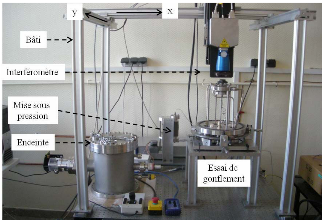
Figure II.41. Bâti de l'essai de gonflement.
