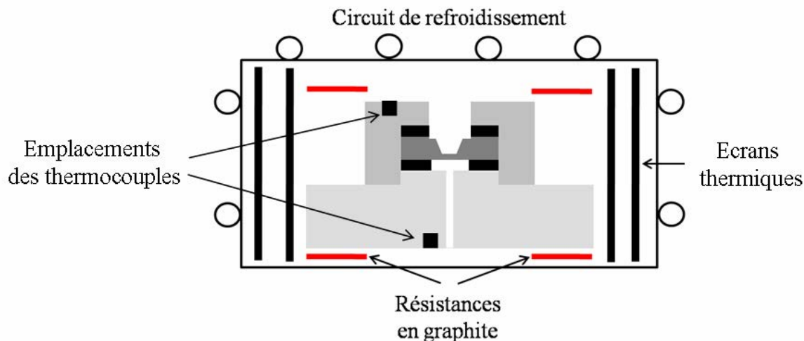
Figure II.31. Schéma du système de chauffage de l'échantillon.
