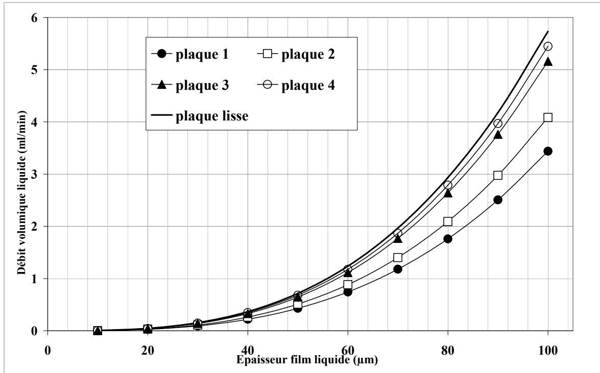
Figure II. 5: Influence de la structuration sur le débit nécessaire pour mouiller la plaque Liquide : éthanol ( \mu_L=1,08 \cdot 10^{-3} Pa.s et \rho_L=789 kg/m 3 à 20°C) (cf. Tableau II.2 pour les plaques)
