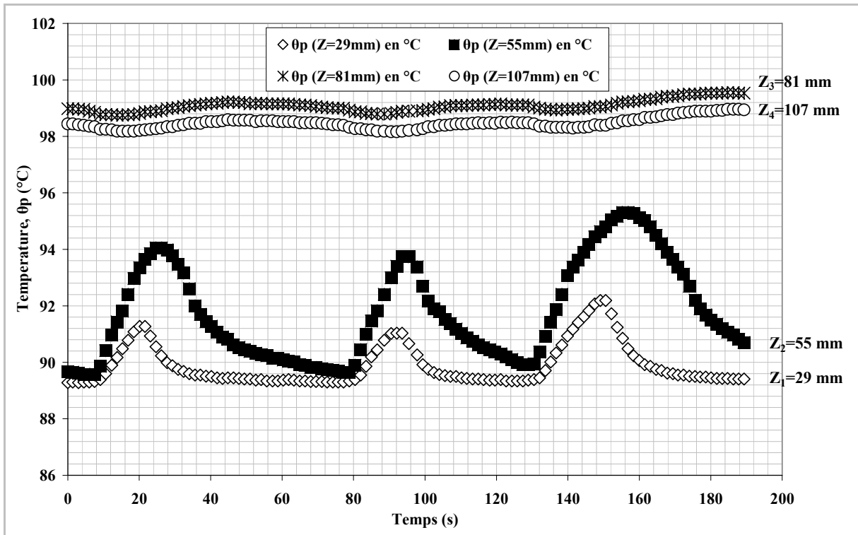
Figure III. 7 : Température de la plaque en fonction du temps à Z=29 mm, Z=55 mm et Z=107 mm - q_{elec}= 3494 W/m 2 , A=1,52 g/min, éthanol pur. Plaque n° 3 : W_C/d_C=5 , D_h=0,33 mm
