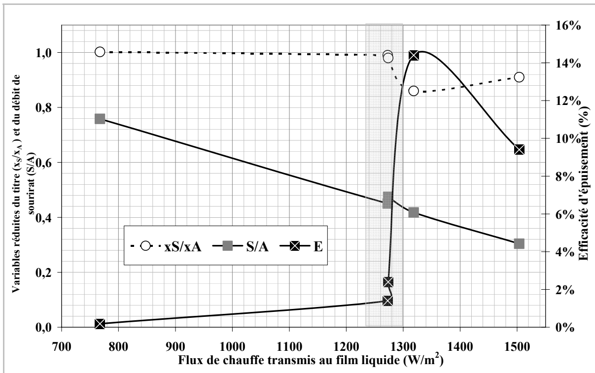
Figure IV. 6: Variables réduites en titre du soutirat ( x_S/x_A ) et en débit de soutirat ( S/A ) et l'efficacité d'épuisement ( E ) en fonction du flux de chauffe transmis au film tombant.
