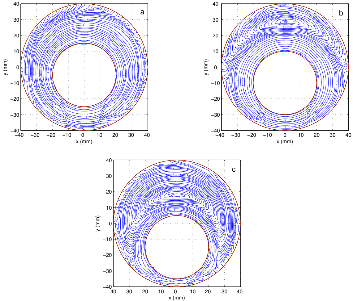
FIG. 7.19: Mesures expérimentales : Lignes de courant pour le CMC 3%, dans des géométries de trois excentricités : a) \delta = 0.25 , b) \delta = 0.5 et c) \delta = 0.75 pour \Omega = 5\text{rad/s}
