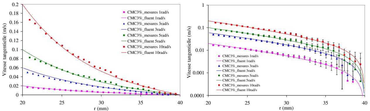
FIG. 7.4: Profils de vitesse obtenus par la mesure (PIV) et par les simulations numériques sur le CMC 3% pour des vitesses de rotation du cylindre intérieur \Omega = 1, 3, 5, \text{ et } 10 \text{ rad/s} .
