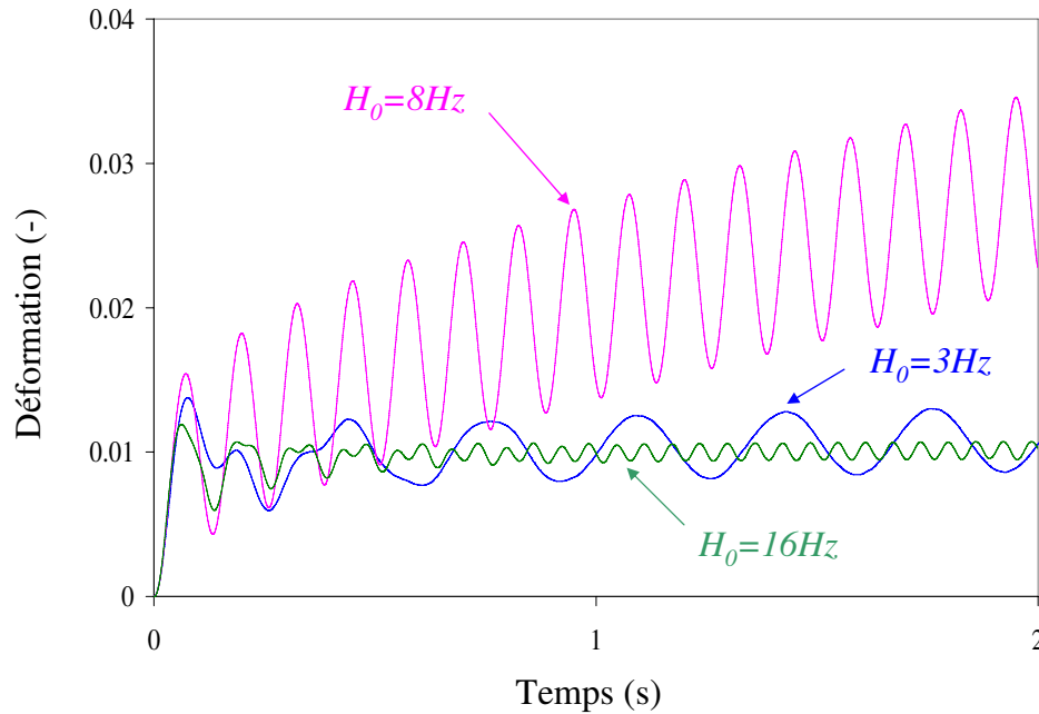
FIG. 3.10: Réponse en déformation à une contrainte oscillante autour de 0.3\text{Pa} pour les fréquences de 3, 8 et 16\text{Hz}
