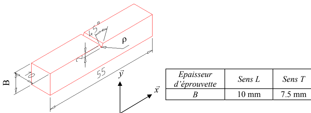
Figure IV-11 : Caractéristiques géométriques des éprouvettes.
