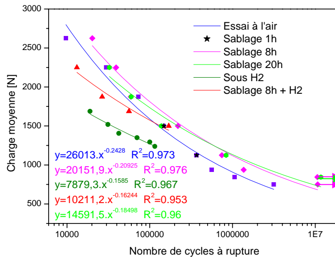
Figure III-18 : Courbes de Wöhler pour l'acier API 5L X52.
