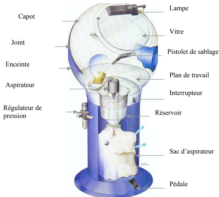
Figure II-8 : Schéma de la sableuse Blaster 2700.
