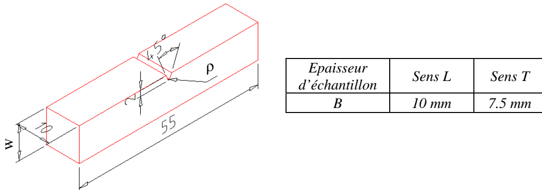
Figure III-8 : Géométrie de l'éprouvette Charpy.
