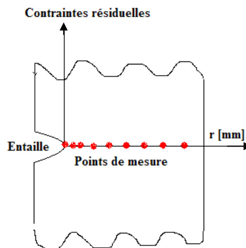
Figure IV-12 : Schéma des points des mesures.
