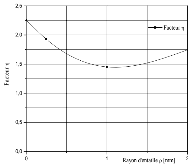
Figure I-42 : Evolution du coefficient \eta avec le rayon d'entaille (cas d'une éprouvette Charpy V) [83-84].
