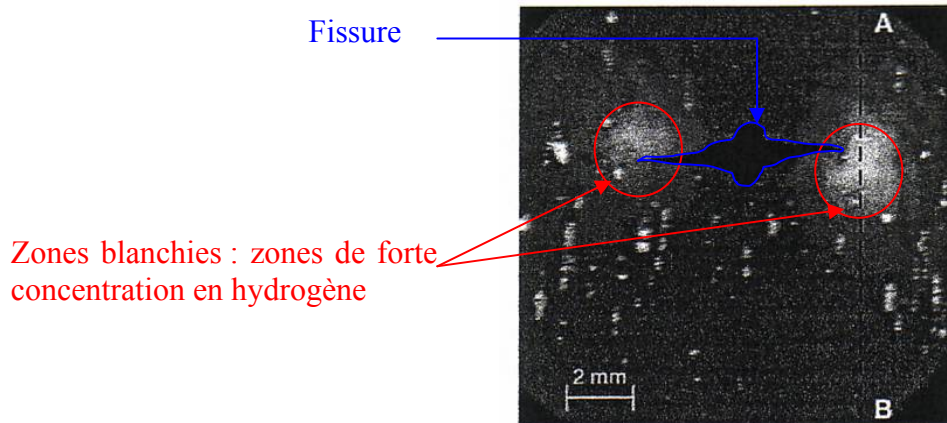
Figure I-56 : Image obtenue par microscopie photoélectrochimique de la zone proche d'une fissure (acier X46 chargé en H 2 ) [93, 112].
