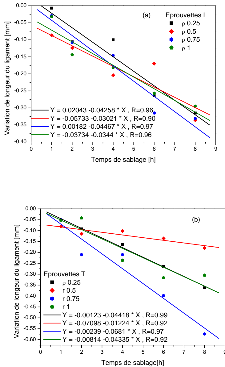
Figure II-31 : Variation de longueur du ligament pendant le sablage dans les deux sens : a) Sens L, b) Sens T.
