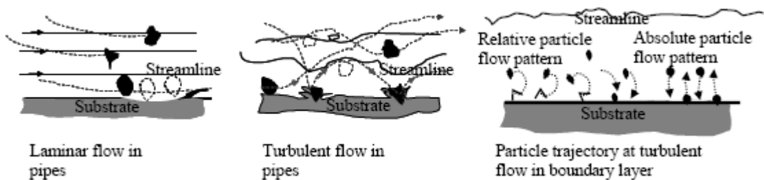
Figure I-12 : Effet des conditions du flux sur l'érosion.
