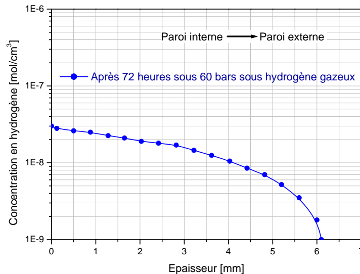
Figure II-43 : Evolution de la concentration en hydrogène dans l'épaisseur du tuyau.
