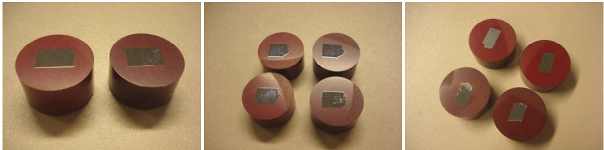
Figure IV-21 : Echantillons de microdureté HV préparés à partir des éprouvettes de : a) fatigue, b) Charpy L, c) Charpy T.
