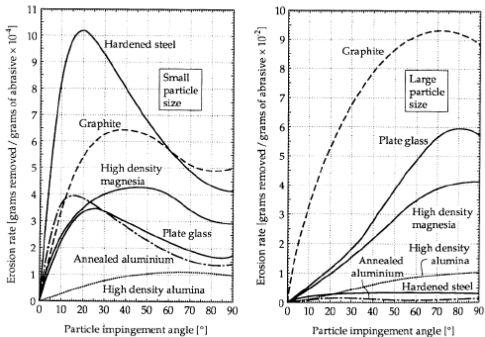
Figure I-13 : Classement de la résistance à l'érosion. Le sable utilisé est le silicium carbide à une vitesse de 152 m/s [10,31].
