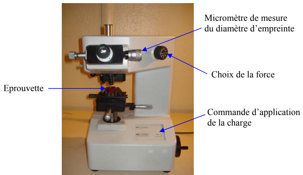
Figure IV-22 : Microduromètre Vickers.
