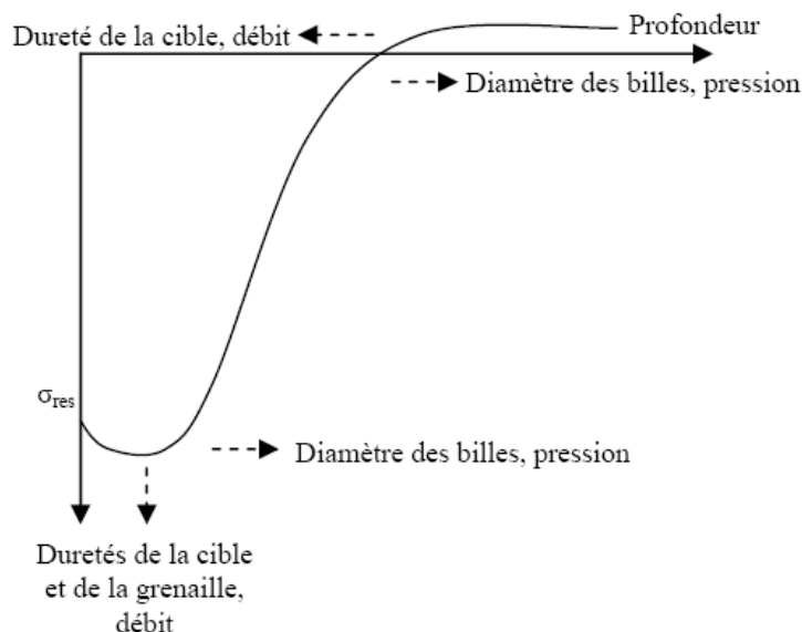
Figure I-34 : Représentation schématique des effets des différents paramètres du processus du grenailage [61].
