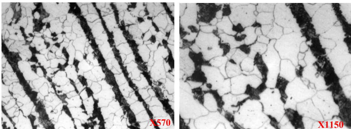
Figure II-3 : Microstructure de l'acier API 5L X52, analyse longitudinale, avec un grossissement de X570 et de X1150.
