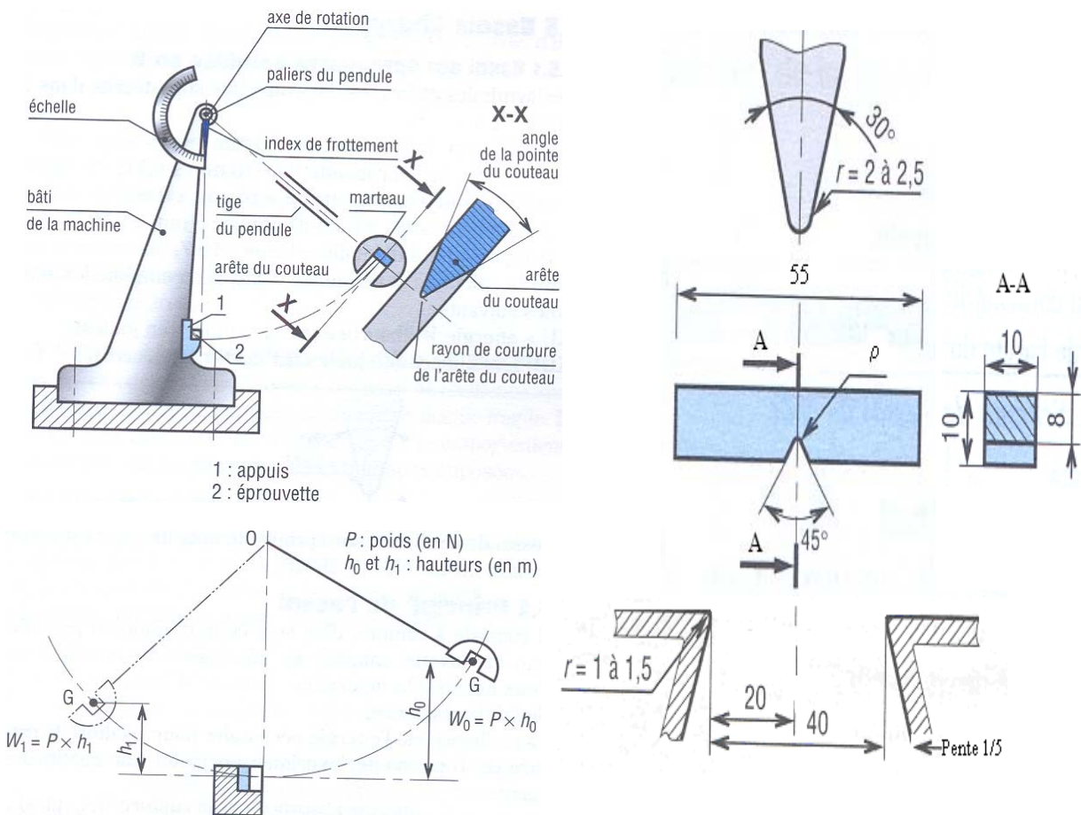
Figure III-7 : Description du mouton-pendule Charpy et du positionnement de l'éprouvette [7].
