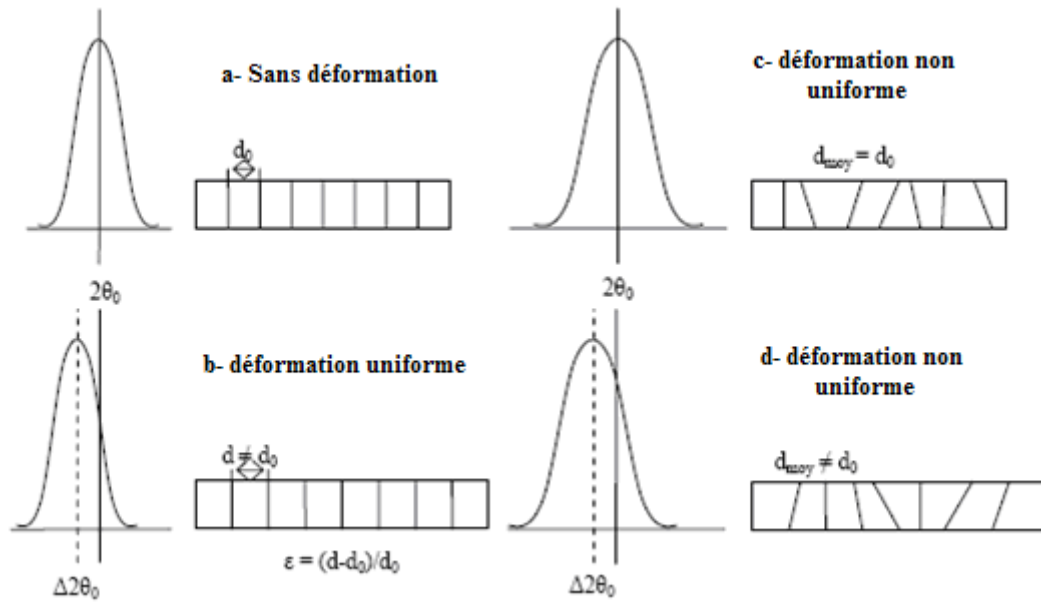
Figure IV-9 : Illustration de l'effet de distorsion sur les pics de diffraction [7].
