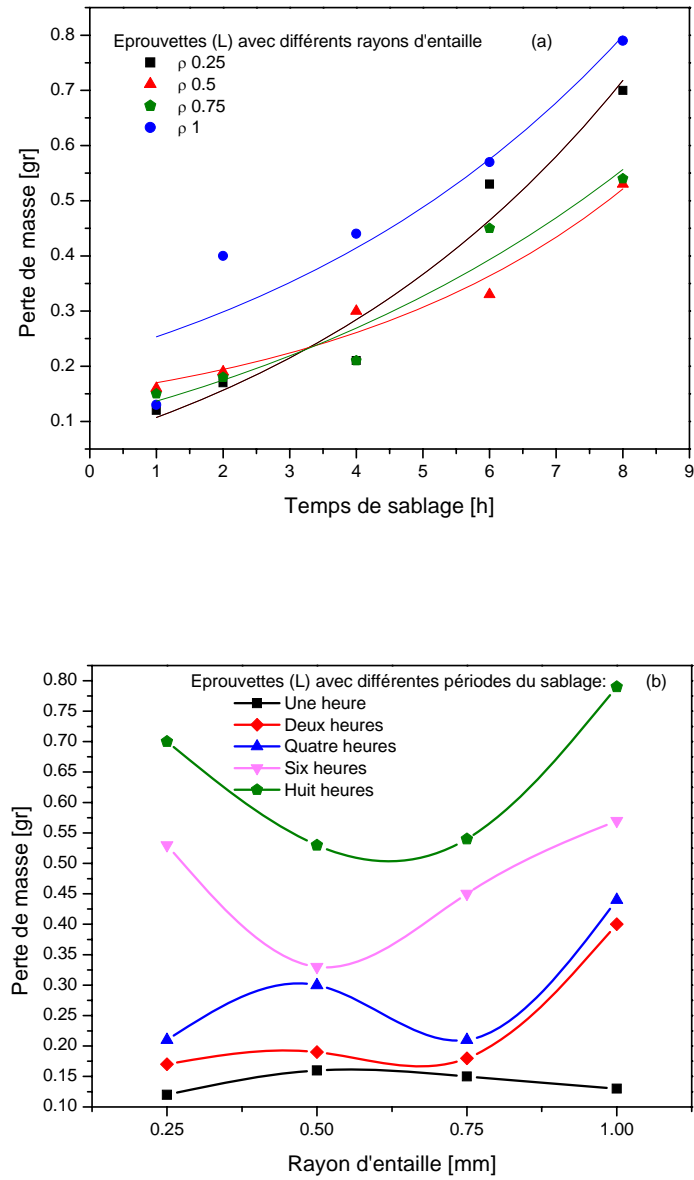
Figure II-18 : Evaluation de la perte de masse dans le sens longitudinal en fonction de : a) Temps de sablage, b) Rayons d'entaille.
