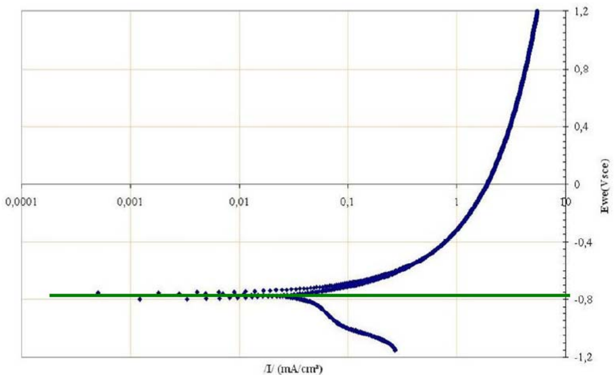
Figure II-34 : Courbe de polarisation de l'acier API 5L X52.
