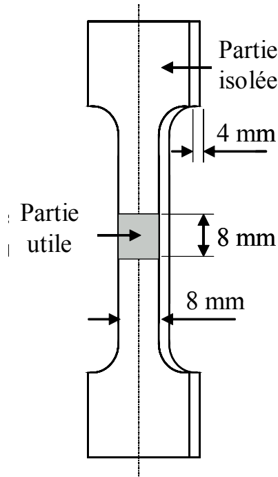
Figure II-37 : Eprouvette de chargement/déchargement en hydrogène.
