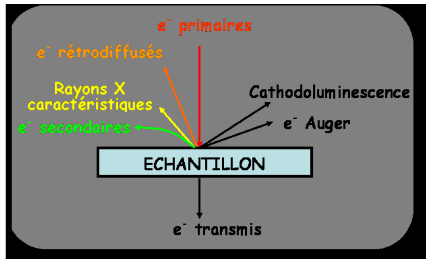
Figure IV-4 : Signaux produits par interaction d'un électron primaire avec l'échantillon.
