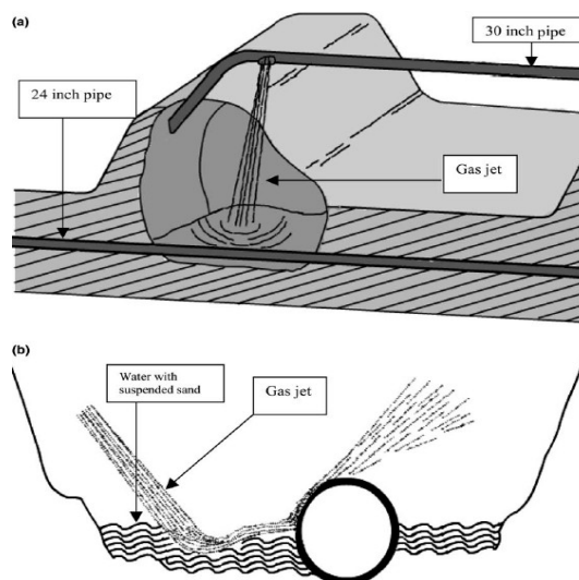
Figure I-22 : Mécanisme d'érosion du tuyau A (610 mm) [52].
