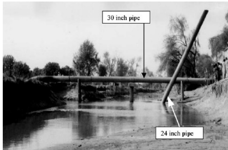
Figure I-21 : Photographie du site de la rupture.
