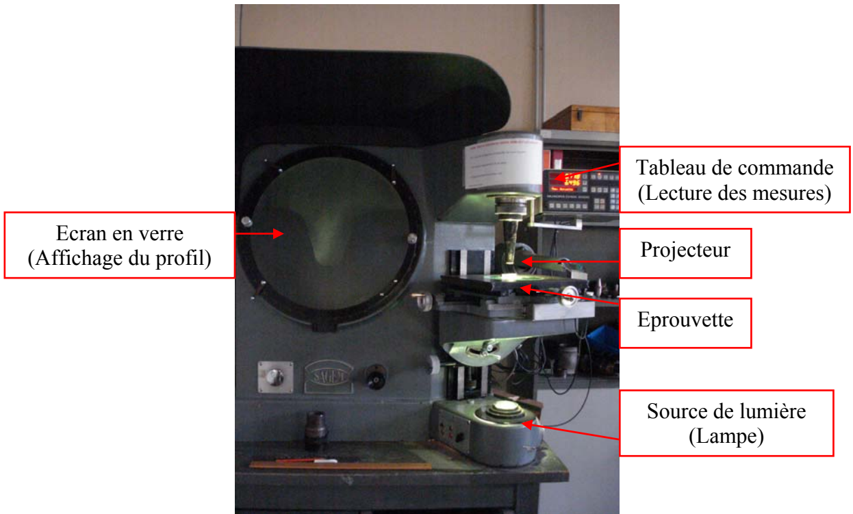
Figure II-26 : Machine de mesure du profil d'entaille.
