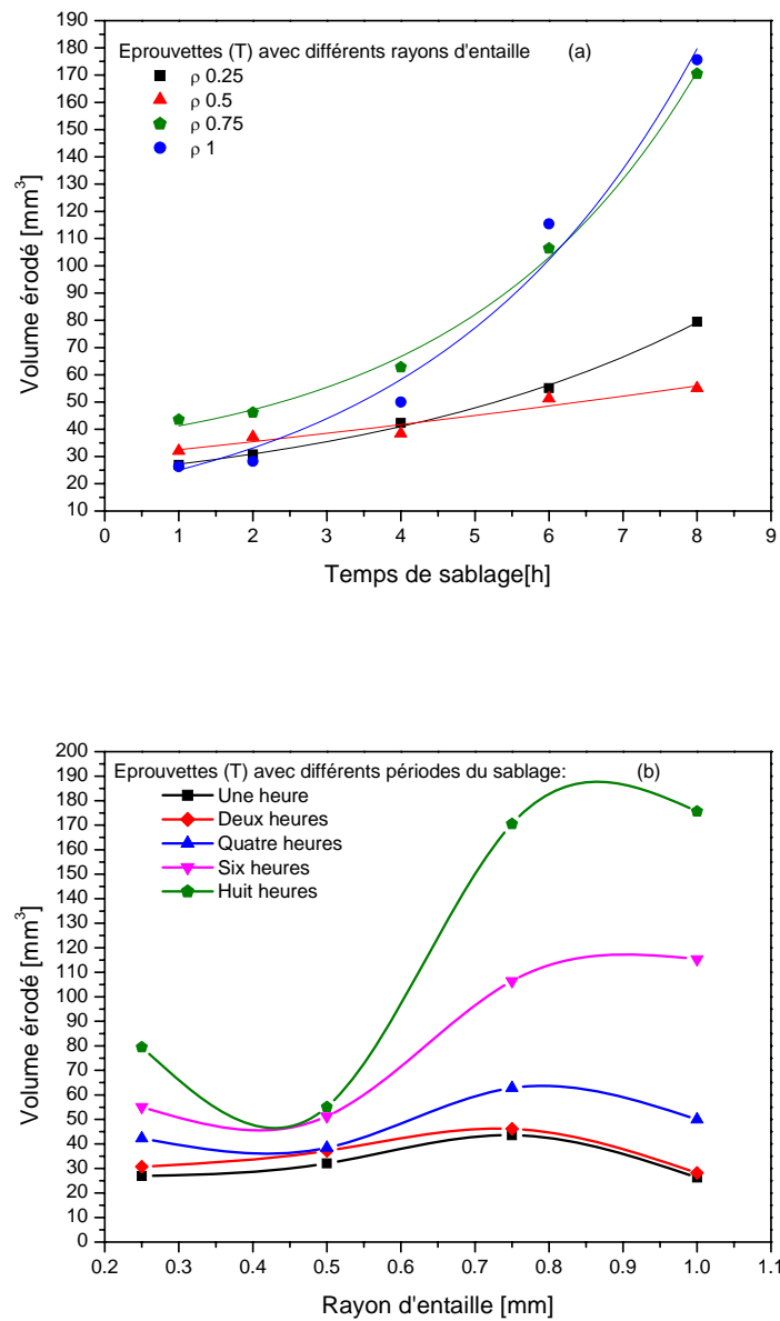
Figure II-21 : Evaluation du volume érodé dans le sens transversal en fonction de : a) Temps de sablage, b) Rayons d'entaille.
