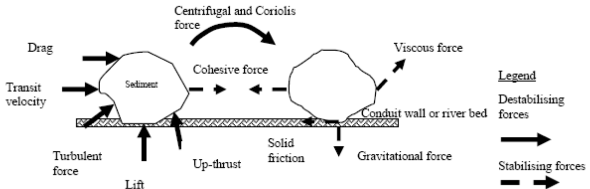
Figure I-16 : Forces agissantes sur les particules dans le champ d'écoulement [38].
