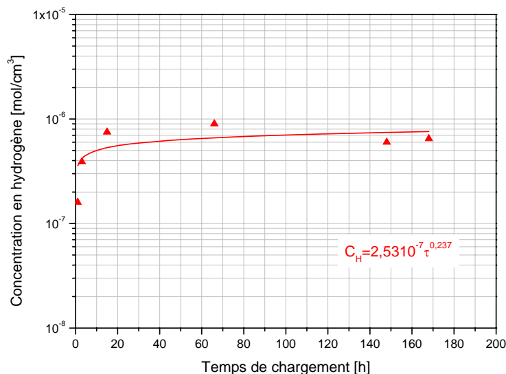
Figure II-41 : Evolution de la concentration en hydrogène en fonction du temps de chargement.
