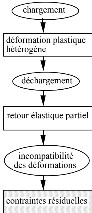
Figure IV-7 : Schéma d'introduction des contraintes résiduelles par déformation plastique.
