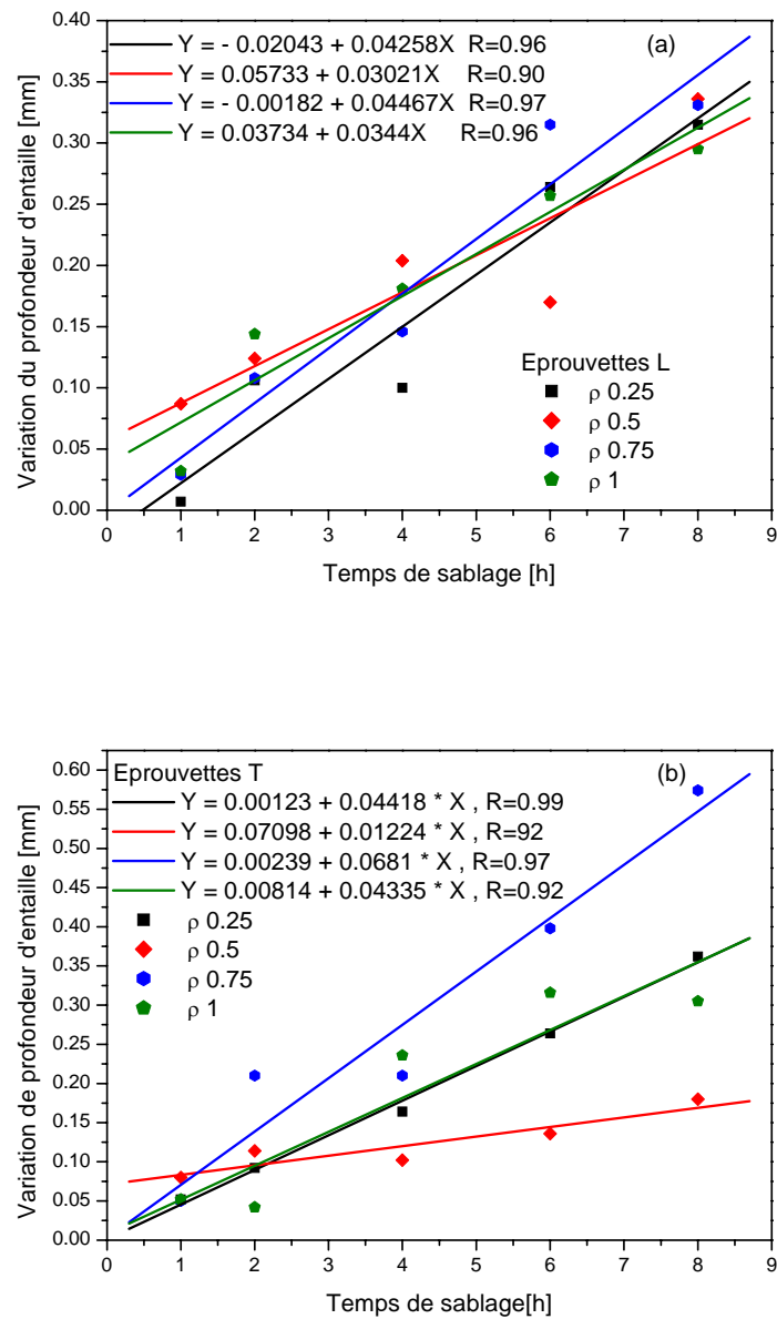
Figure II-30 : Variation de profondeur d'entaille pendant le sablage dans les deux sens : a) Sens L, b) Sens T.
