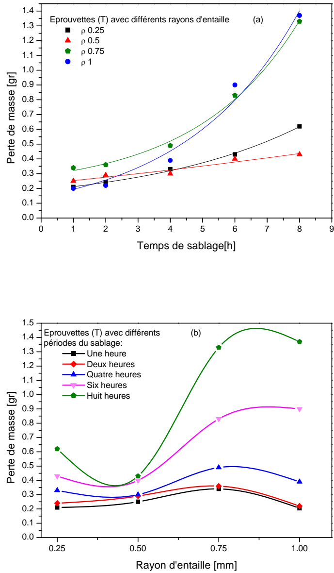
Figure II-19 : Evaluation de la perte de masse dans le sens transversal en fonction de : a) Temps de sablage, b) Rayons d'entaille.
