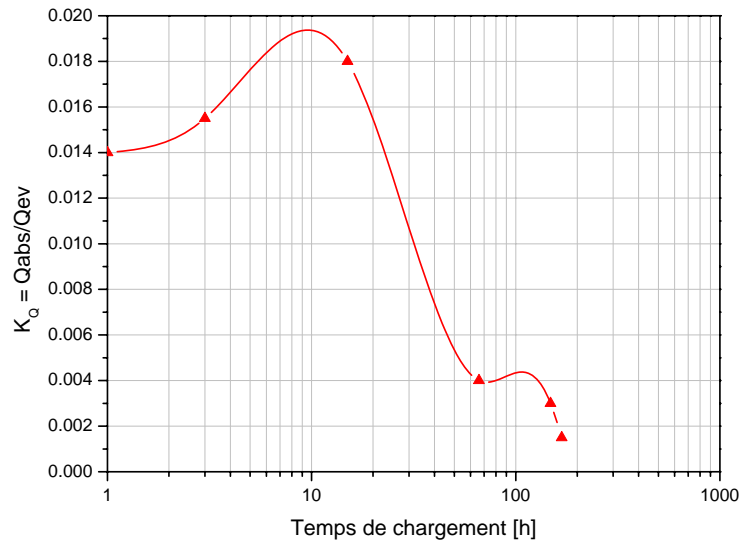
Figure II-42 : Efficacité du chargement de l'acier API 5L X52.
