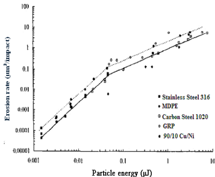
Figure I-9 : Erosion en fonction de l'énergie des particules affectées sur une surface de tuyau, pour un angle de 90° [27].
