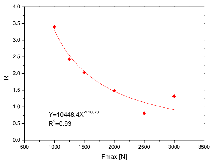
Figure III-19 : Variation du gain en durée de vie en fonction de la charge maximale appliquée.
