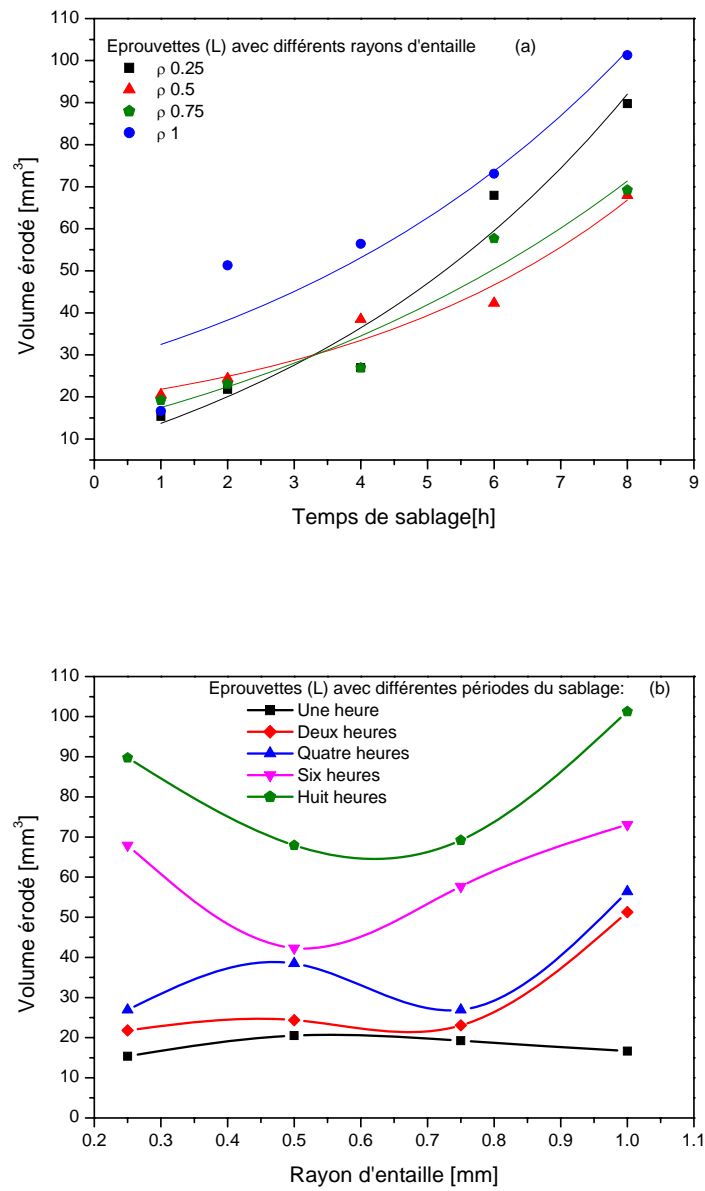
Figure II-20 : Evaluation du volume érodé dans le sens longitudinal en fonction de : a) Temps de sablage, b) Rayons d'entaille.
