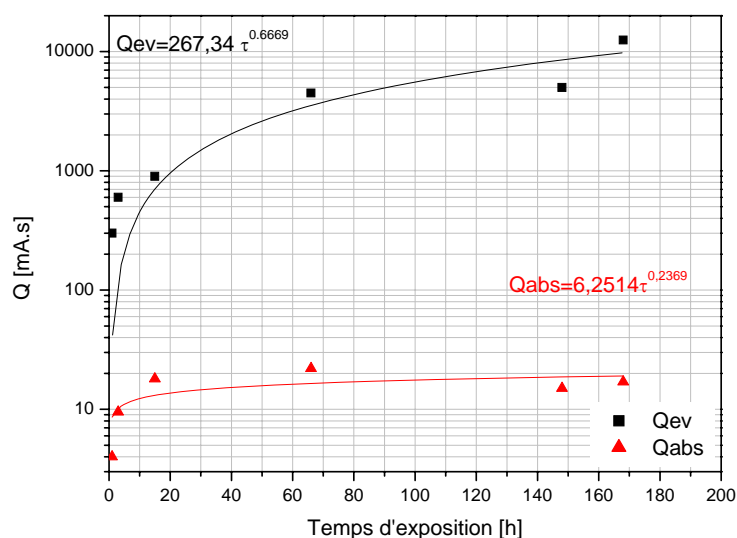
Figure II-40 : Quantité d'hydrogène créée et absorbée par l'acier API 5L X52.
