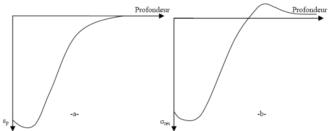
Figure I-33 : Représentation schématique : a) Profil de déformation plastique et b) Distribution de contraintes résiduelles associées en profondeur [57].
