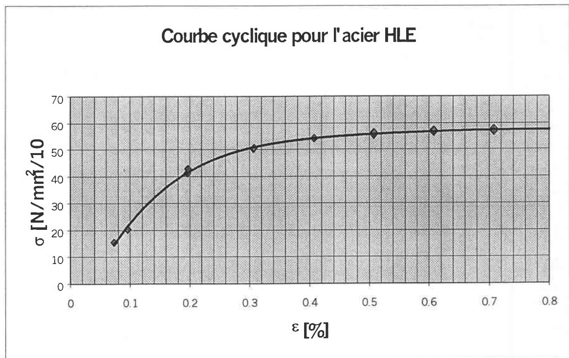
Fig. 10.10 : Risultati delle prove oligocicliche per l'acciaio HLE.
