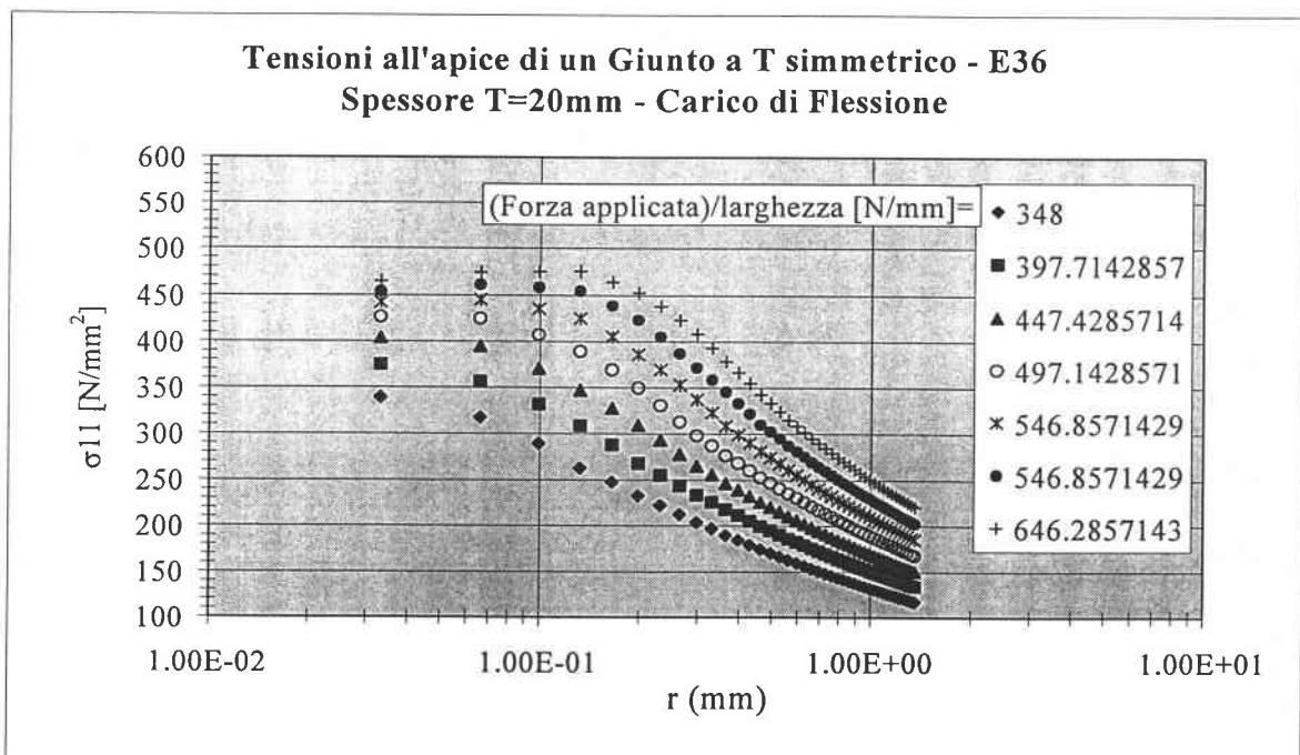
Fig. 12.1 : Andamento della prima tensione principale all'apice dell'intaglio.
