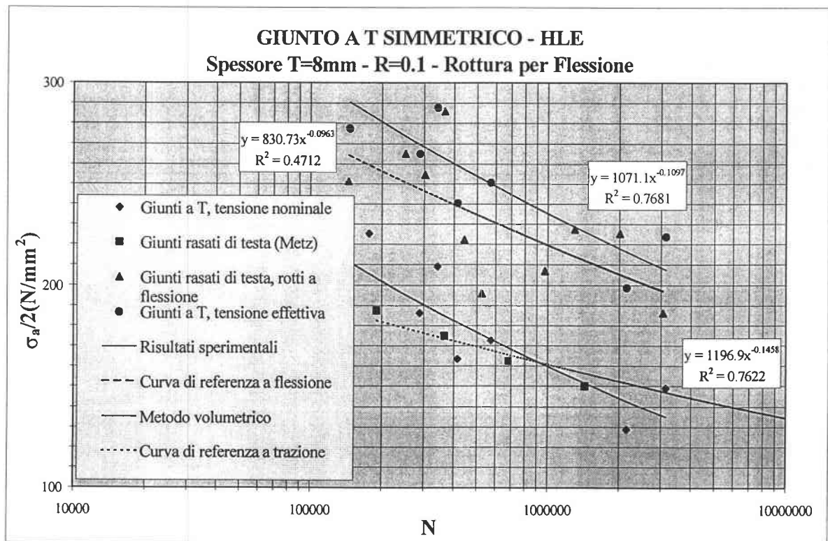
Fig. 12.6 : Risultati sull'applicazione del Metodo volumetrico per giunti a T da 8 mm in HLE
