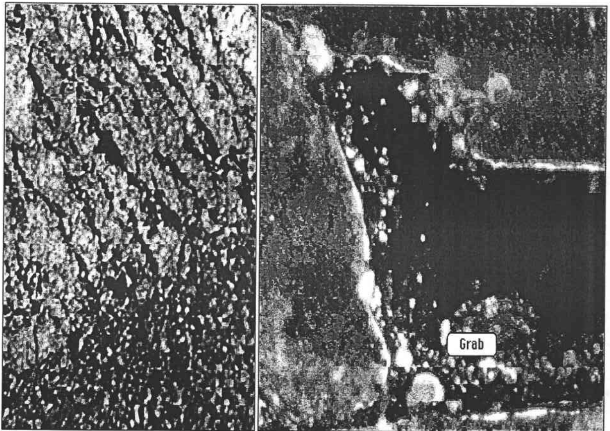
Foto. 11.3 : HAZ e Materiale base.
