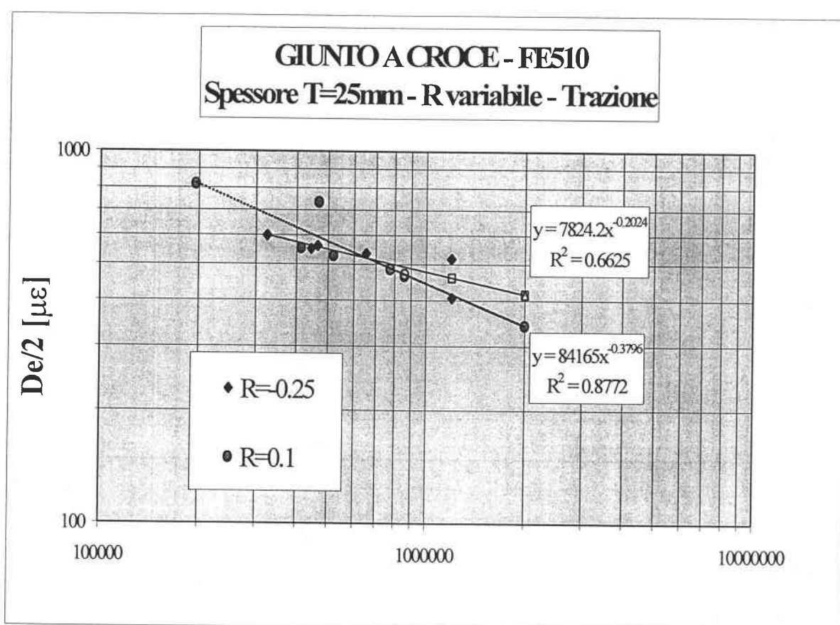
Fig. 13.6 : Applicazione del Metodo a giunti a croce da 25 mm.
