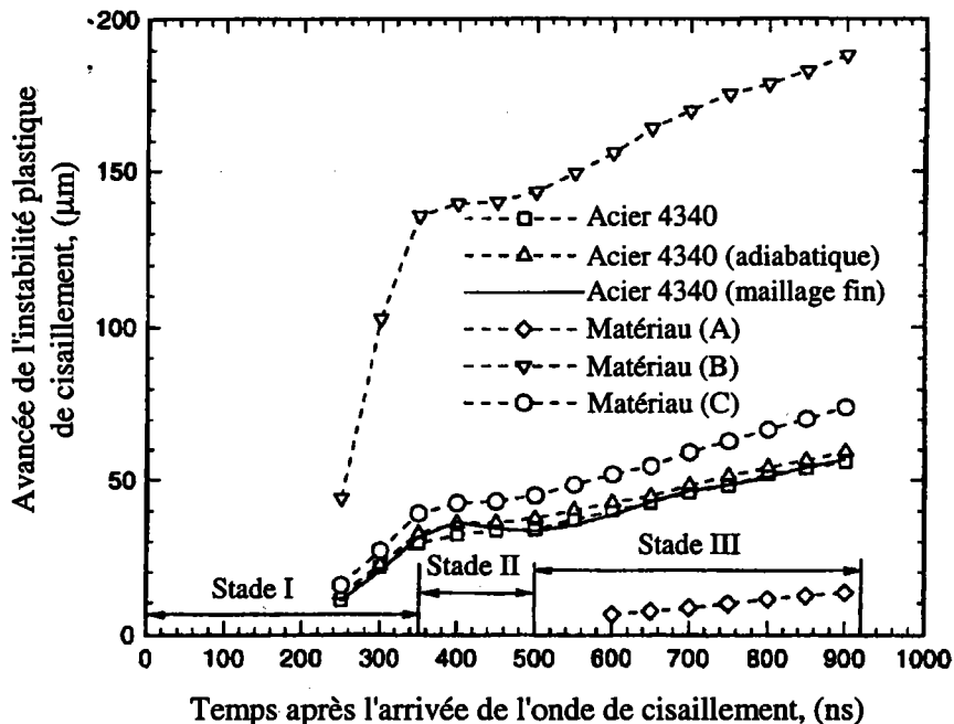
Figure 1.18. Evolution de l'avancée de l'instabilité plastique, en fonction du temps après l'arrivée, de l'onde de cisaillement pour différentes configurations. Trois régimes sont visualisables dans chacun des cas. D'après Lee et Prakash (1998).
