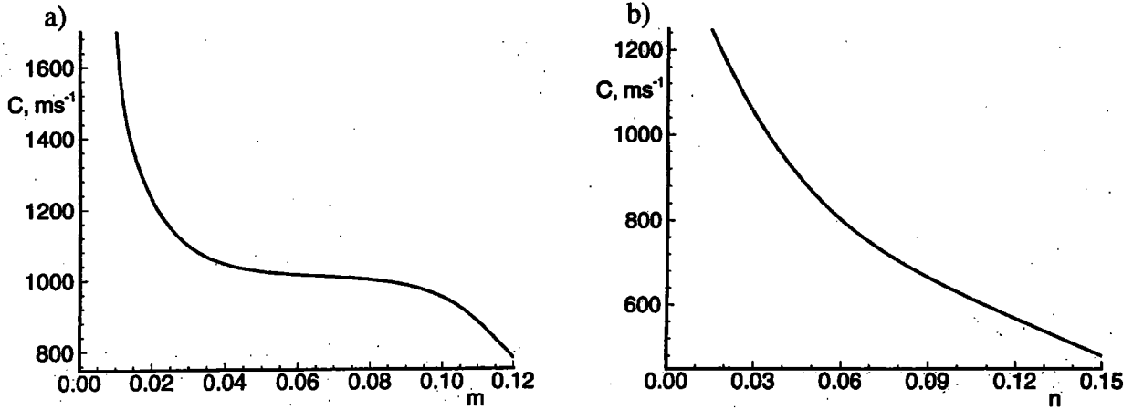
Figure 4.18. Effet stabilisant a) de la sensibilité à la vitesse de déformation m , b) de l'écroutissage n , sur la célérité C . La vitesse appliquée est V=2\text{m/s} . D'après Mercier et Molinari (1998).
