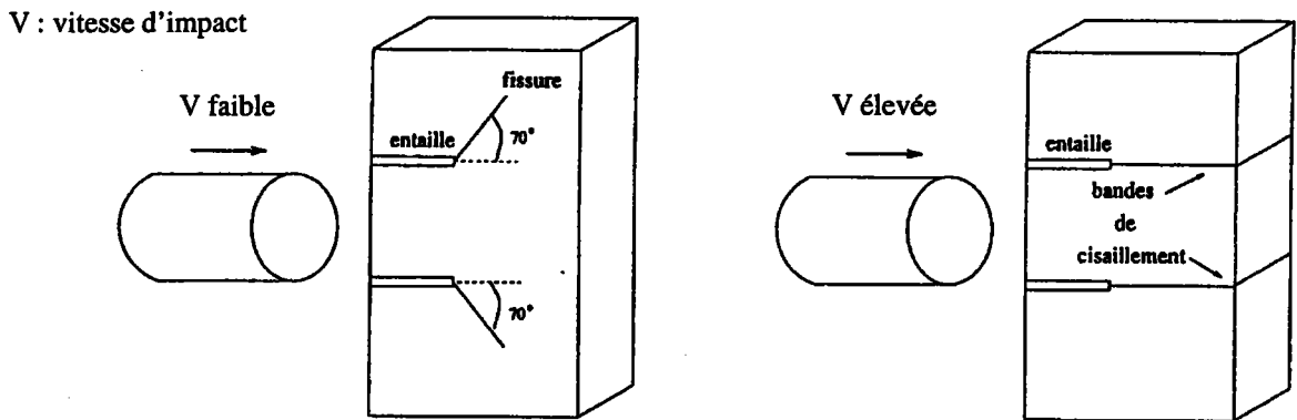
Figure 1.3. Schéma de principe du dispositif expérimental développé par Kalthoff et Wrinkler (1987).
