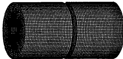
Figure 1.15. Représentation discrétisée de l'éprouvette cylindrique à paroi épaisse utilisée par Batra et Ratazzi (1997). Une entaille en V est introduite pour faciliter l'apparition d'une bande de cisaillement adiabatique.
