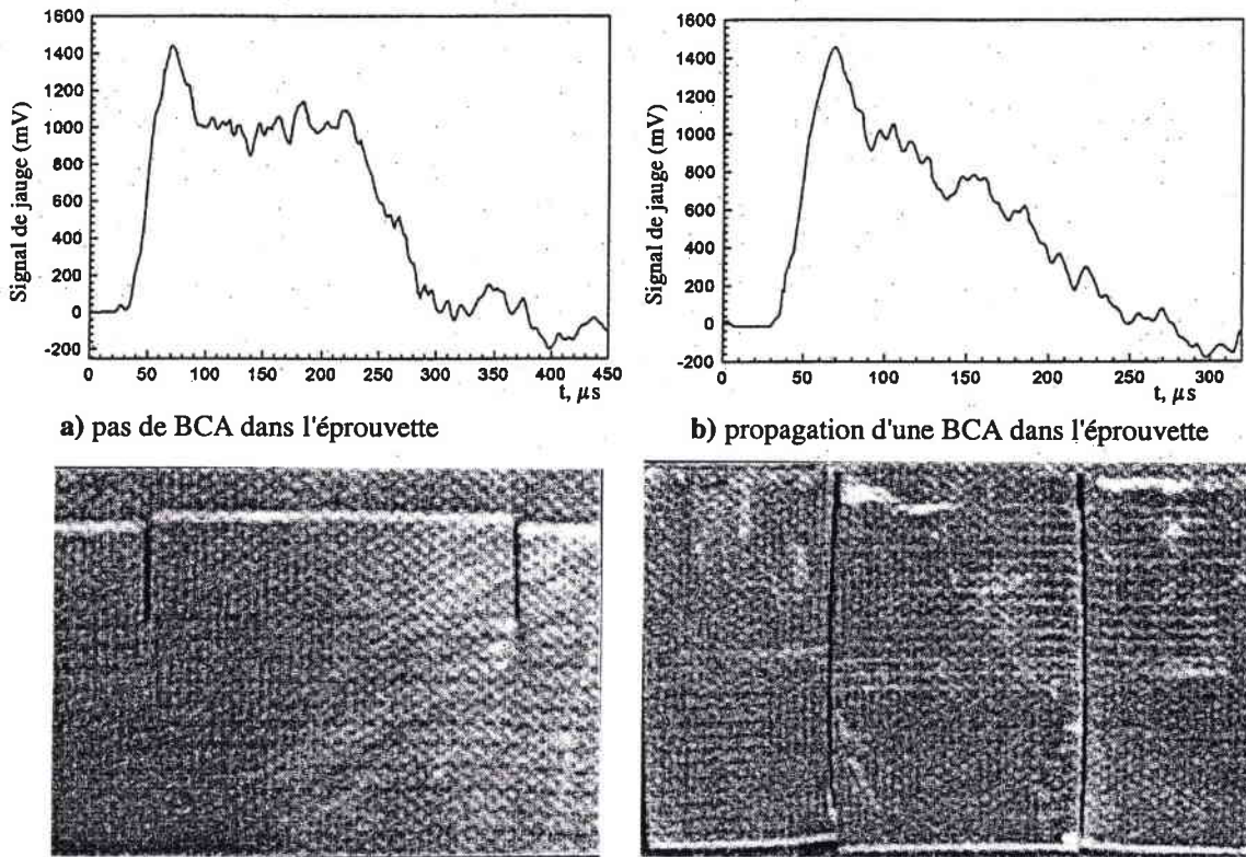
Figure 1.8. Représentation des signaux de jauge recueillis
