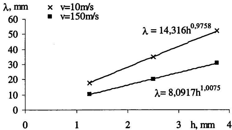
Figure 4.24. Evolution de la taille caractéristique de la zone de transition en fonction de la hauteur de l'éprouvette. Deux vitesses distinctes sont étudiées V=10\text{m/s} et V=150\text{m/s} .
