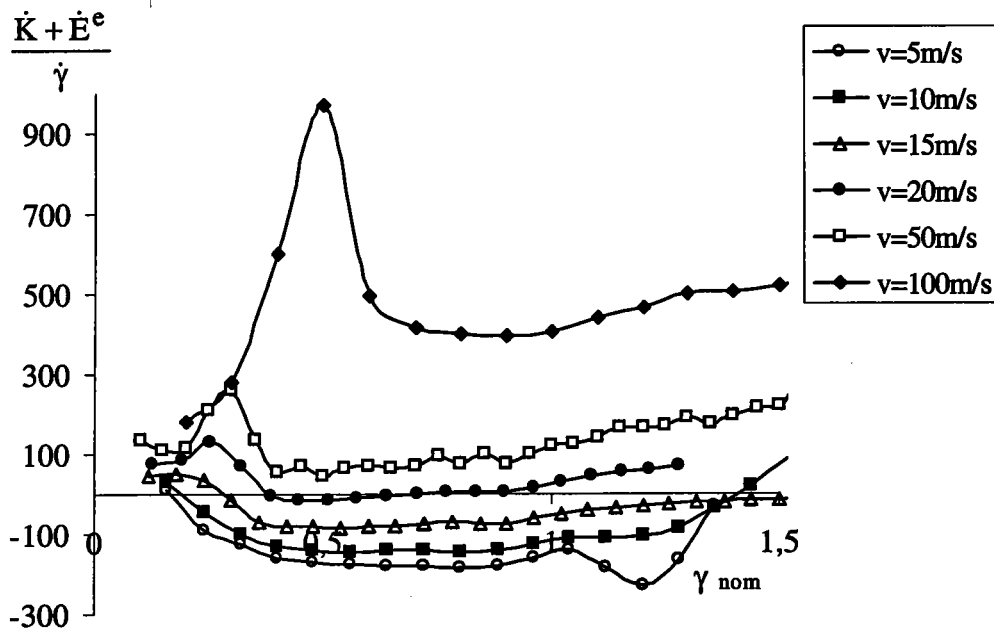
Figure 3.23. Evolution de (\dot{K} + \dot{E}^e) / \dot{\gamma} en fonction de \gamma_{nom} pour différentes valeurs de vitesse appliquée. La vitesse V=20\text{m/s} engendre une évolution quasi-nulle de (\dot{K} + \dot{E}^e) / \dot{\gamma} en fonction du cisaillement nominal. La loi de comportement A est considérée.
