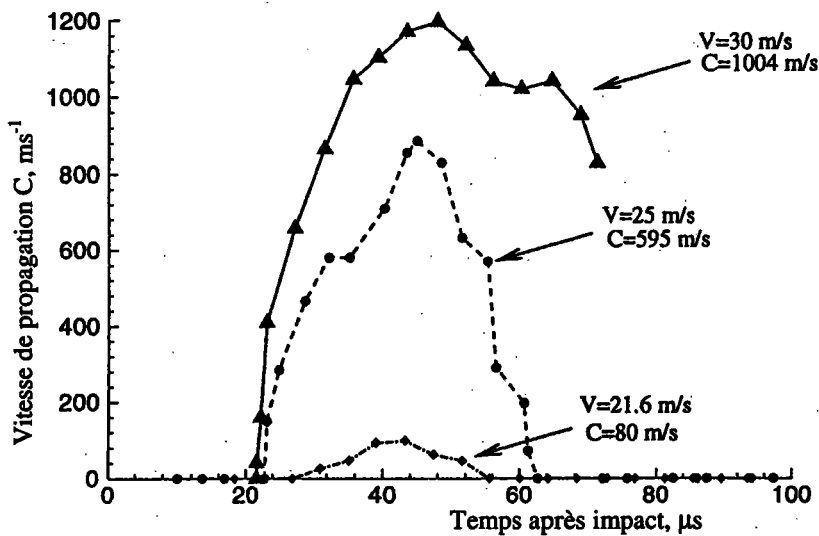
Figure 1.5. Evolution au cours du temps de la célérité de propagation de la bande pour l'acier C300. Différentes vitesses d'impact sont considérées. D'après Zhou et al. (1996a).
