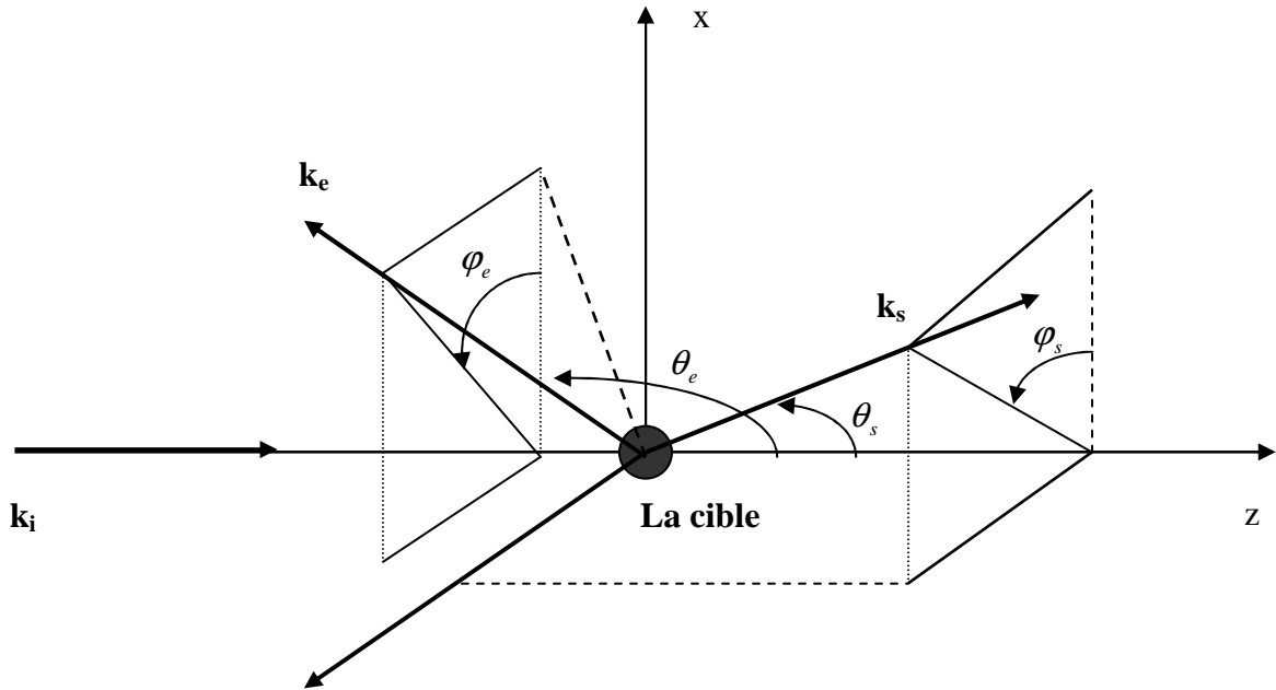
Figure 1.1 : Schéma de la collision (e,2e)
