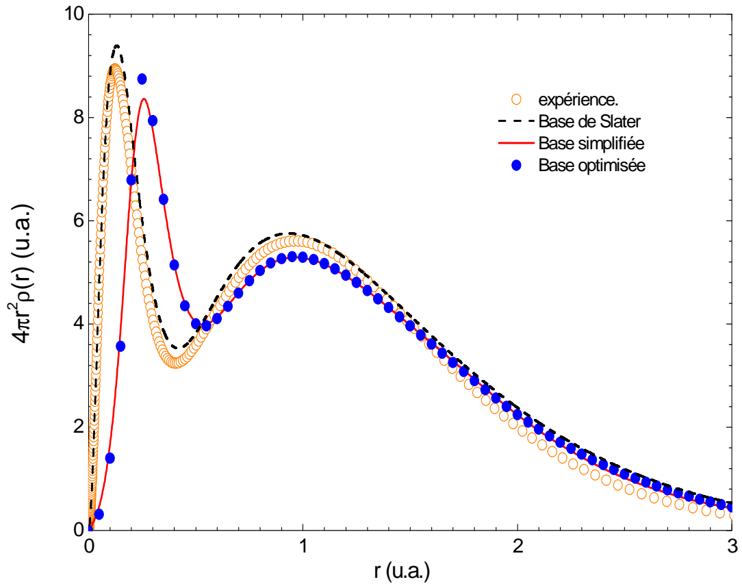
Figure 4.1 : Distributions électroniques de charges pour la molécule H_2O obtenues dans les différentes bases étudiées : base de fonctions de type Slater proposée par Moccia (courbe pointillée), base gaussienne de type 6-31G (courbe en étoile) et base gaussienne de type aug-cc-pVQZ (Courbe continue). Les données expérimentales reportées correspondent aux expériences de Ellison et al., et Banyard et al. [30-31].
