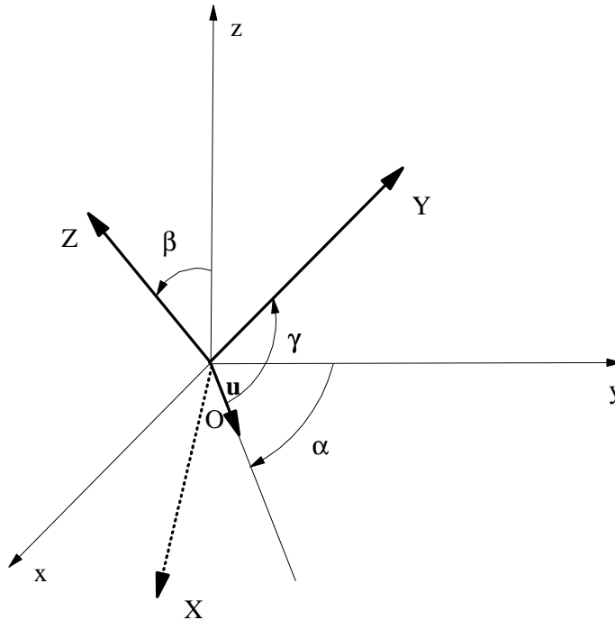
Figure 3.1 : Représentation de la rotation \mathfrak{R}_o(\alpha, \beta, \gamma) de centre O caractérisée par les angles d'Euler (\alpha, \beta, \gamma) . Le trièdre (O, X, Y, Z) est l'image du trièdre (O, x, y, z) par cette rotation.
