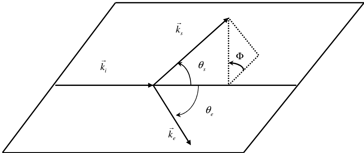
Figure 4.2 : Géométrie symétrique non coplanaire
