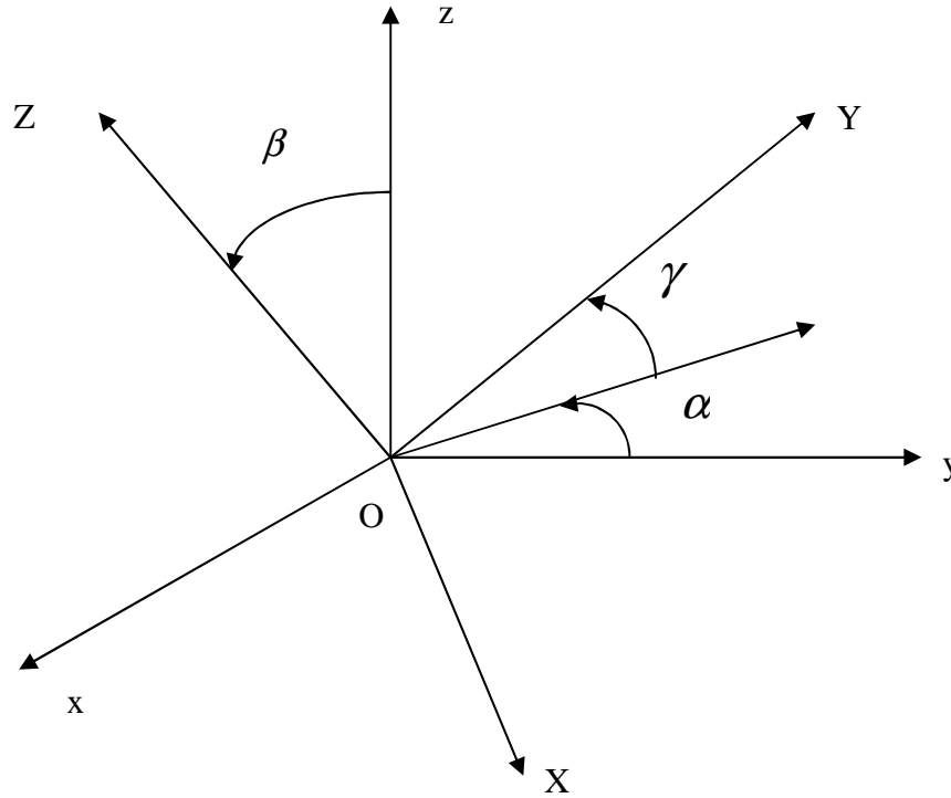
Figure 1.2 : Angles d'Euler permettant le passage du repère lié à la molécule (Oxyz) vers le repère du laboratoire OXYZ
