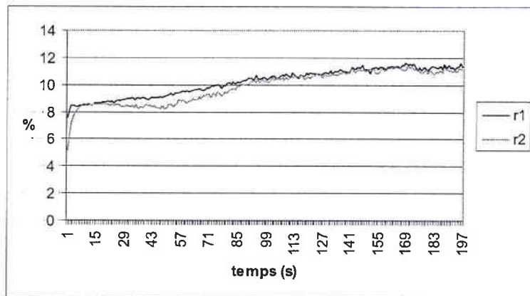
FIG. 5.23 – Evolution temporelle des rendements du DPCM dans le cristal non dopé avec deux faisceaux fins pour h = 60 \mu\text{m}
