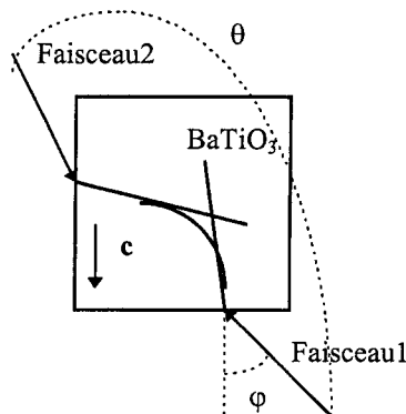
FIG. 3.11 – Modified Bridge dans BaTiO_3 présenté par Wang et al. [45]
