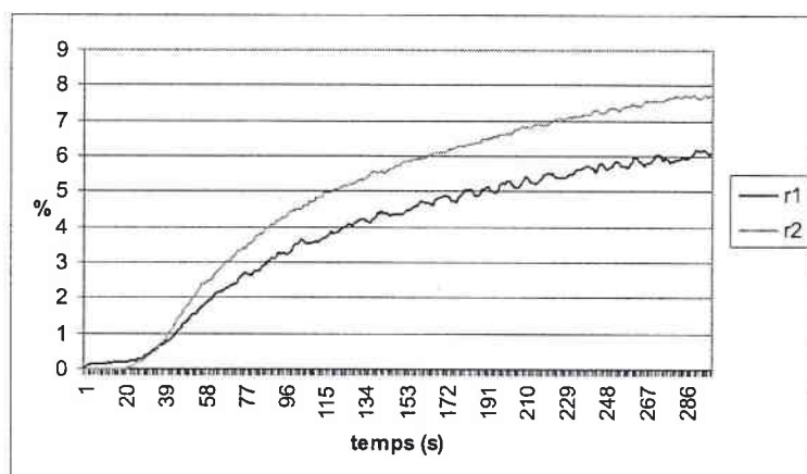
FIG. 5.76 – Evolution des rendements du DPCM dans le cristal dopé en faisceaux fins d = -327 \mu\text{m}
