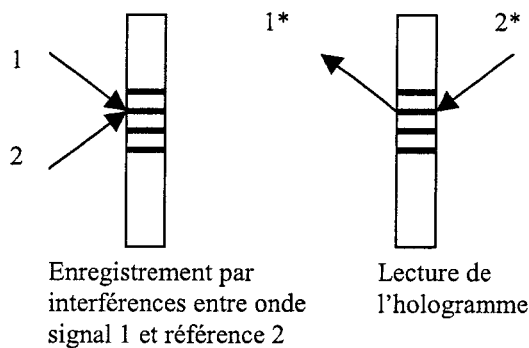
FIG. 2.3 – Inscription et lecture d'un hologramme statique
