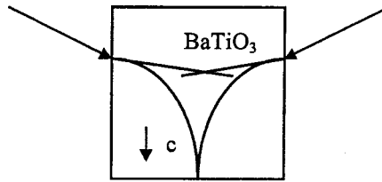
FIG. 3.4 – BWPC présenté par Ewbank [39]
