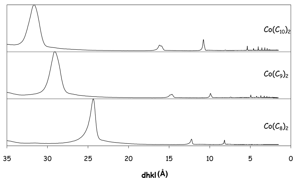
Figure 9 : diffractogrammes des carboxylates de cobalt roses du type \text{Co}(\text{C}_x)_2 pour x = 7, 8, 9 et 10
