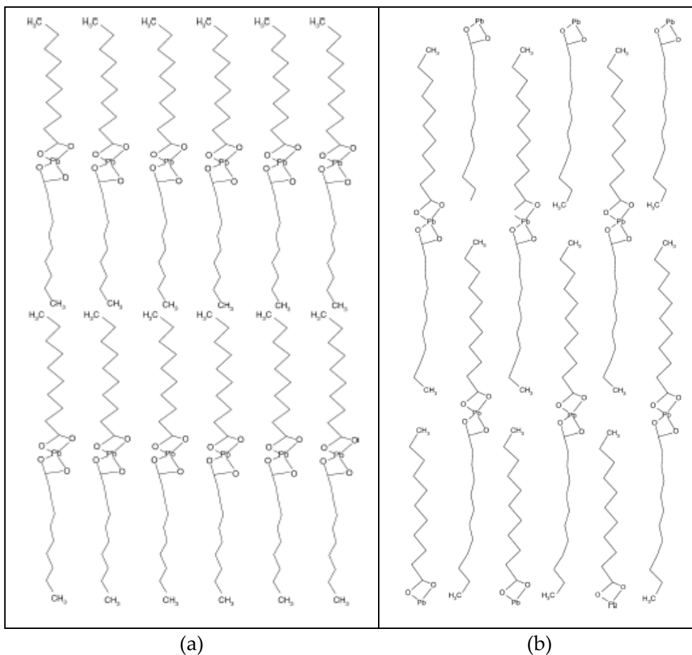
Figure 4 : représentation des empilements double couche (a) et mono couche (b) des chaînes aliphatiques dans les feuillets [Ellis, 2005]
