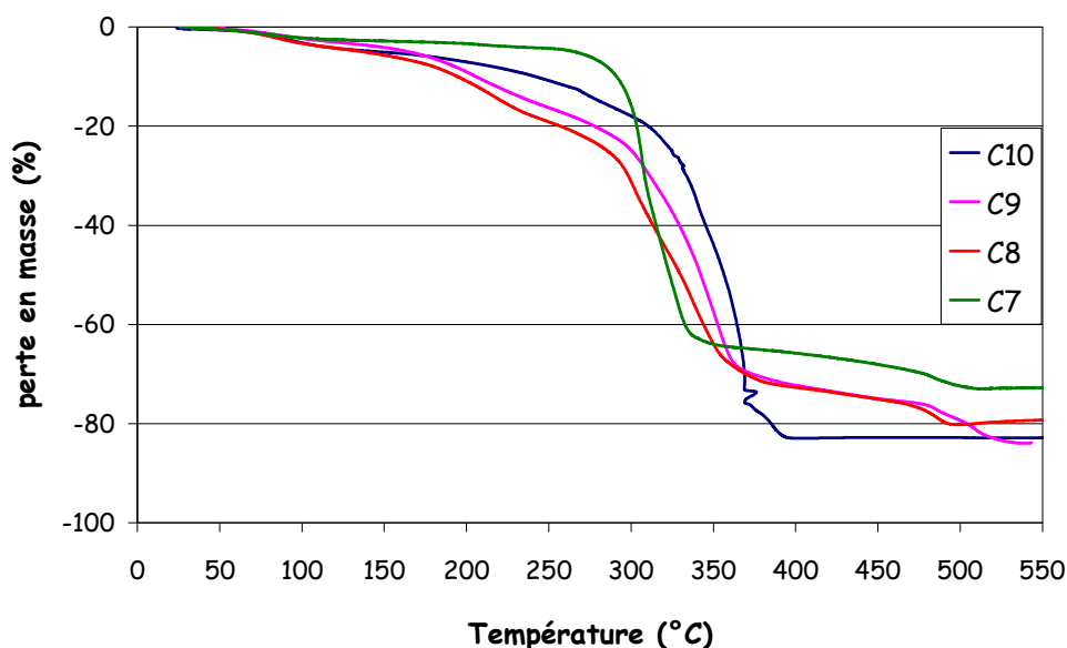
Figure 32 : thermogrammes des carboxylates de nickel du type Ni(C_x)_2 pour x = 7, 8, 9 et 10
