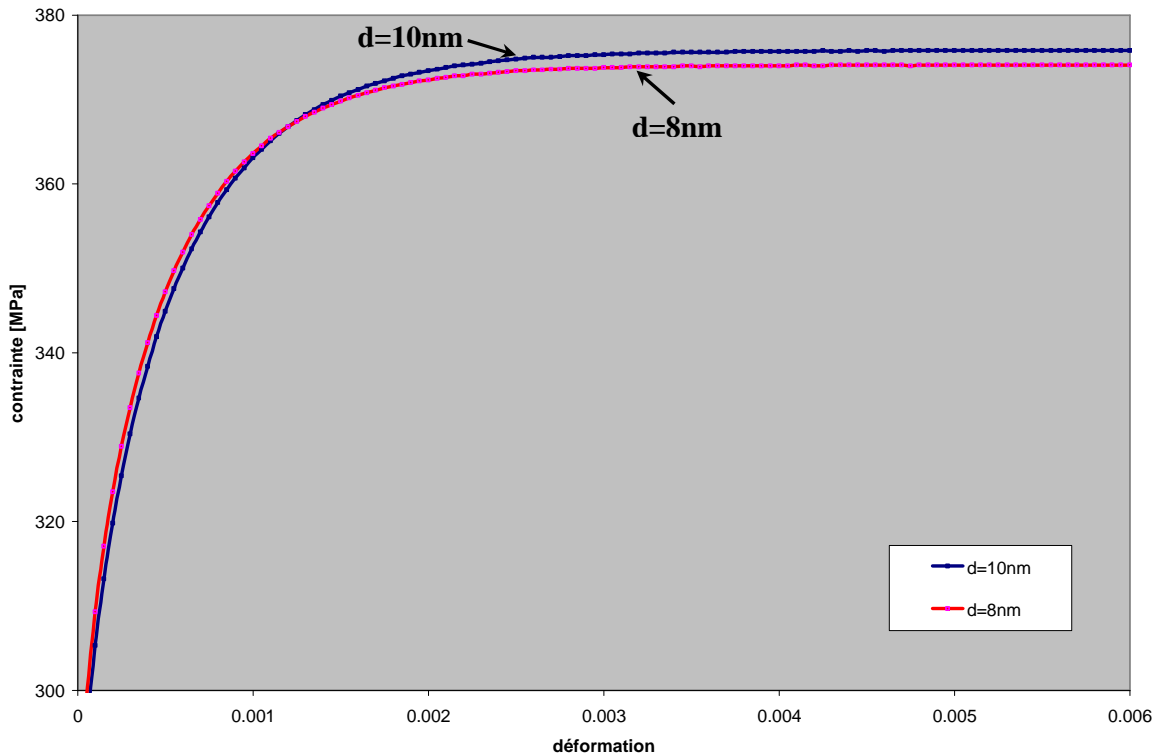
Figure VI-33 : Réponse globale à K_{cc}=2 et 1.E-3/s pour d= 10\text{ nm} et 8\text{ nm}
