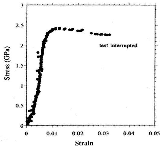
Figure II-44: Courbe de compression à la température ambiante du fer nanométrique dense, d=80 nm (Ma, 2000)
