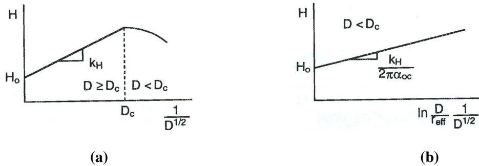
Figure III-1 : (a) courbe montrant l'inversion de la pente de Hall Petch (b) Pente de Hall Petch modifiée (Scattergood et Koch, 1992)
