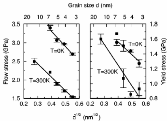
Figure II-42 : limite d'élasticité et contrainte d'écoulement en fonction de la taille des grains (Schiotz et al., 1999)
