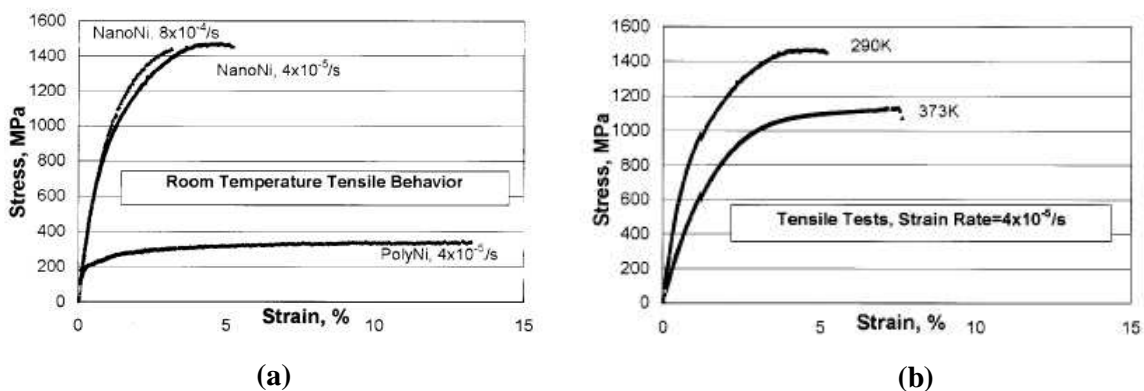
Figure II-47 : Courbe contrainte-déformation du nickel nanocristallin (a) en fonction de la vitesse de déformation et à température ambiante (b) en fonction de la température (Yin et al., 2001)
