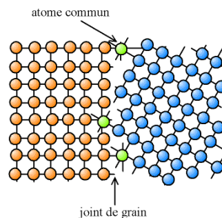
Figure II-54 : Joint de grande désorientation. Atomes communs aux deux réseaux
