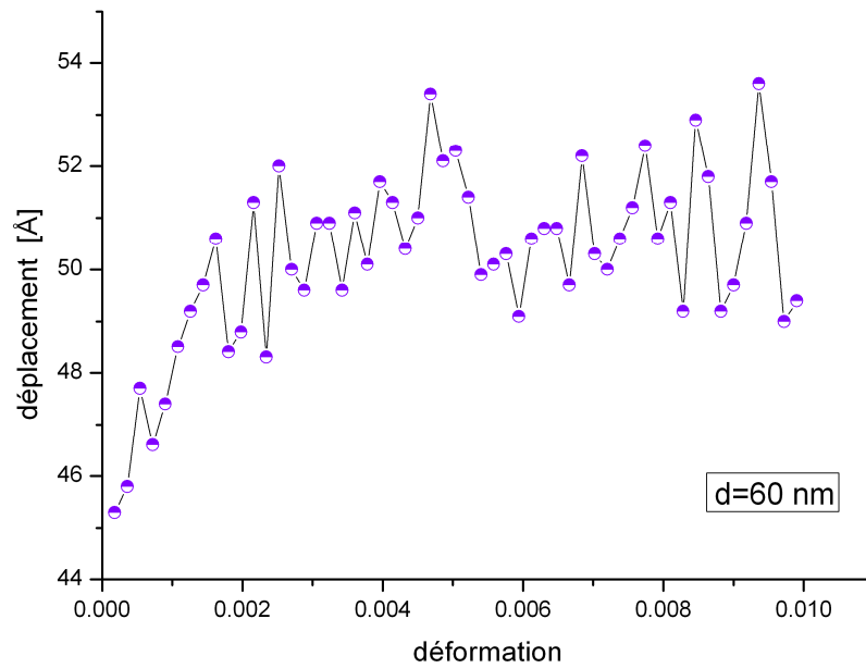
FigureVI-20 : Courbe déformation-déplacement pour d=60 nm
