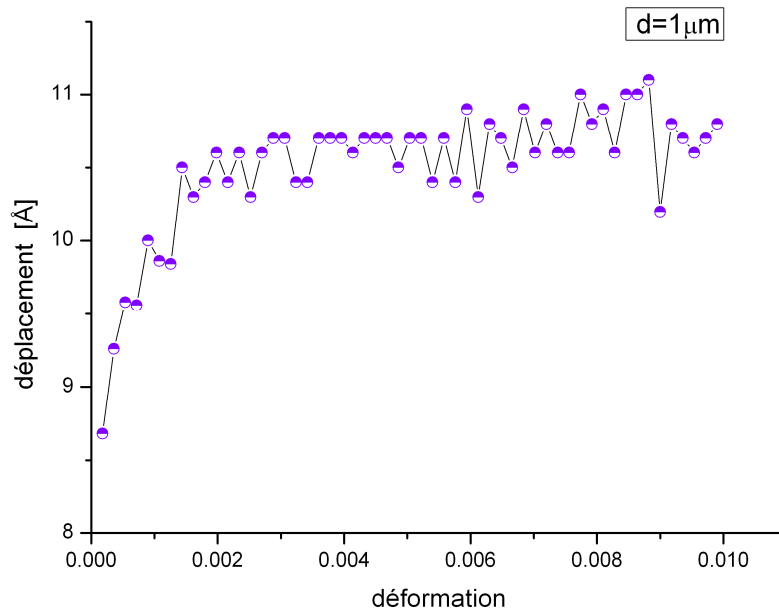
FigureVI-19 : Courbe déformation-déplacement pour d=1 μm
