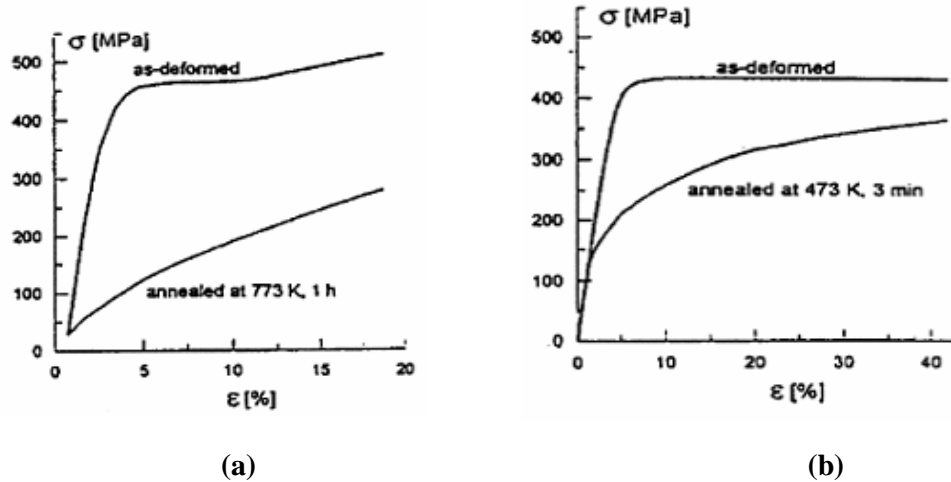
Figure II-46 : Courbes de traction du cuivre à grains ultrafins bruts recuits (a) pendant 1h à 773K, (b) pendant 3 min à 473K (Valiev et al., 2000)
