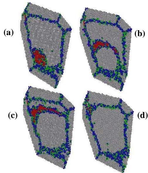
Figure V-5 : émission de dislocations par le joint de grains
