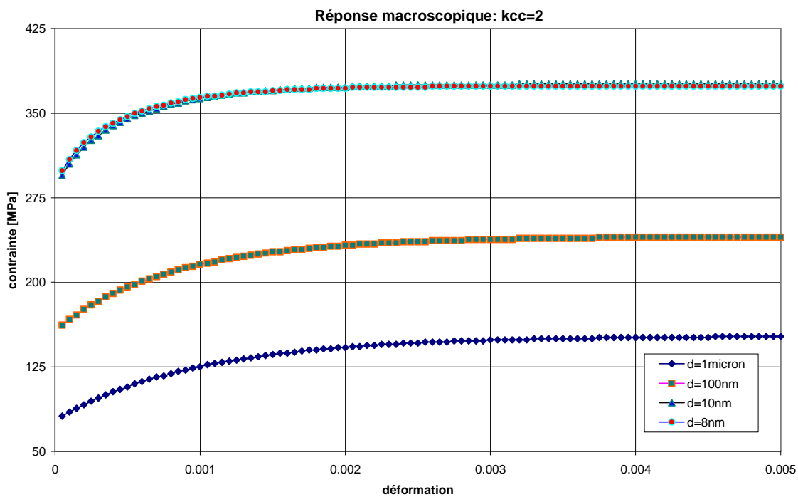
Figure VI-32 : Réponse globale à K_{cc}=2 et 1.E-3/s ( d= 1000 ; 100 ; 10 et 8 \text{ nm} )
