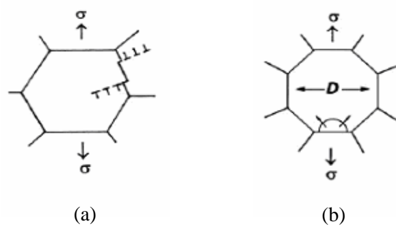
Figure V-3 : Schémas décrivant l'émission de dislocations par les joints de grains (a)-modèle de Li, (b)- modèle de Cheng et al.
