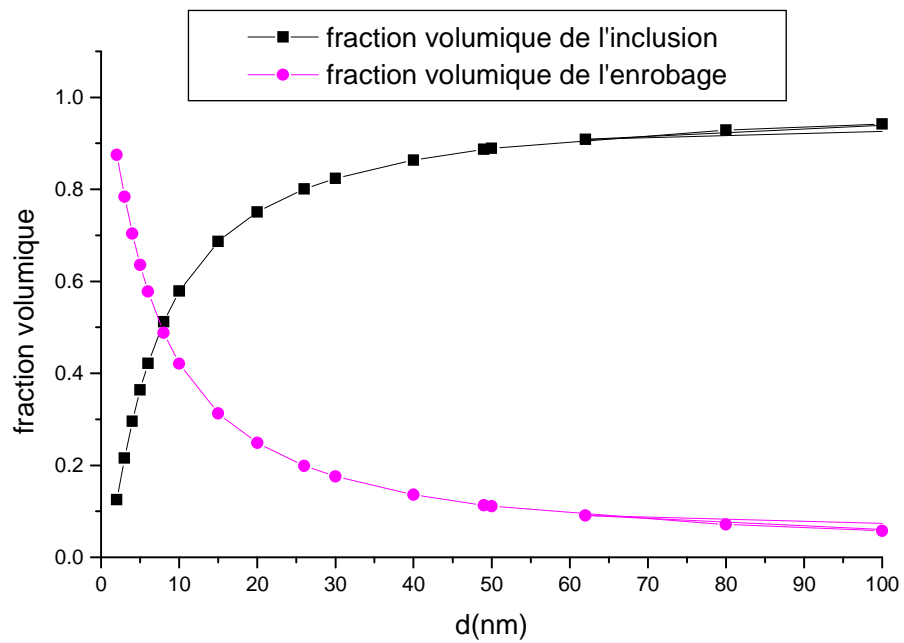
Figure IV-16 : Evolution des fractions volumiques entre 0 et 100 nm
