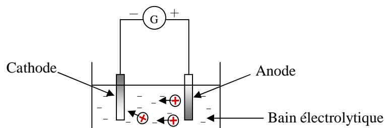
Figure II-16: Principe de l'électrodéposition
