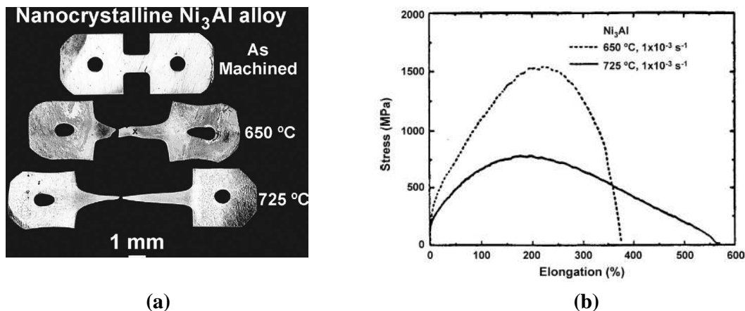
Figure II-45 : (a)- Apparence des échantillons du Ni 3 Al avant et après la déformation (b)- Variation de la contrainte d'écoulement en fonction de l'élongation à 1.E-3/s (Valiev et al., 2000)
