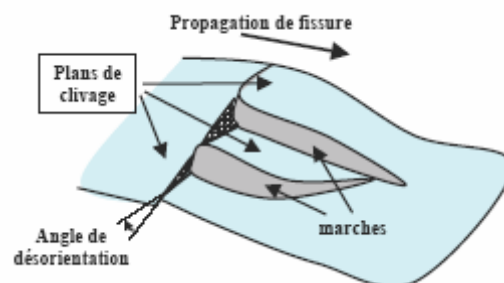
Figure IX-18 : Mécanisme de formation des marches ou lignes de rivières lors du franchissement d'un joint de grain
