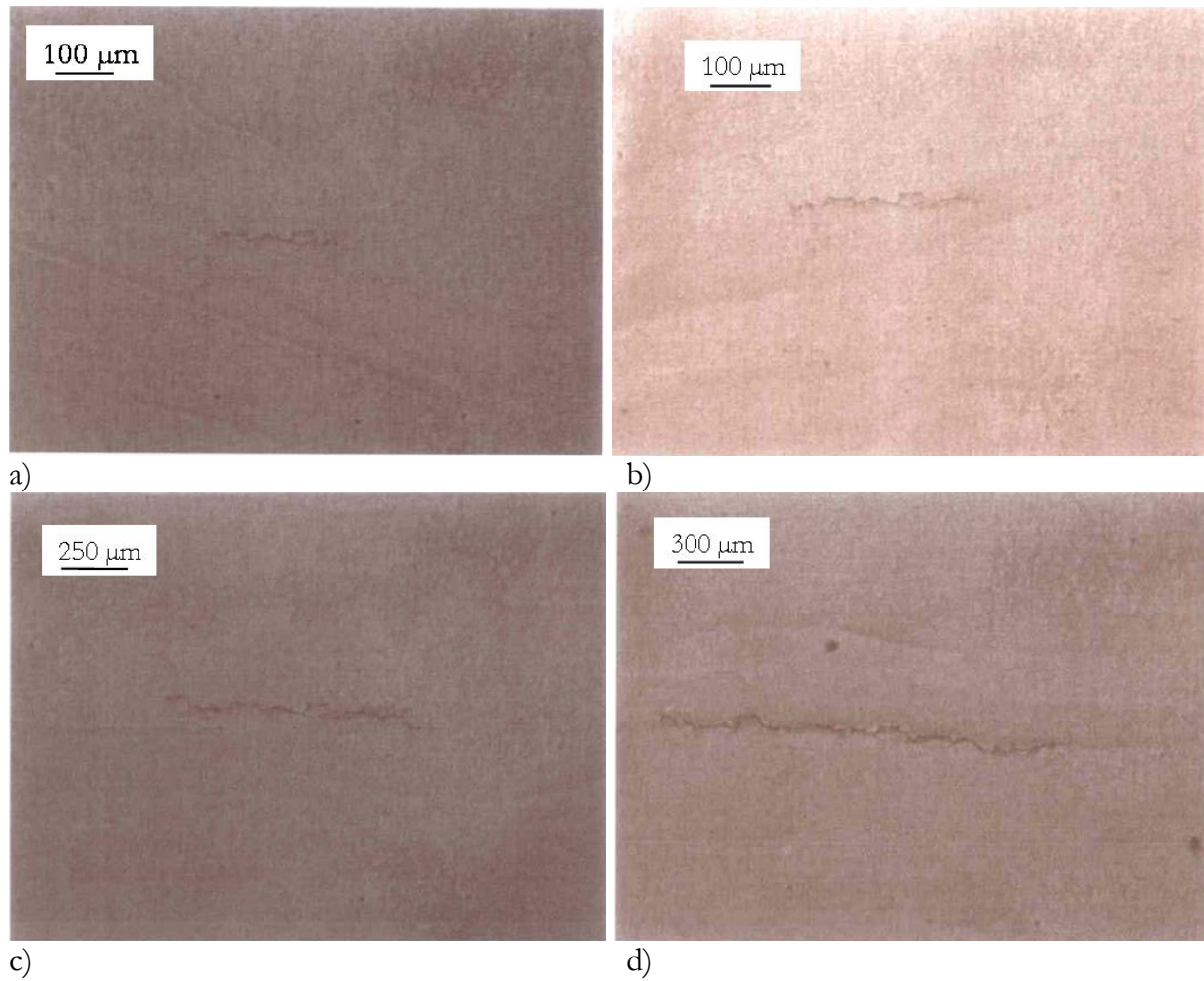
Figure V-1 : Exemple de suivi de fissure à l'aide de réplique plastiques
