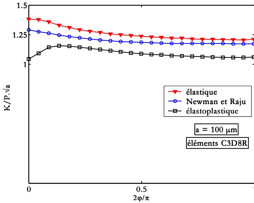
Figure VII-19 : Calcul de K pour des comportements élastique et élastoplastique pour une fissure circulaire ( a/c = 1 et a = 100 \mu\text{m} , \sigma_{app} = 260 \text{ MPa} ).
