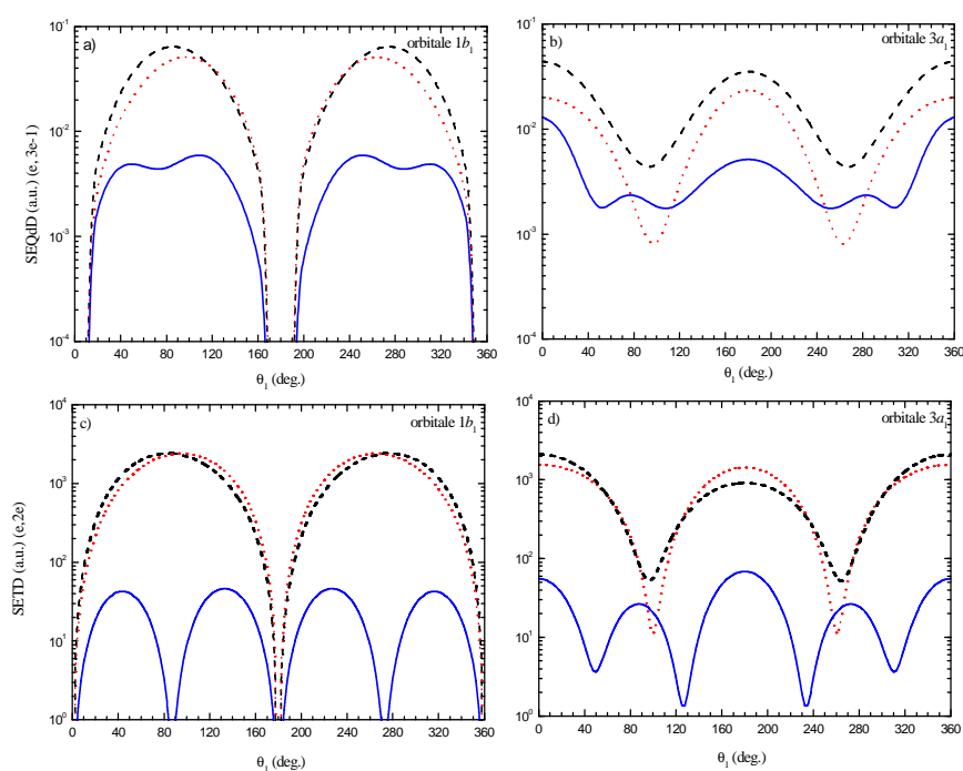
Figure III.10 : SEQdD et SETD pour les orbitales 1b_1 (a, c) et 3a_1 (b, d). Les contributions de l'interaction (électron-électron) et (électron-noyau) sont respectivement représentées par une ligne discontinue et pointillée. Les sections efficaces obtenues avec le potentiel d'interaction total sont représentées par une ligne continue. Les conditions cinématiques sont : E_i = 250 eV, E_1 = E_2 = 5 eV, \theta_d = 0^\circ et \varphi_d = \varphi_1 = 0^\circ pour la double ionisation (a, b) et E_i = 250 eV, E_1 = 5 eV, \theta_d = 0^\circ , et \varphi_d = \varphi_1 = 0^\circ pour la simple ionisation (c, d). Pour les deux cas, l'orientation de la molécule est donnée par (\alpha, \beta, \gamma) = (0^\circ, 0^\circ, 0^\circ) .
