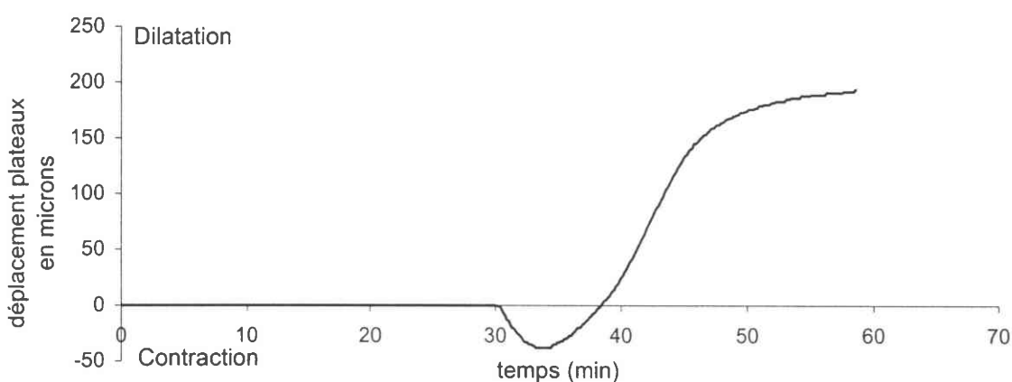
Figure II-4 : Déplacement des plateaux DMTA lors de la cuisson à 3°C/min.
