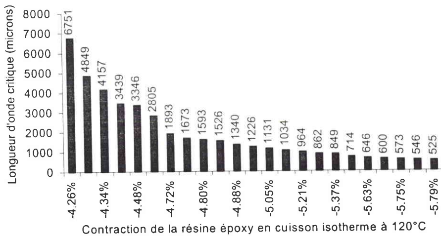
Figure III-25 : Longueur d'onde critique en fonction de la contraction de la résine pour la cuisson en isotherme à 120°C, modèle de BHALERAO (plaque élastique en contrainte plane).
