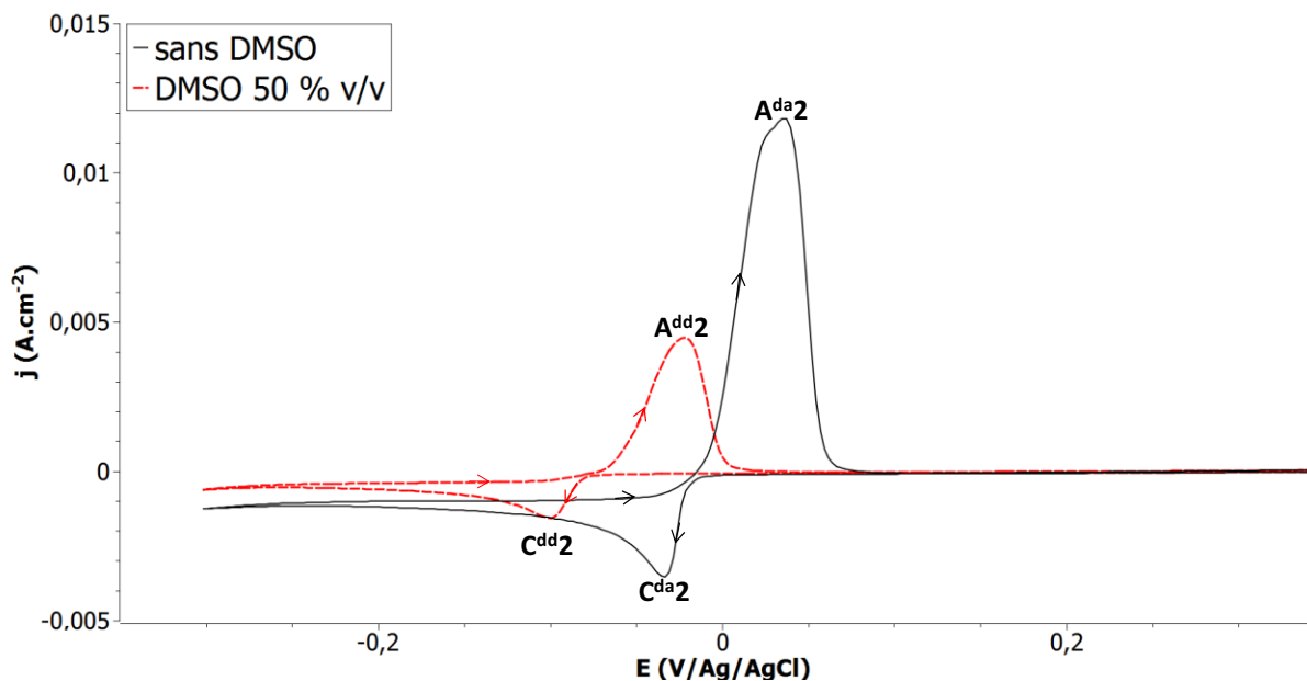
Figure 4.2 : Voltampérométries cycliques à 5 \text{ mV.s}^{-1} sur disque de platine dans des électrolytes d'acide nitrique 1M avec ou sans DMSO (50 % v/v) et contenant [\text{Bi}^{3+}] = 10^{-2} \text{ M} .
