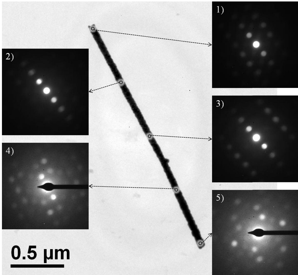
Figure 5.5 : Image en champ clair et clichés de micro-diffraction électronique d'un nanofil électrodéposé à -100\text{ mV/Ag/AgCl} dans une membrane M50 dans un électrolyte d'acide nitrique 1\text{ M} contenant 10\text{ mM} de \text{Bi}^{3+} , 10\text{ mM} de \text{Te}^{\text{IV}} et 50\% v/v de DMSO.
