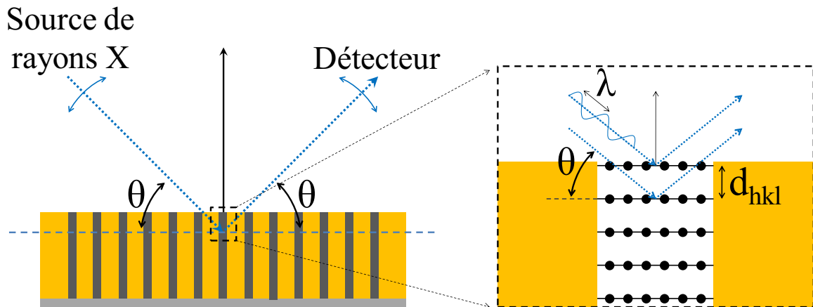
Figure 5.17 : schéma de principe de l'analyse par DRX en mode 2θ.
