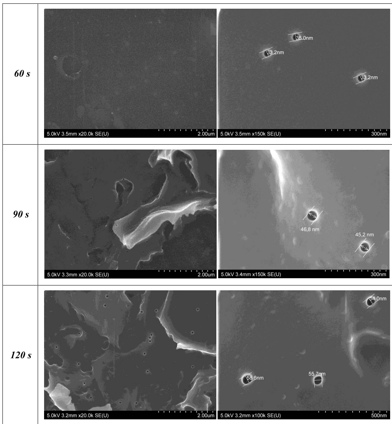
Figure 2.4 : Images MEB de la surface de membranes de PC-BPA de 30 \mu\text{m} d'épaisseurs après des attaques sélectives à la soude 6M à 50°C pendant 30, 60 et 120 s.
