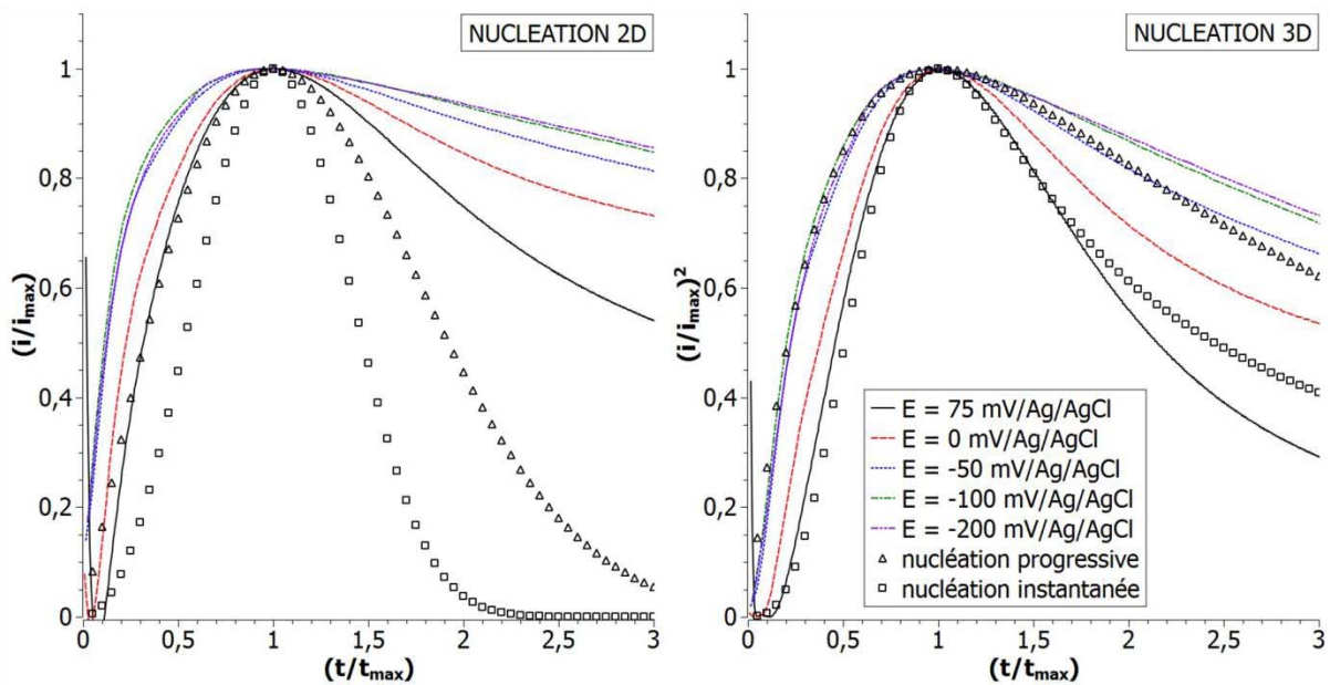
Figure 4.9 : étude des modes de nucléation et croissance sur platine dans un milieu mixte de DMSO 50% v/v, HNO 3 1M et de [Te IV ] = [Bi 3+ ] = 10 -2 M par comparaison des dépôts de Bi 2 Te 3 à différents potentiels avec les modèles théoriques de nucléation 2D (gauche) et 3D (droite).
