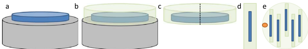
Figure 6.5 : Schémas de préparation des échantillons pour analyses EDX et EPMA. (a) Film de \text{Bi}_x\text{Te}_y déposé sur un substrat d'inox, (b) enrobage du film avec une résine spécifique, (c) découpe du film deux parties, (d) échantillon enrobé pour la découpe par ultra-microtomie et l'analyse par EDX, (e) cinq échantillons analysés par EPMA [215].
